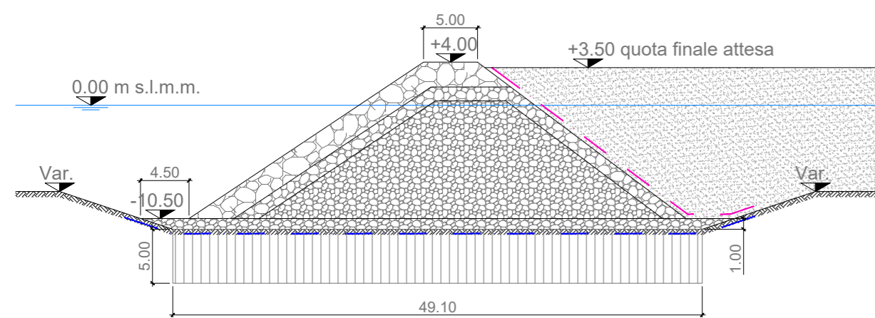
WBS 4a (Sezione F-F) Scala 1:500
