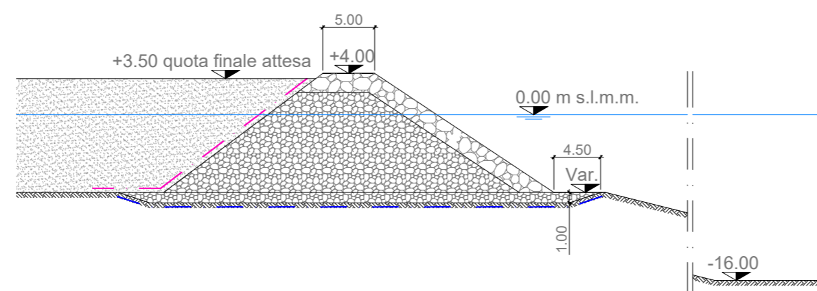
WBS 4b (Sezione Q-Q) Scala 1:500
