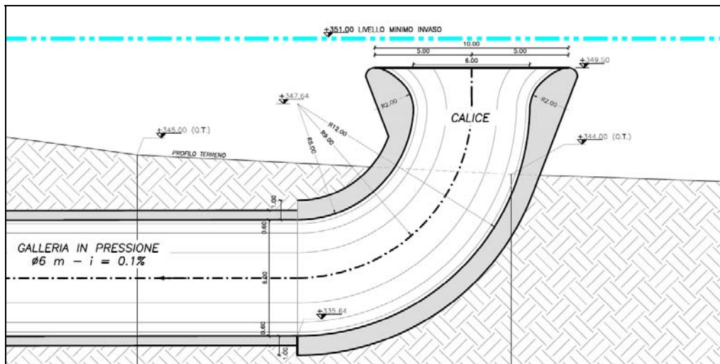
Figura 39 –sezione trasversale opera di presa/restituzione di valle
