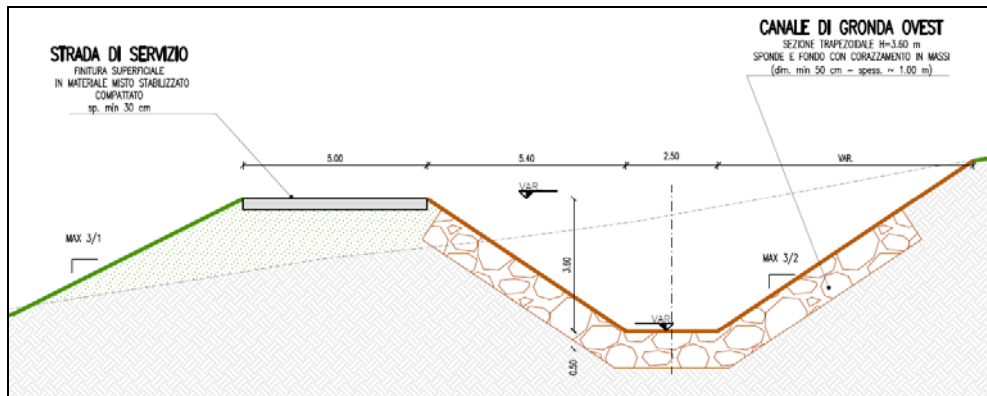
Figura 17 – sezione tipo canale di gronda Ovest
