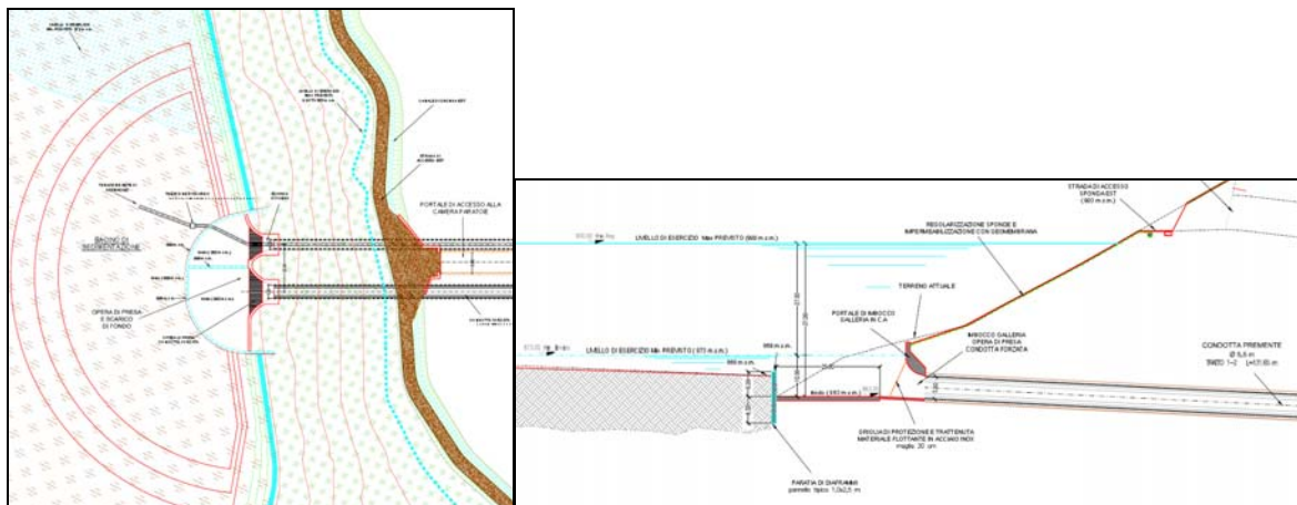
Figura 29 – pianta e sezione manufatto di presa di Monte Alto
