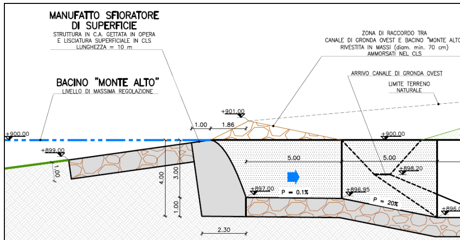
Figura 23 –sezione manufatto sfioratore di superficie
