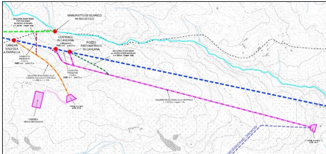
Figura 44 –stralcio planimetrico tracciato galleria di accesso alla centrale
