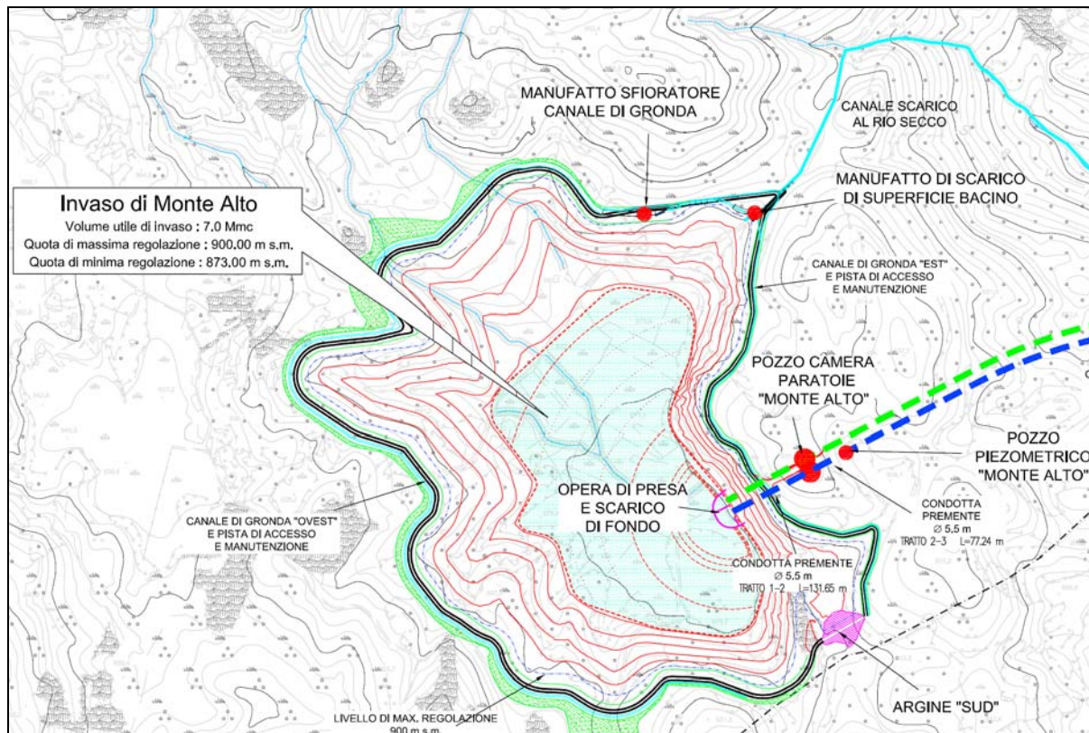
Figura 14 – stralcio planimetrico delle opere in progetto del bacino di Monte Alto
