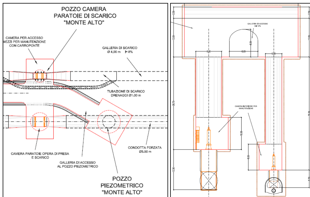
Figura 30 – pianta e sezione camera paratoie di Monte Alto
