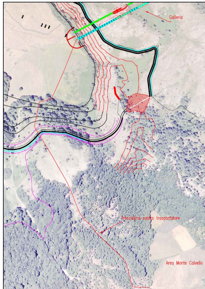
Figura 15 – tracciato del nastro trasportatore di collegamento tra M. Alto e M. Calvello
