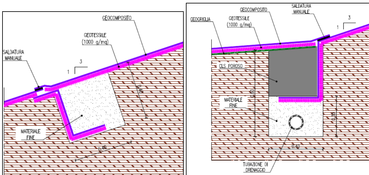
Figura 16 – collegamento teli in PVC per impermeabilizzazione bacino di Monte Alto
