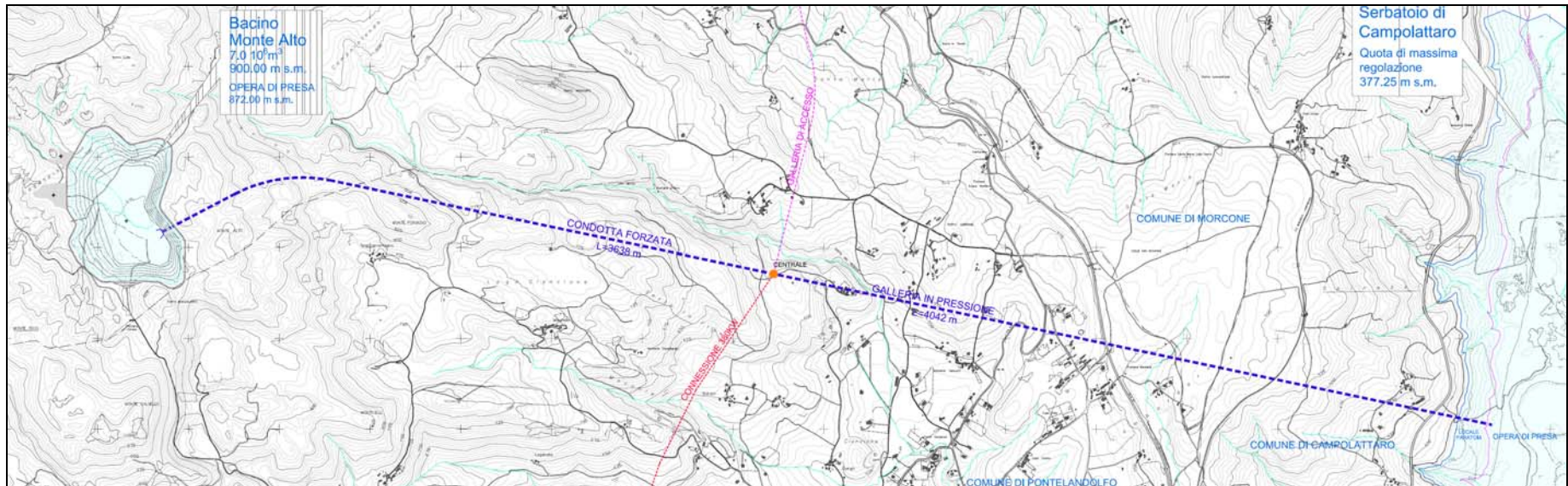
Figura 2 – planimetria progetto di massima dell’impianto – soluzione in variante Aprile 2010
