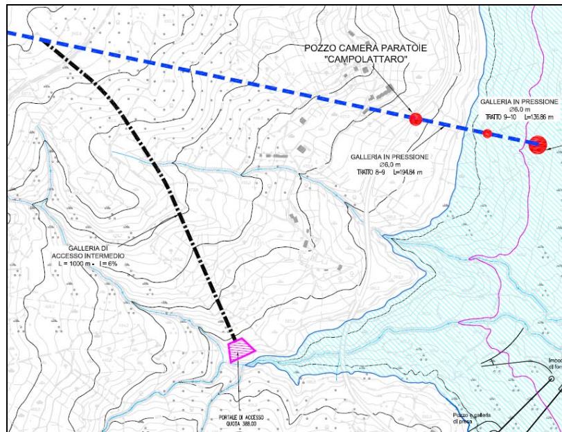
Figura 46 –stralcio planimetrico tracciato galleria di accesso intermedio
