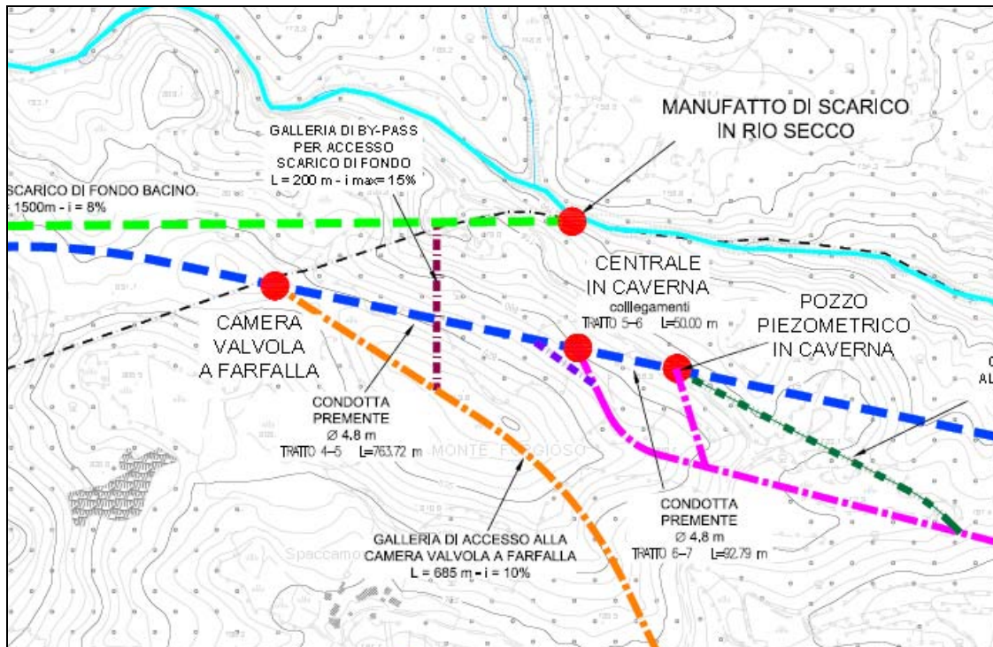
Figura 43 –stralcio planimetrico tracciato galleria di collegamento
