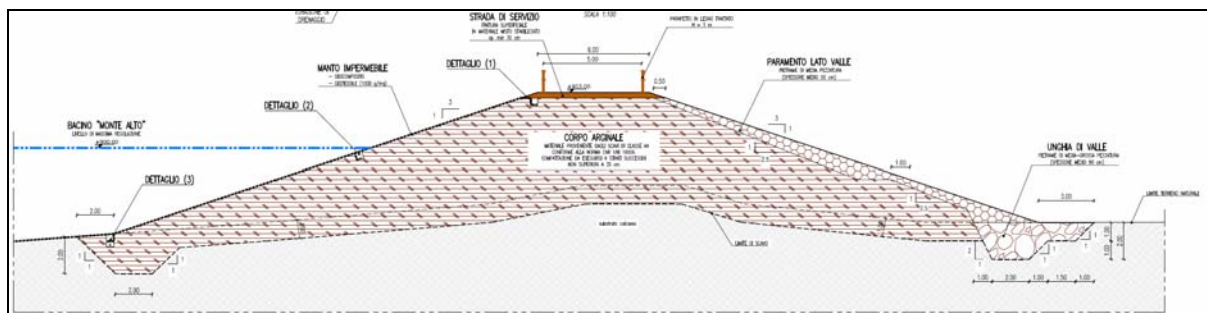
Figura 21 – sezione tipo argine sud
