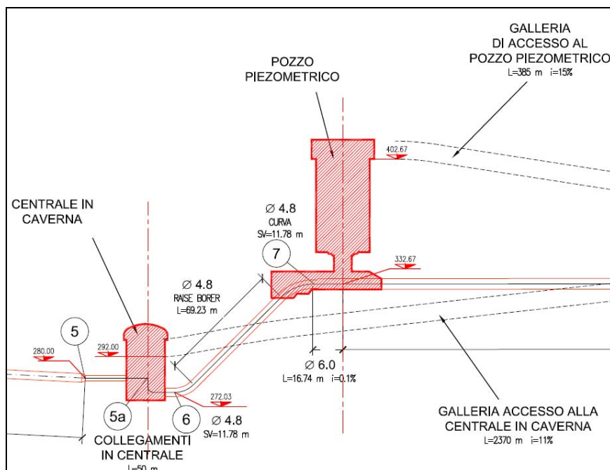
Figura 11 – nodo idraulico pozzo piezometrico di valle
