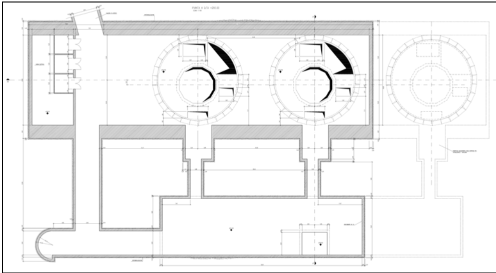
Figura 34 – pianta centrale in caverna alla quota 292 m s.m.
