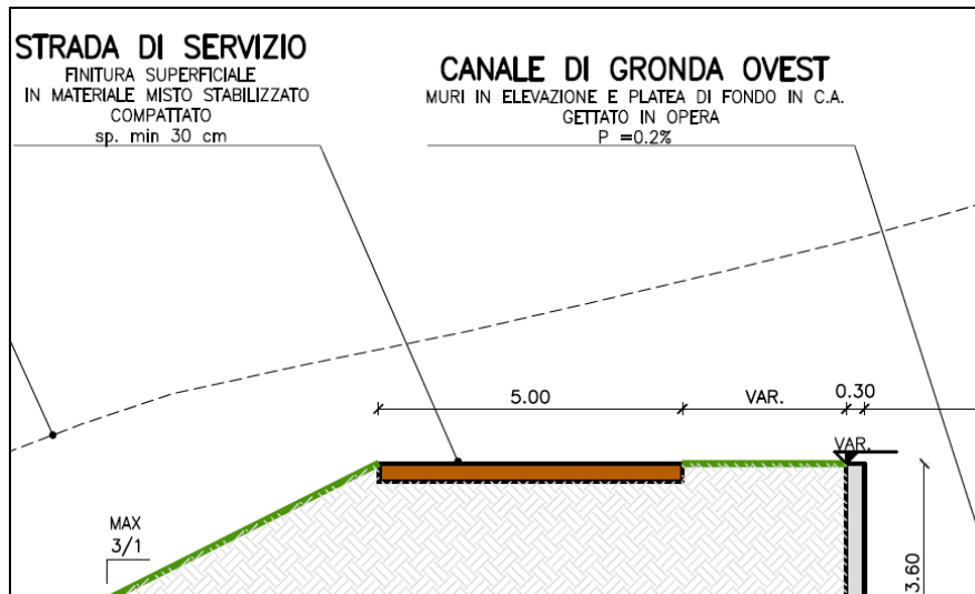
Figura 20 – sezione tipo strada perimetrale al bacino di Monte Alto
