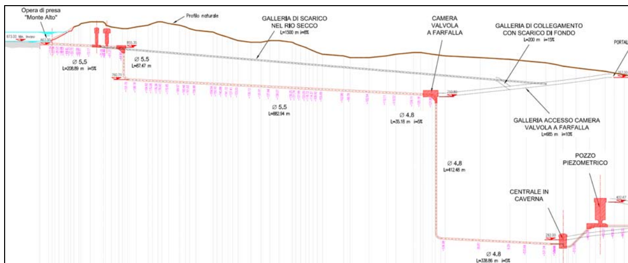
Figura 32 – profilo condotta forzata
