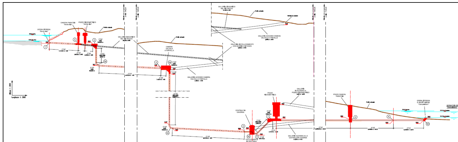
Figura 4 – profilo schematico di impianto
