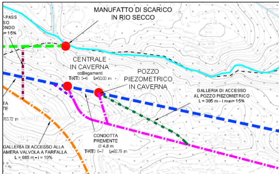
Figura 45 –stralcio planimetrico tracciato galleria di accesso sup. al pozzo piezometrico di valle
