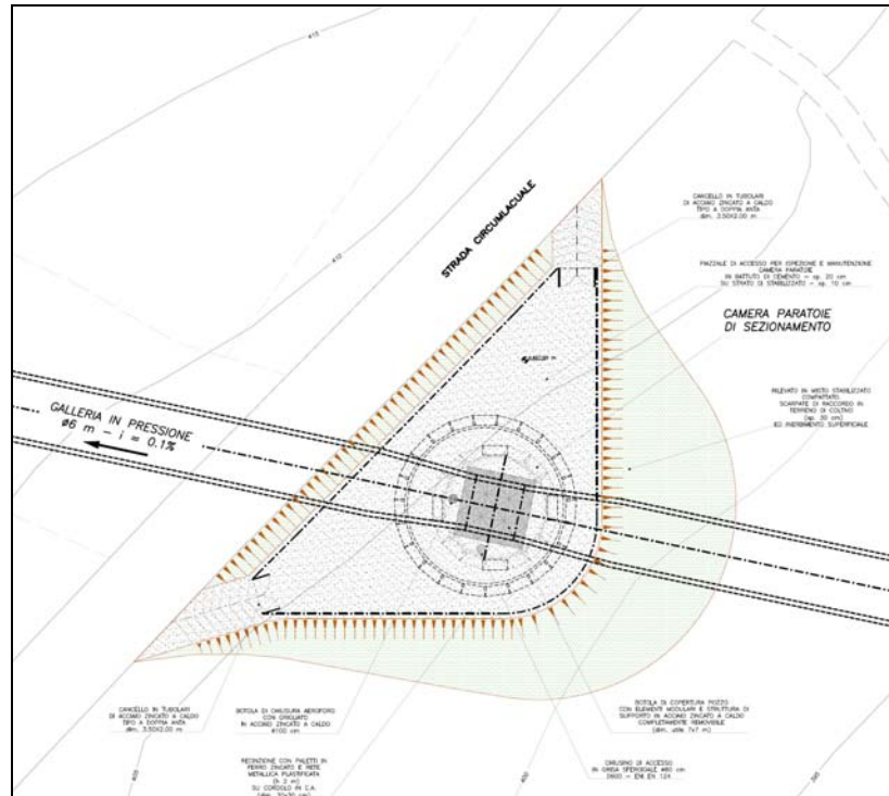
Figura 38 –stralcio planimetrico piazzale di accesso al pozzo paratoie di valle
