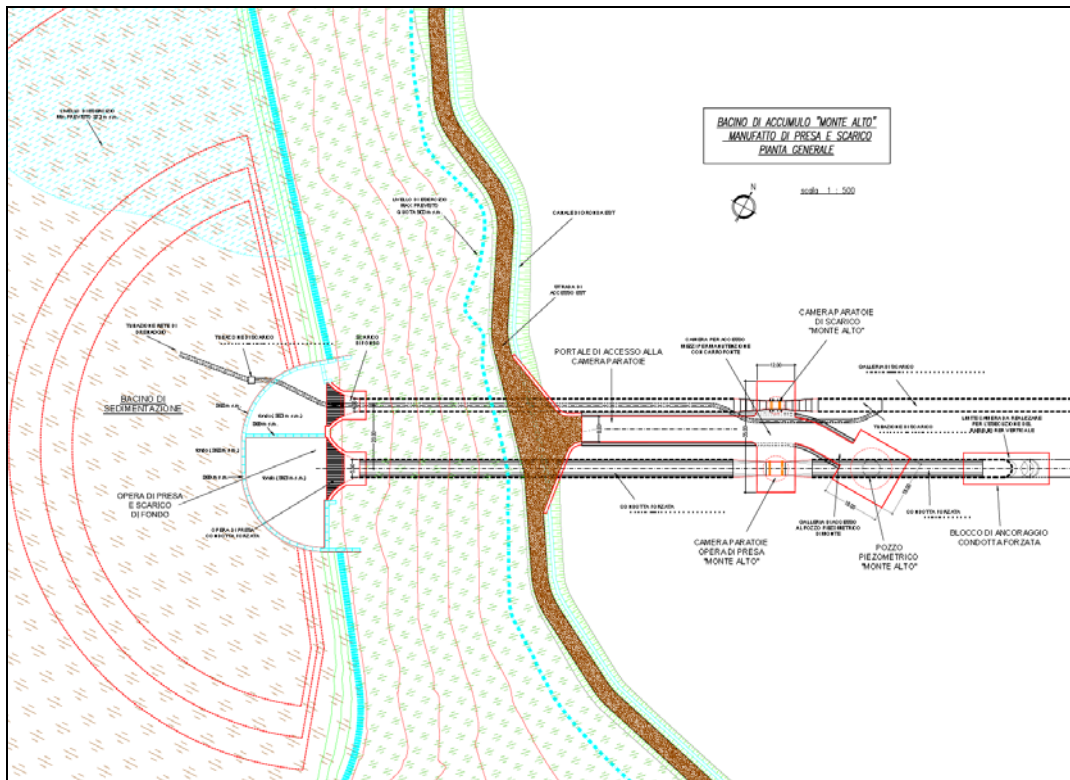
Figura 6 – stralcio planimetrico bacino ed opera di presa di Monte Alto
