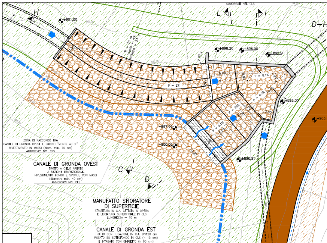
Figura 24 – pianta manufatto di confluenza
