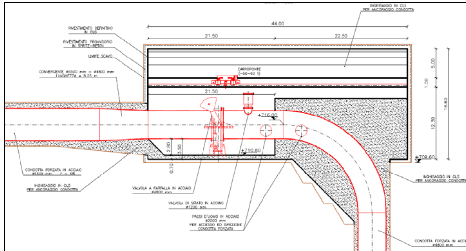
Figura 33 – camera valvola a farfalla
