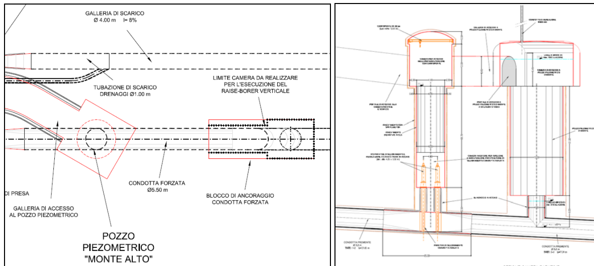
Figura 31 – pianta e sezione pozzo piezometrico di monte
