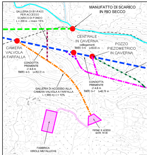
Figura 27 – stralcio planimetrico tracciato galleria di collegamento
