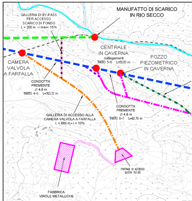
Figura 42 –stralcio planimetrico tracciato galleria di accesso alla camera valvola a farfalla
