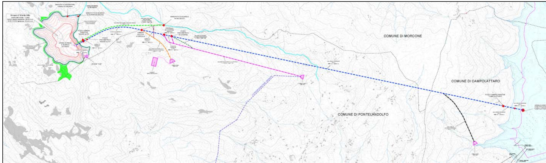
Figura 3 – planimetria opere previste nel presente progetto
