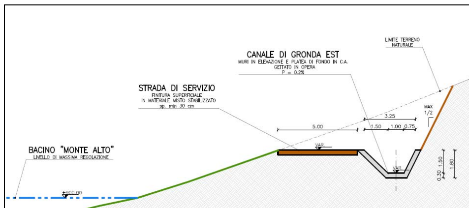
Figura 19 – sezione tipo canale di gronda Est
