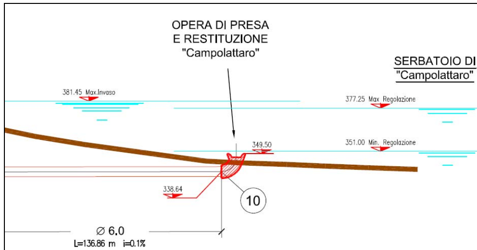
Figura 10 – nodo idraulico opera di presa/restituzione di valle
