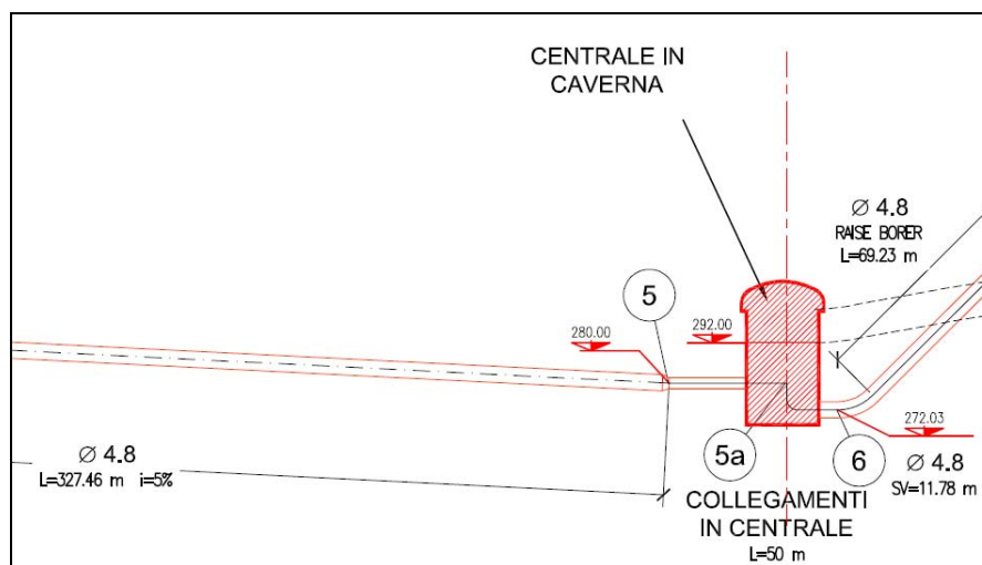
Figura 9 – centrale in caverna
