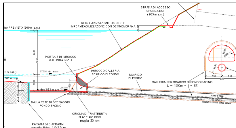
Figura 25 – sezione longitudinale manufatto di presa dello scarico di fondo
