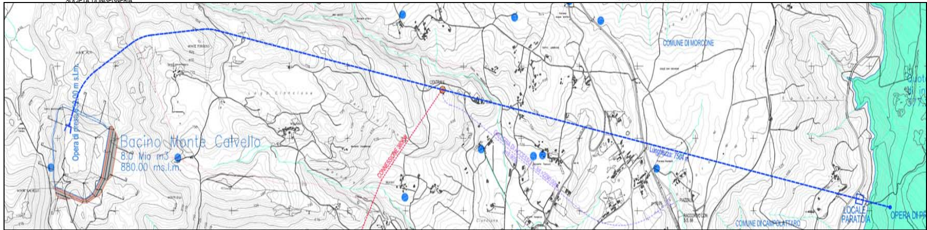
Figura 1 – planimetria progetto di massima dell’impianto– soluzione Aprile 2008
