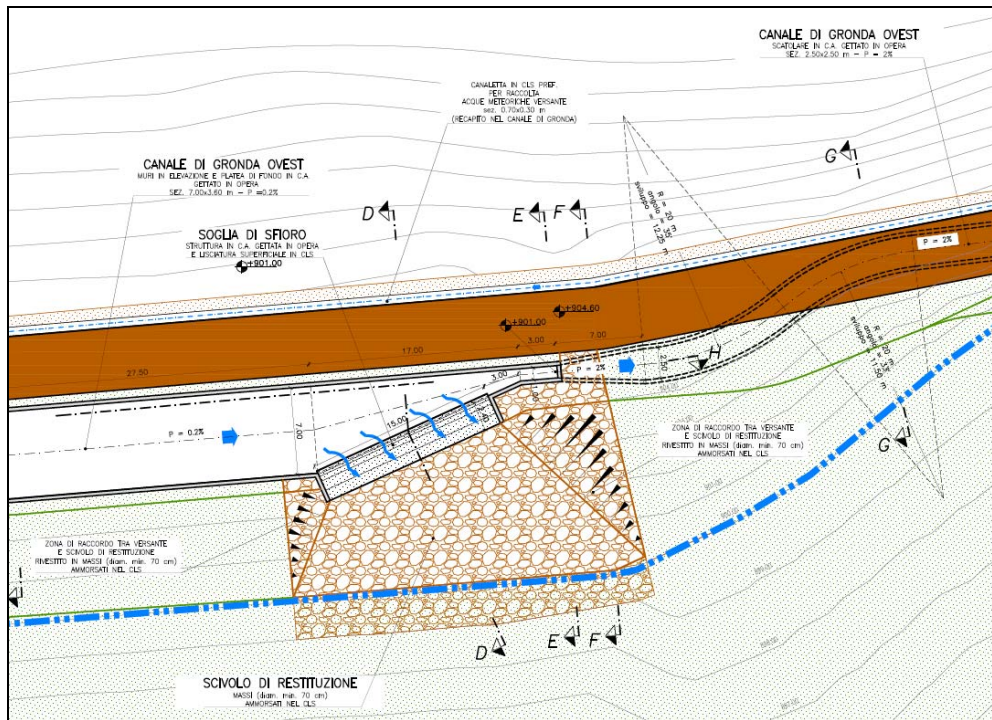
Figura 18 – manufatto di sfioro del canale di gronda Ovest
