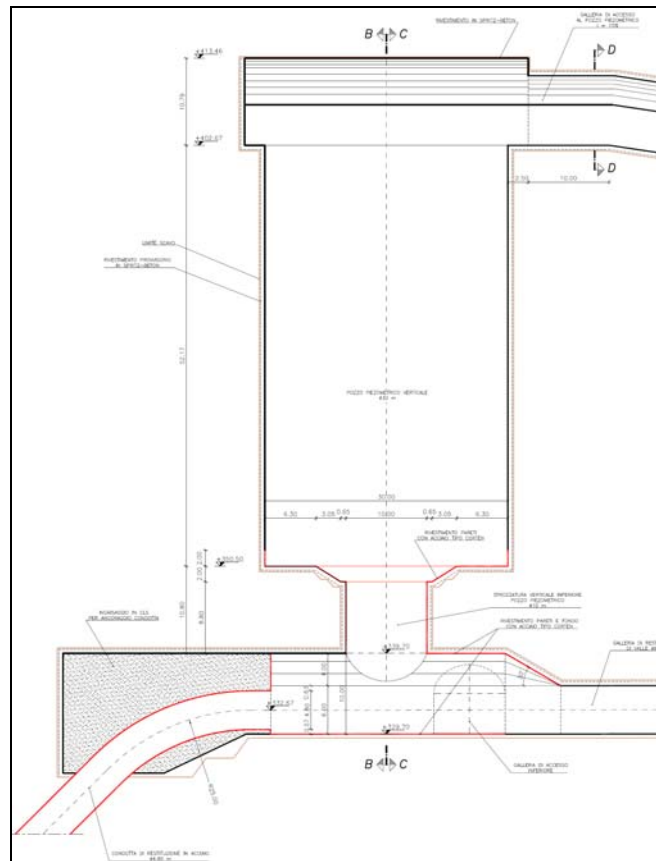
Figura 36 – sezione trasversale pozzo piezometrico di valle
