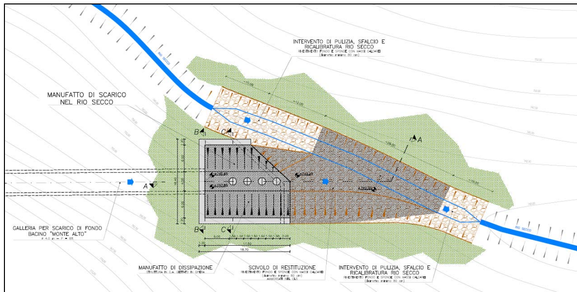
Figura 28 – manufatto di dissipazione dello sbocco dello scarico di fondo nel Rio Secco
