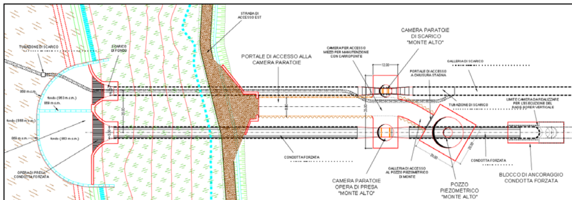
Figura 41 –stralcio planimetrico galleria di accesso alla camera paratoie di monte
