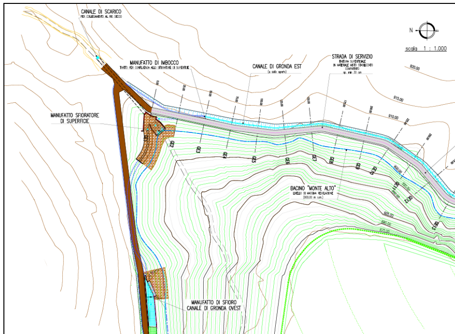
Figura 22 – localizzazione opere di scarico
