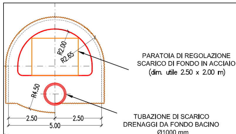
Figura 26 – sezione tipo galleria di scarico con tubazione di convogliamento drenaggi
