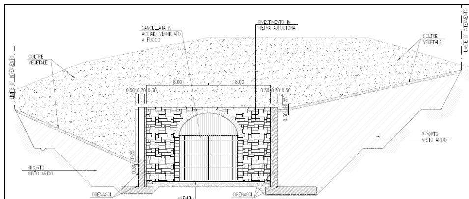
Figura 47 –sistemazione portali di accesso gallerie
