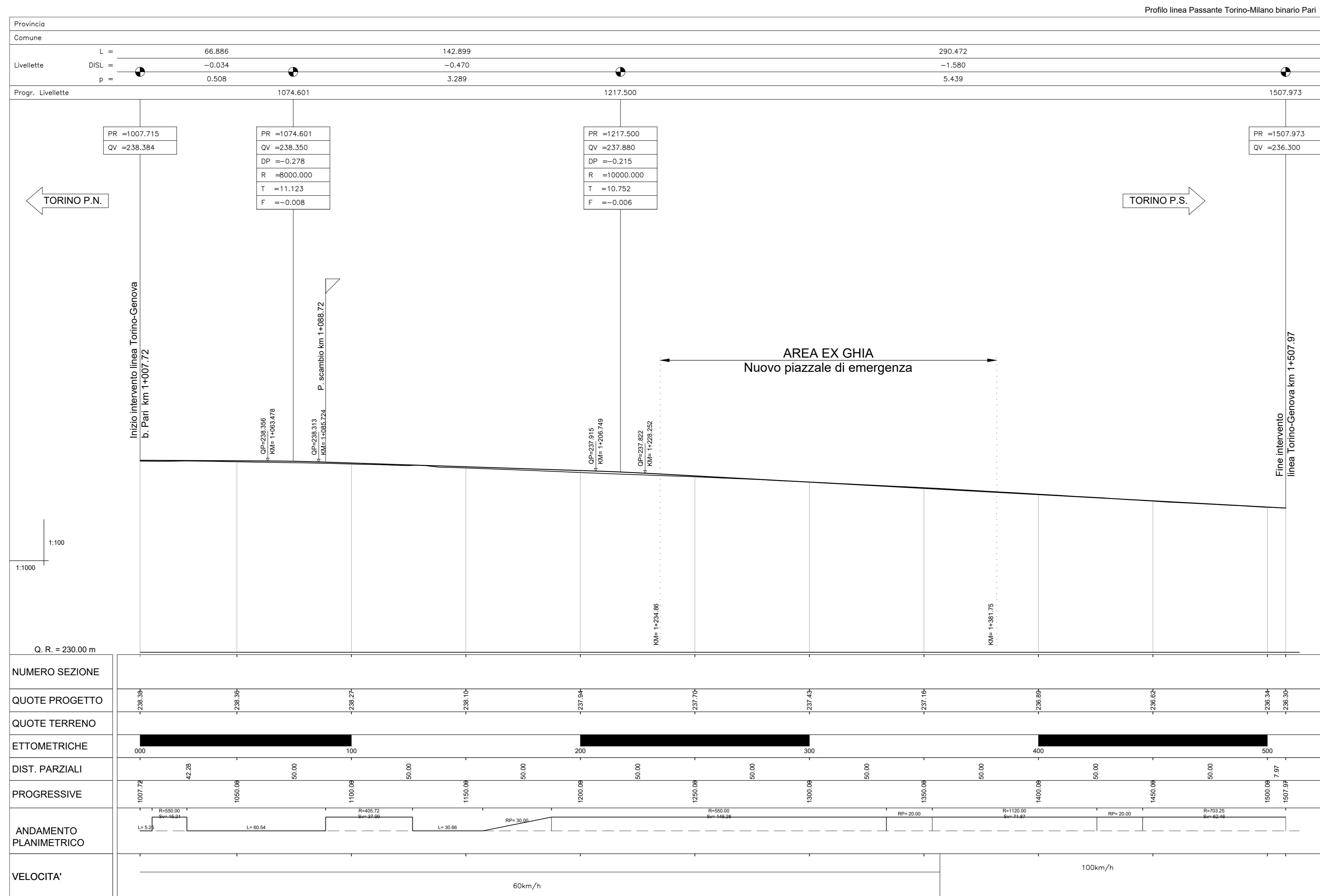
Profilo linea Passante Torino-Milano binario Pari
