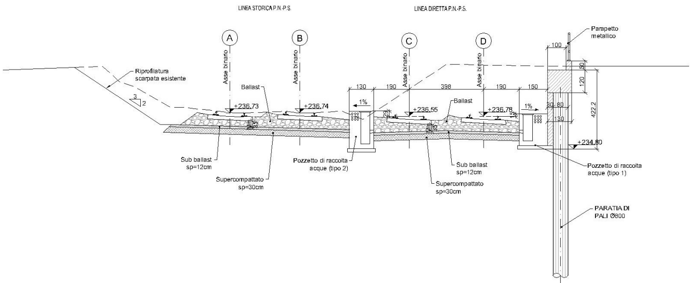
FIGURA 4 SEZIONE TRASVERSALE DELLA PARATIA
