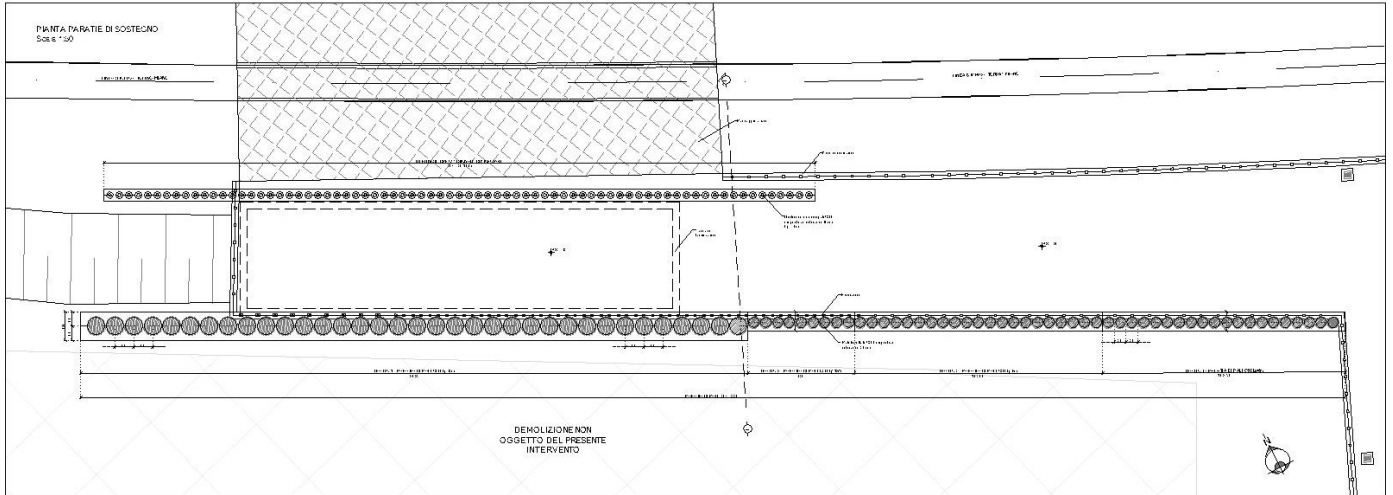
FIGURA 2 STRALCIO PLANIMETRICO PARATIA DI SOSTEGNO PROVVISORIALE B
