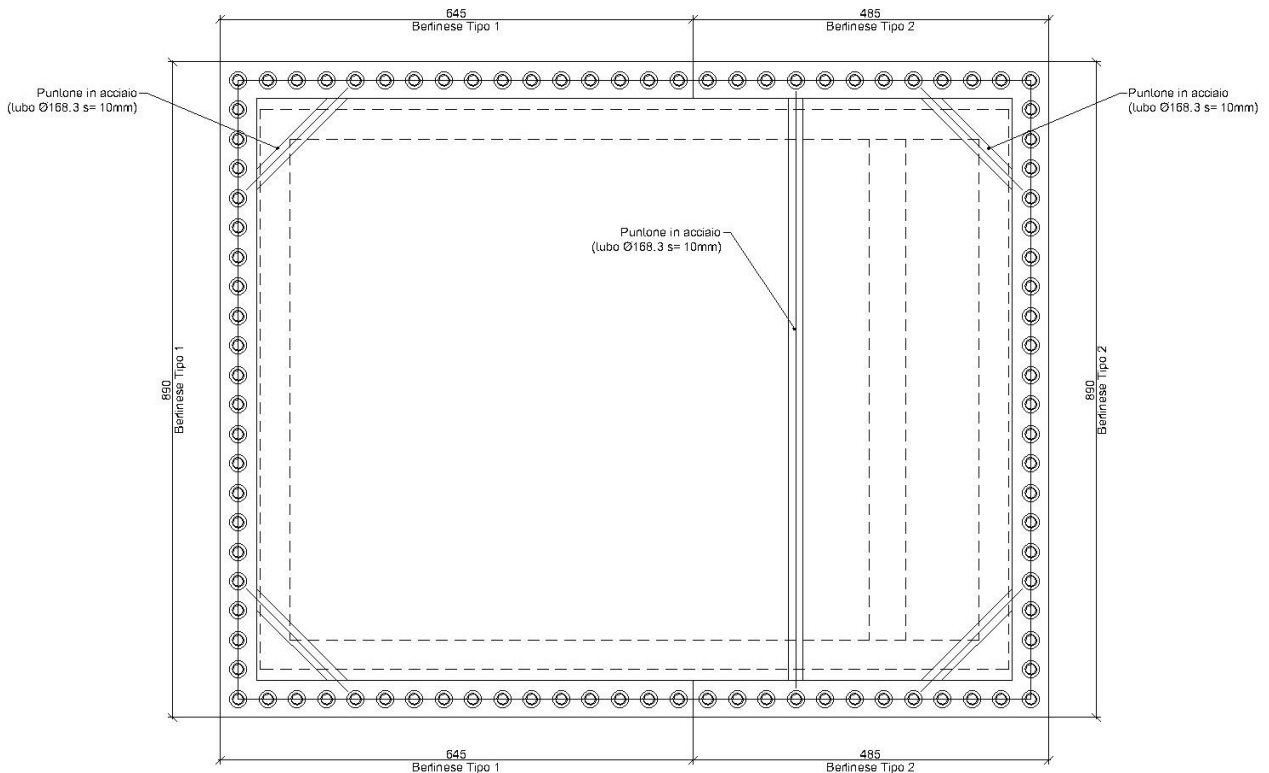
FIGURA 4 PIANTA
