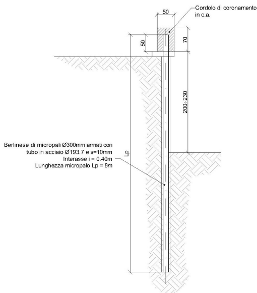
FIGURA 8 SEZIONE TIPO
