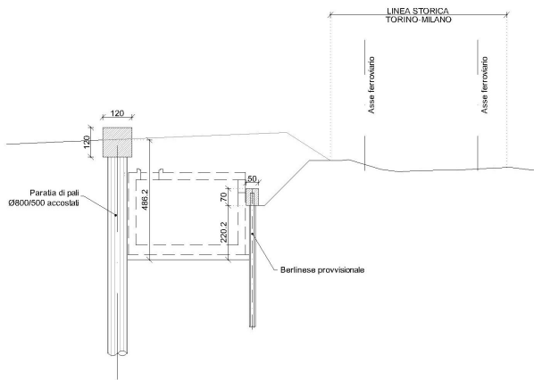
FIGURA 8 SEZIONE TIPO
