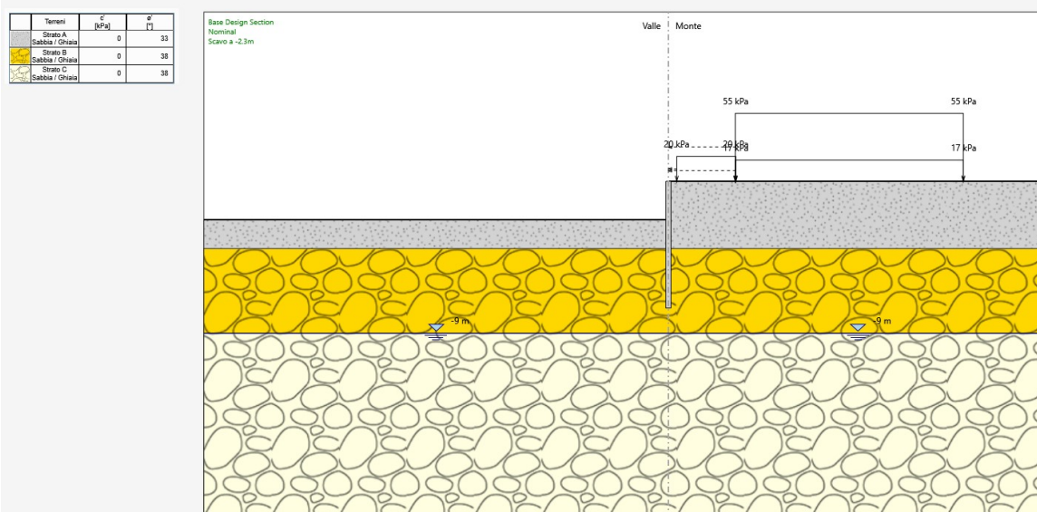
FIGURA 9 FASE FINALE DI SCAVO
