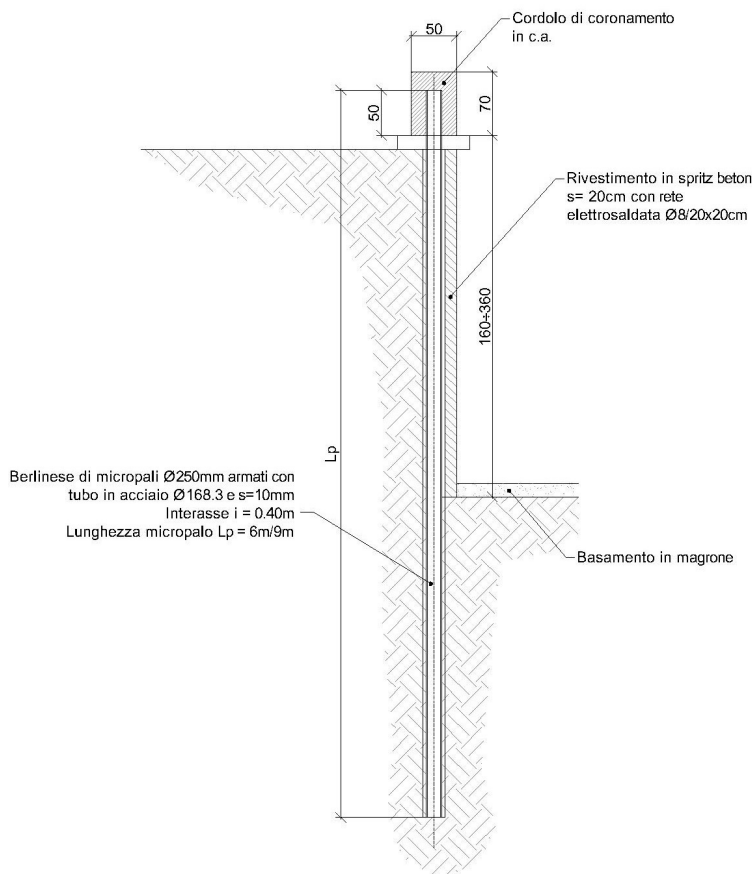
FIGURA 5 SEZIONE LONGITUDINALE
