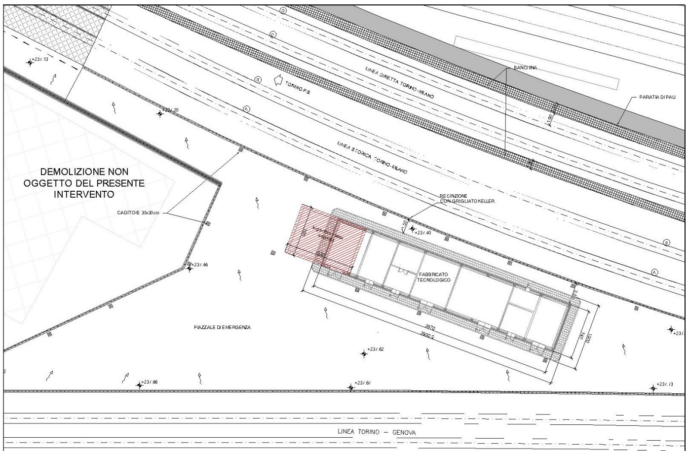
FIGURA 1 STRALCIO PLANIMETRICO PARATIA DI SOSTEGNO PROVVISORIALE A
