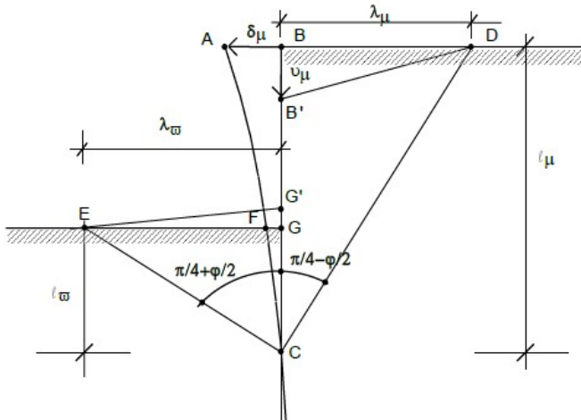
FIGURA 3 VALUTAZIONE DEI CEDIMENTI IN TERRENI INCOERENTI
