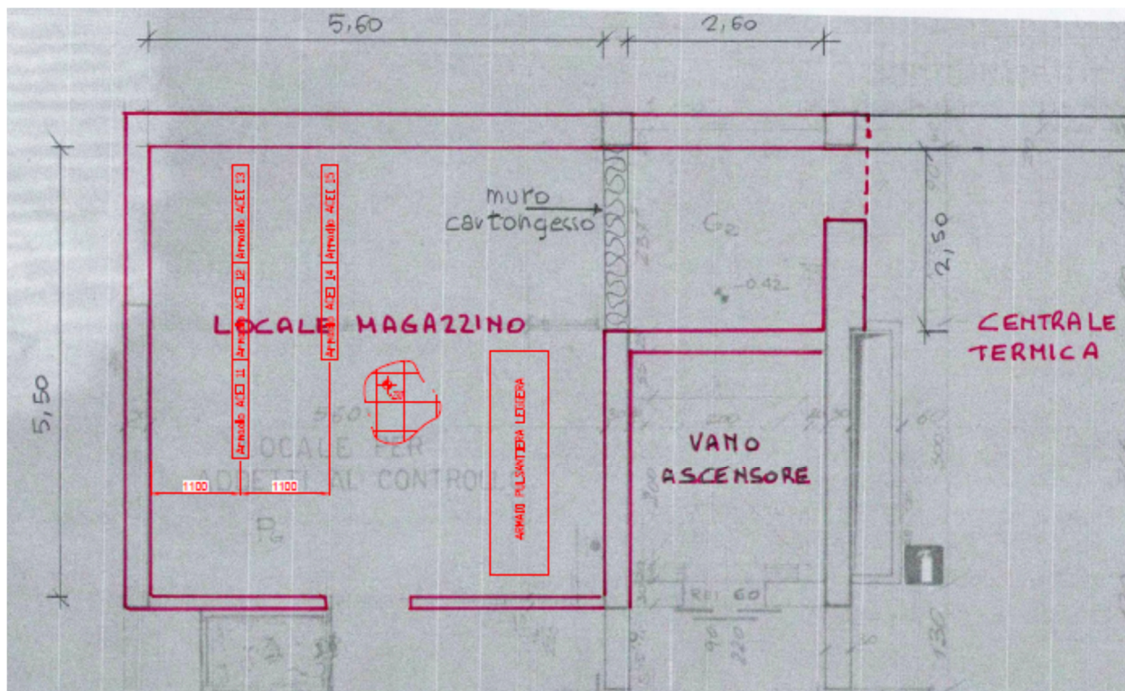
Figura 5: Nuovo Locale tecnico ACEI TO Porta Nuova - posizione nuovi armadi ACEI e Pulsantiere Leggere
