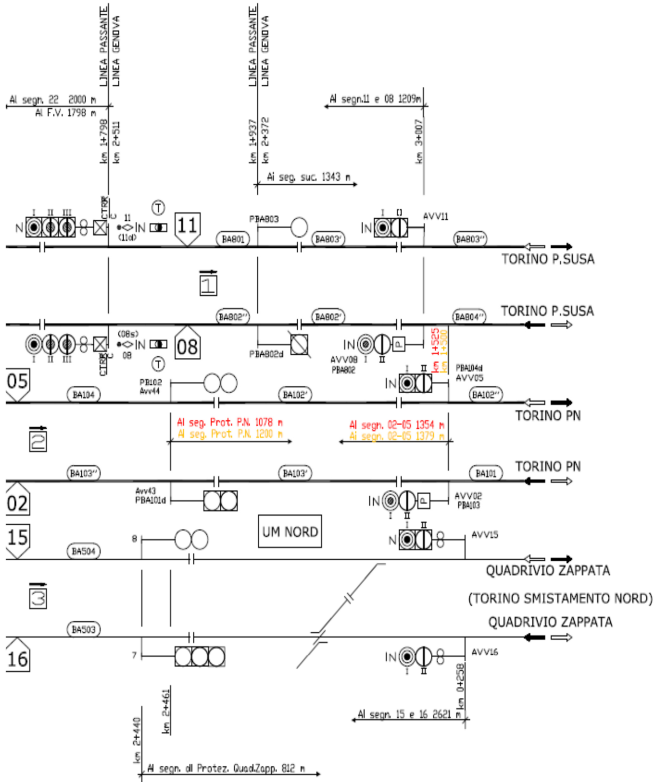
• Figura 4: ACC TO Lingotto – modifica PBA tratta TO Lingotto-TO Porta Nuova
