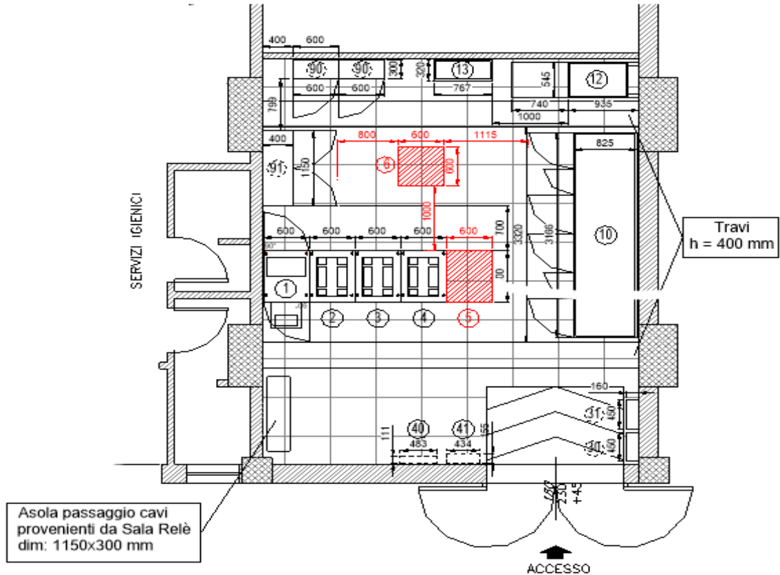
• Figura 2: Layout Locali GEA TO Porta Nuova (GEA-L e PP1)
