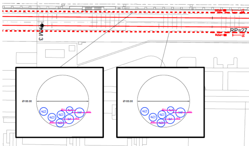
Figura 6: Rappresentazioni tubi nel tunnel (occupazioni cavi IS)
