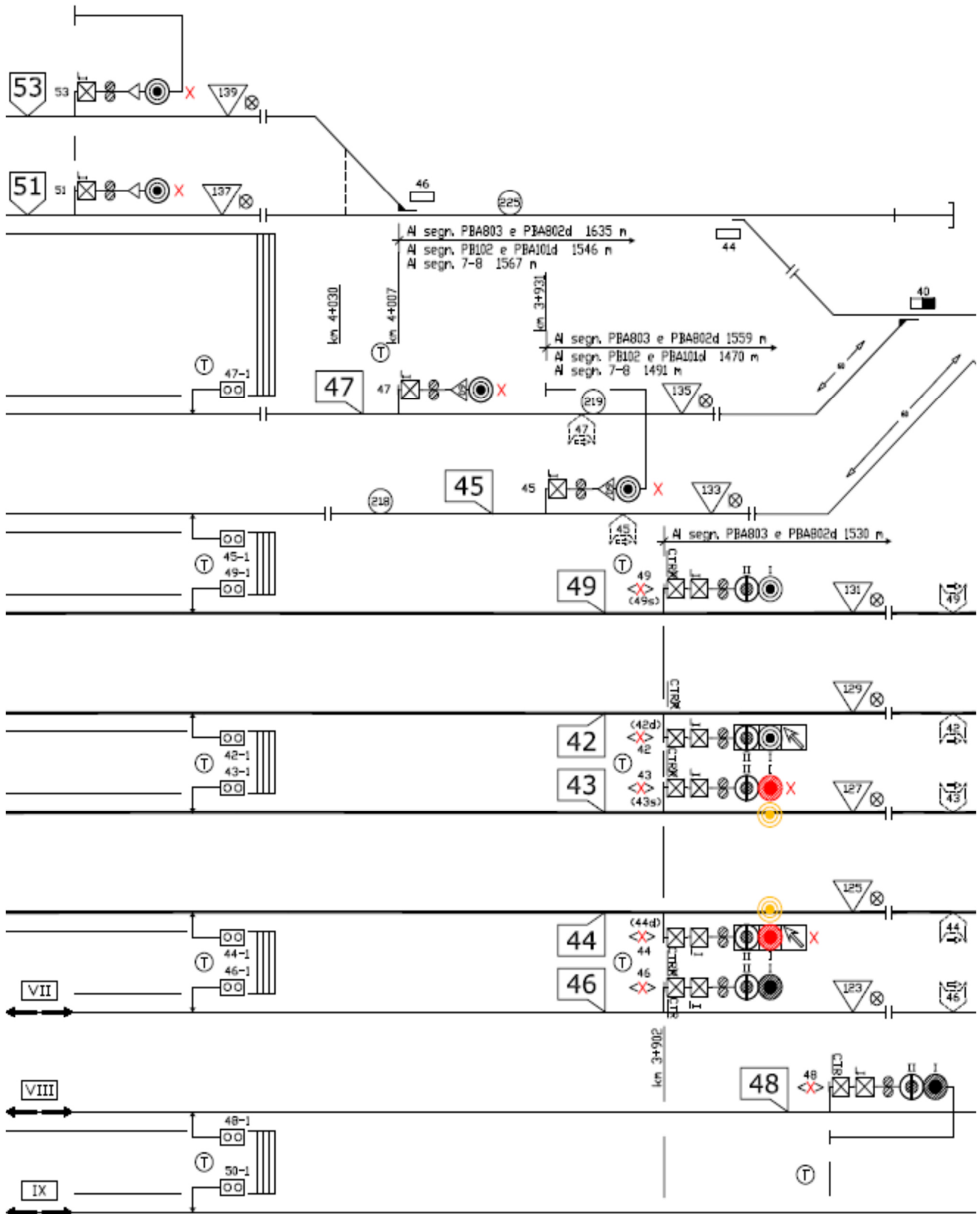
• Figura 3: ACC TO Lingotto – modifica aspetti segnali di partenza
