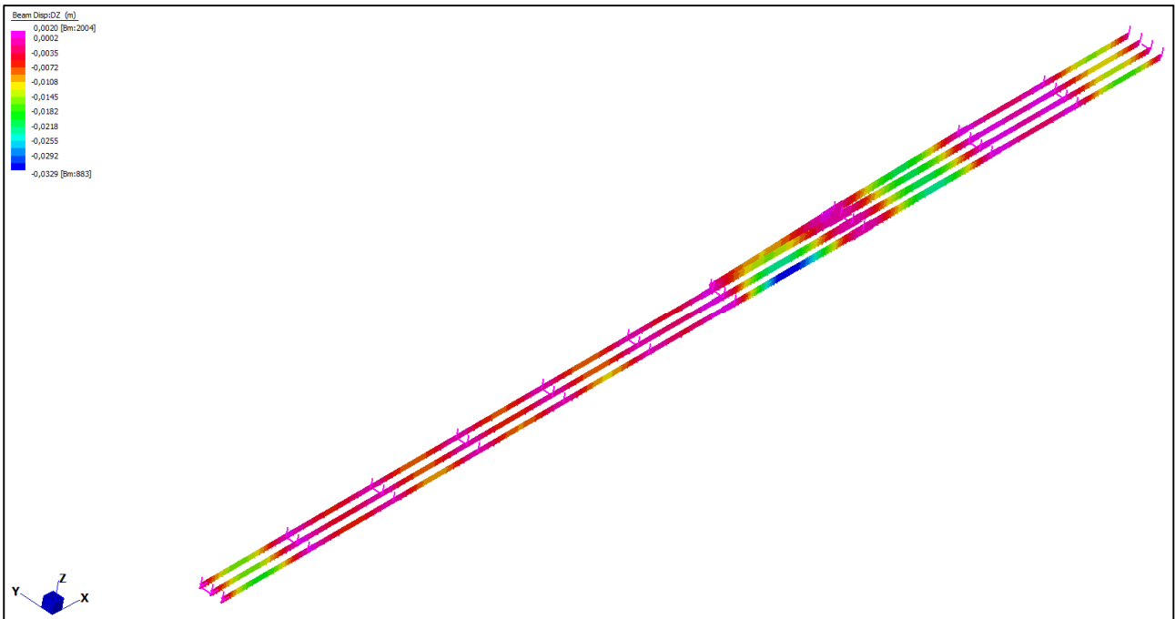
Figura 24: Fase 2 - deformata SLE rara
