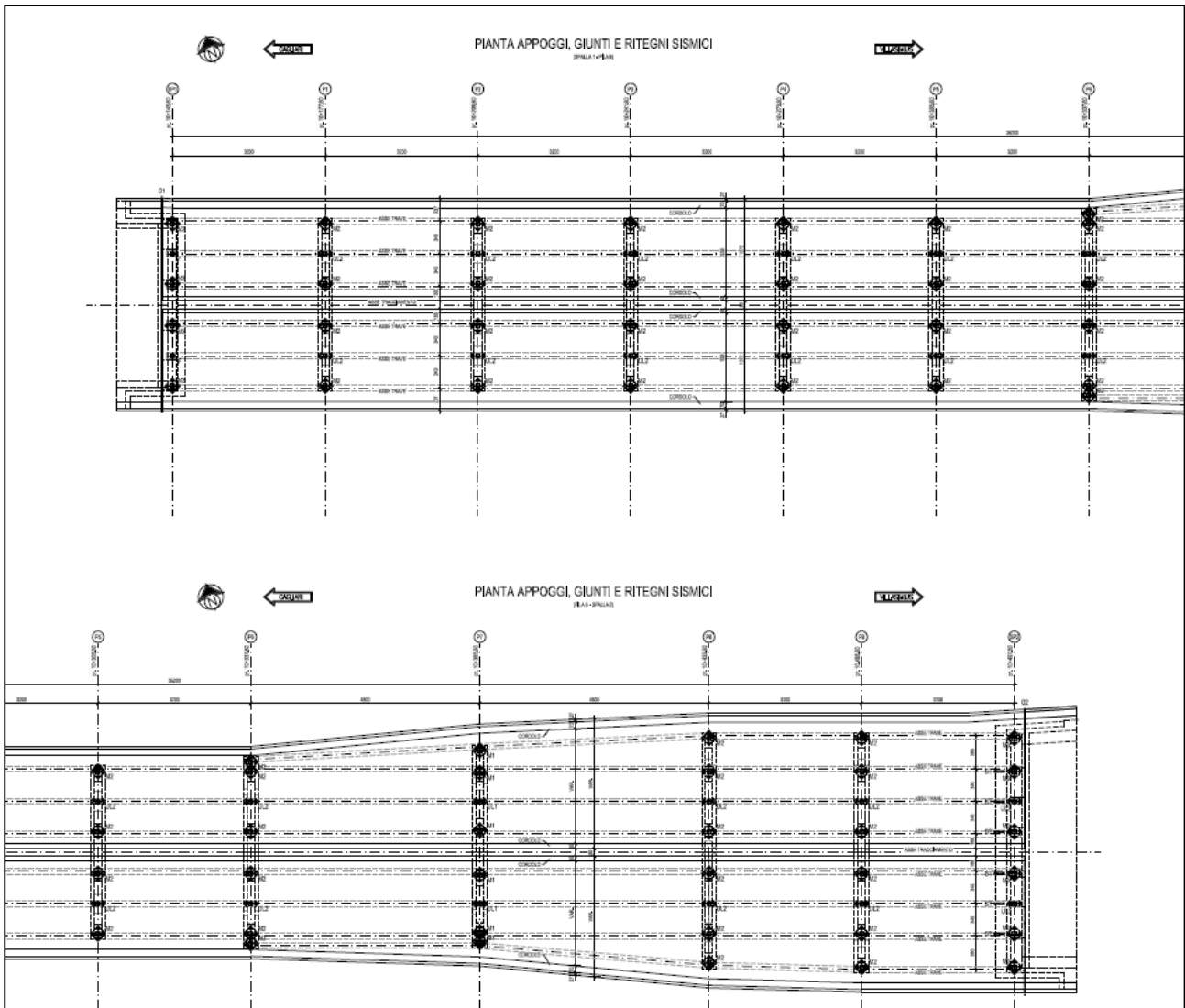
Figura 33 – Pianta appoggi e giunti.
