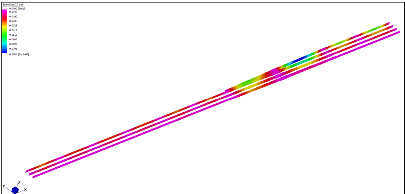
Figura 25: Fase 3 - deformata SLE rara
