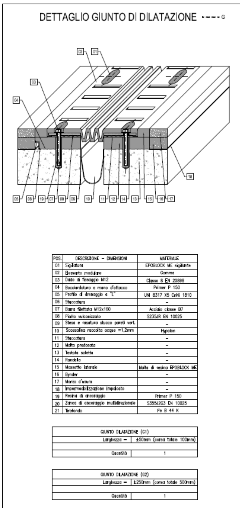
Figura 37 – Giunti di dilatazione(G): specifiche tecniche e spostamenti.
