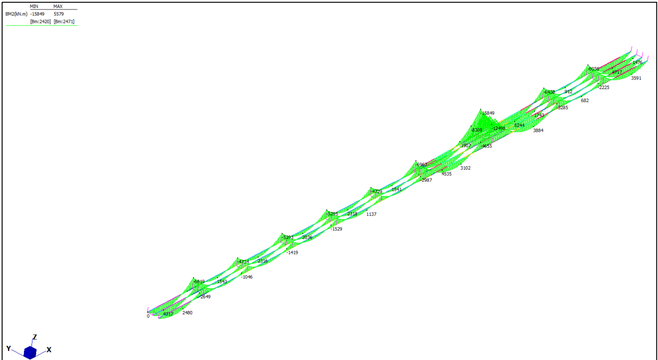
Figura 9: Fase 1: momento flettente impalcato
