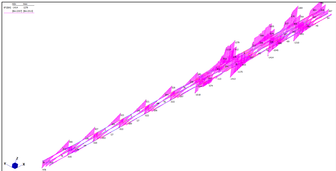
Figura 14: Fase 3: taglio impalcato (involuppo)
