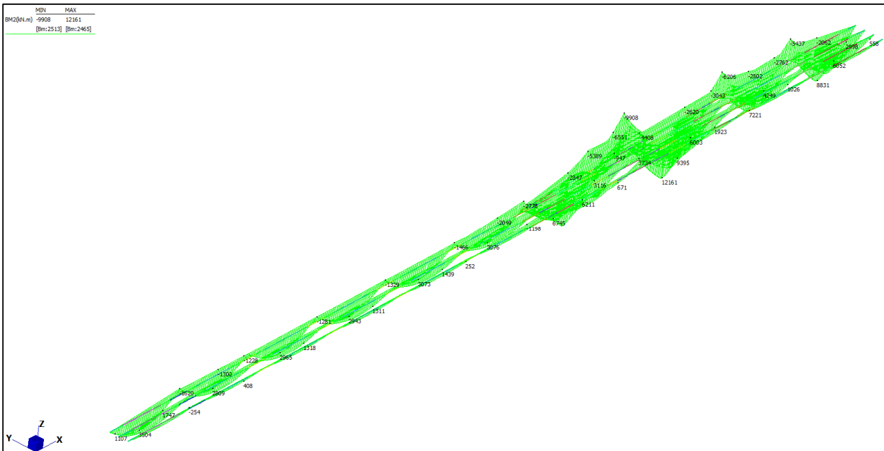
Figura 11: Fase 3: momento flettente impalcato (inviluppo)
