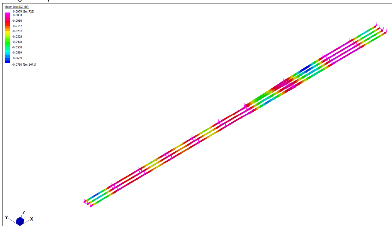
Figura 23: Fase 1 - deformata SLE rara
