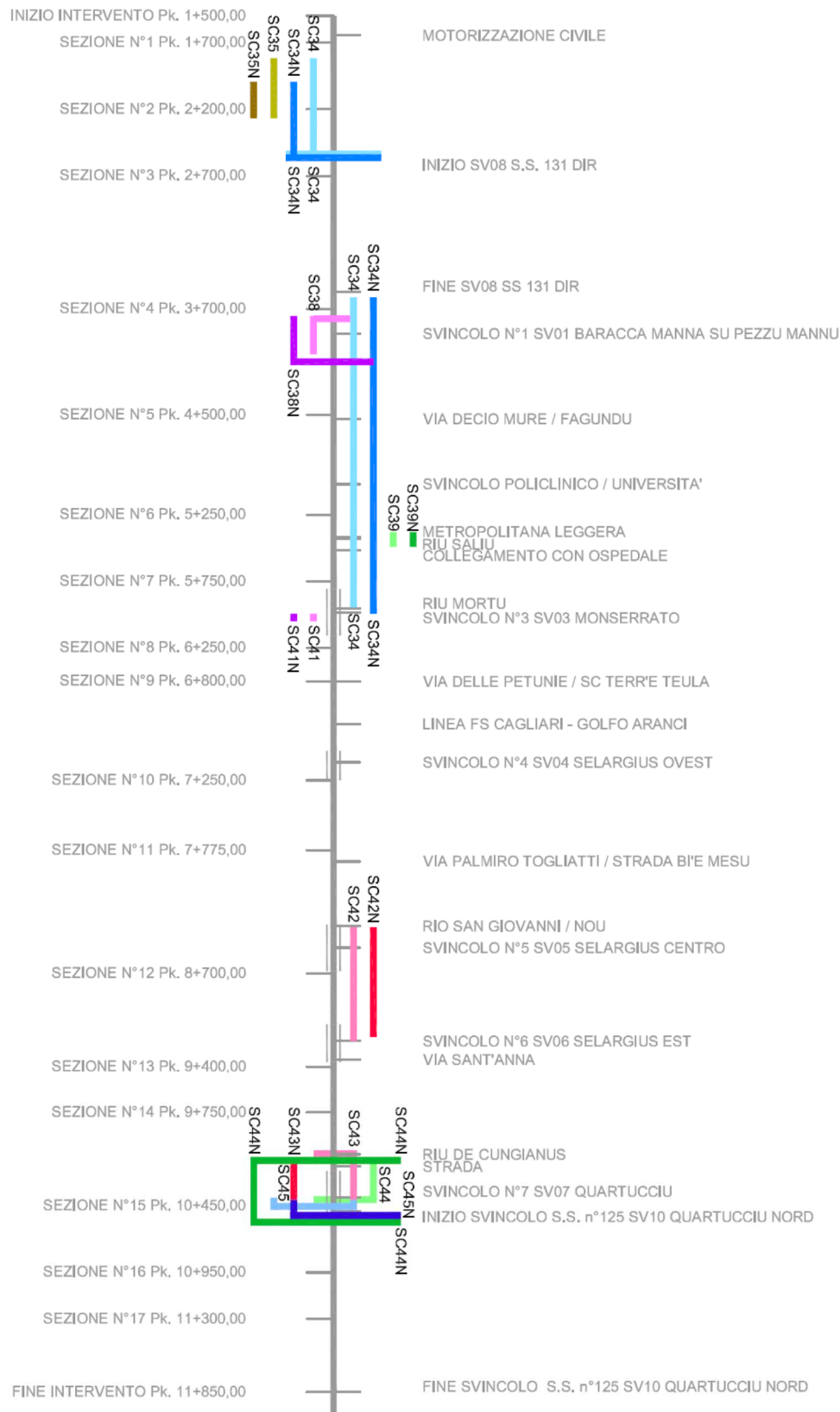
Figura 2. Schema interferenze idriche - Fognature
