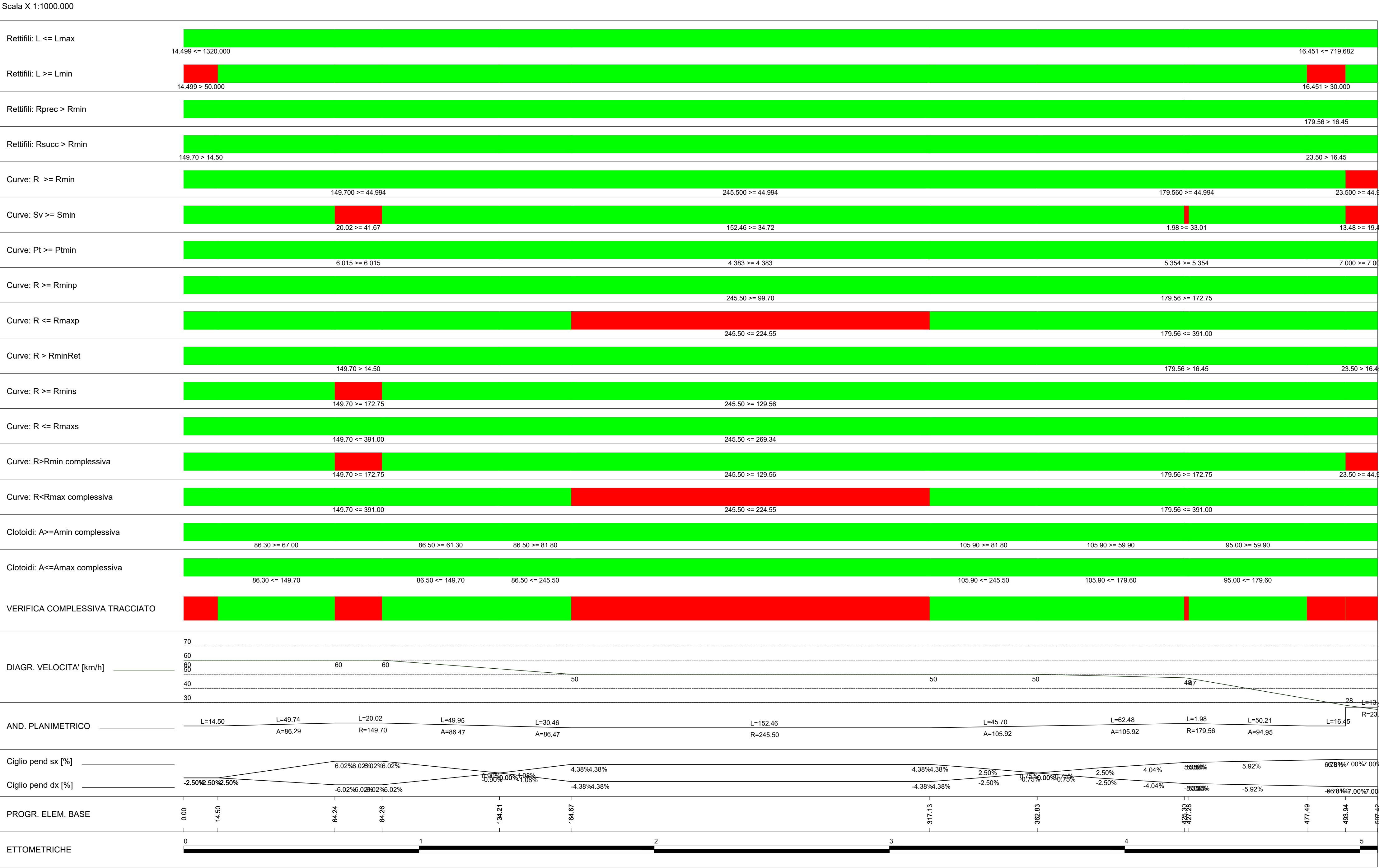
DIAGRAMMA DI VERIFICA GEOMETRICA COMPLESSIVA DEL TRACCIATO. RAMPA 3
