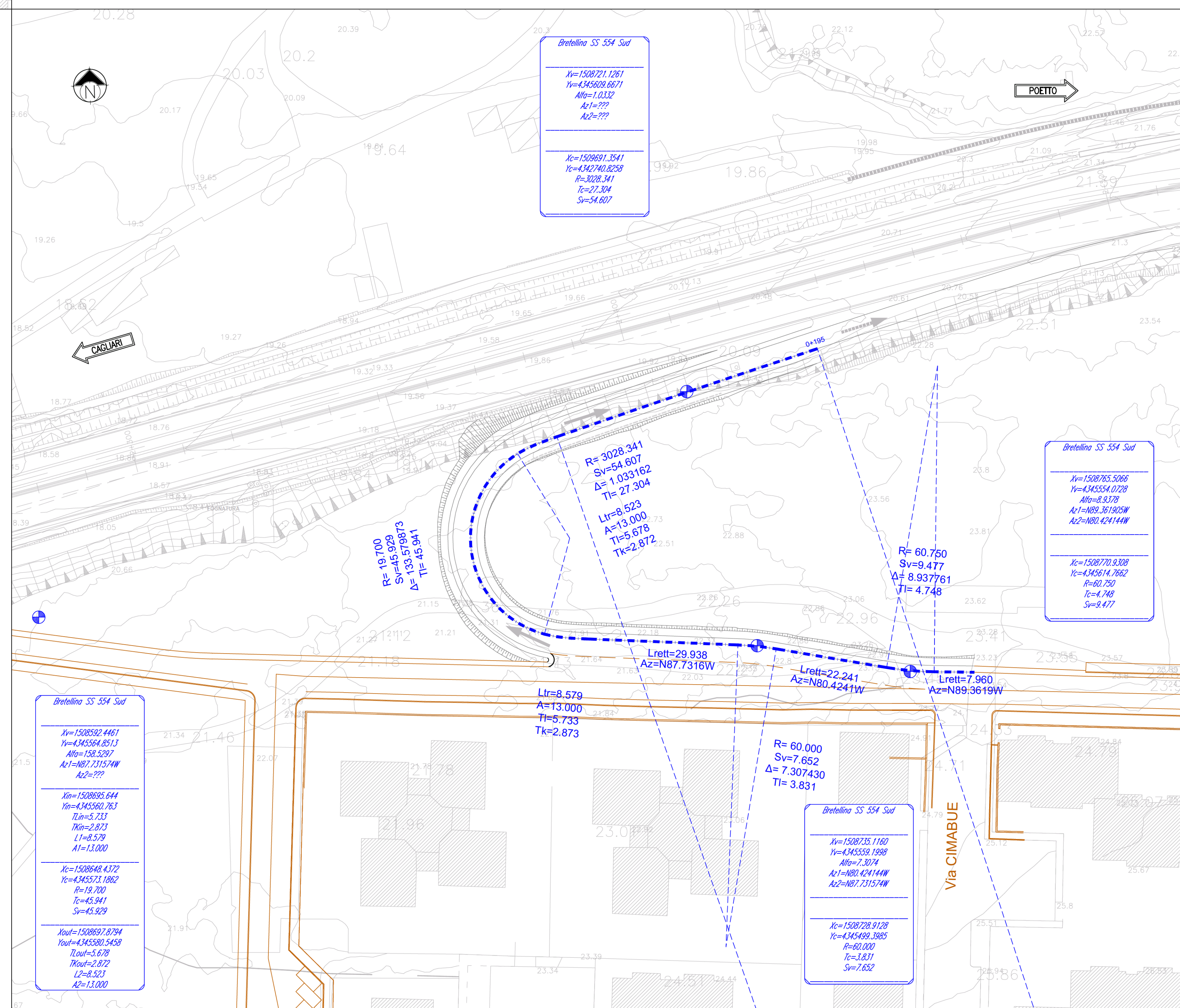
PLANIMETRIA DI TRACCIAMENTO scala 1:500
