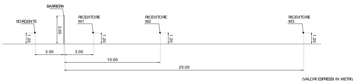
Figura B: schema della prova in campo libero
