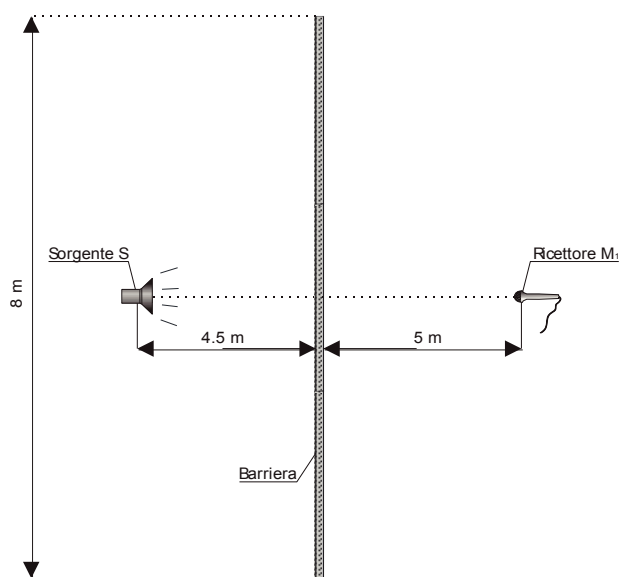
PLANIMETRIA SCHEMATICA
