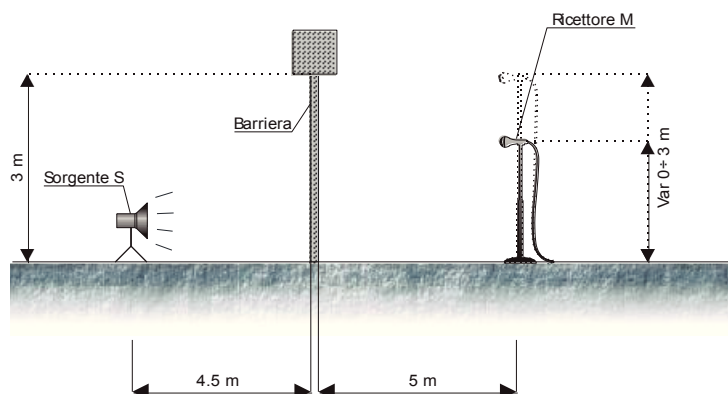
Figura F: schema della prova su elementi antidiffrattivi
