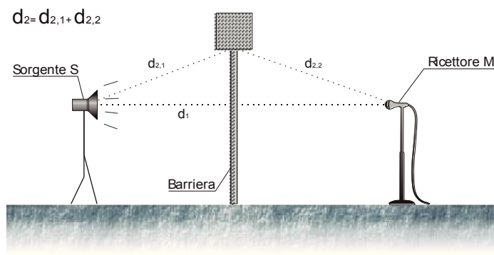
Figura E: schema per il calcolo dei valori di IL
