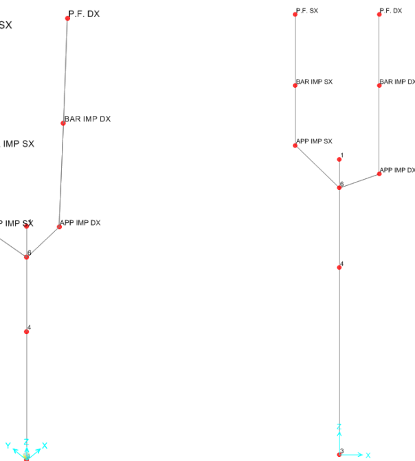
Figura 8.1 Vista 3D (a sinistra) e frontale (a destra) del modello di calcolo utilizzato per il dimensionamento delle pile
