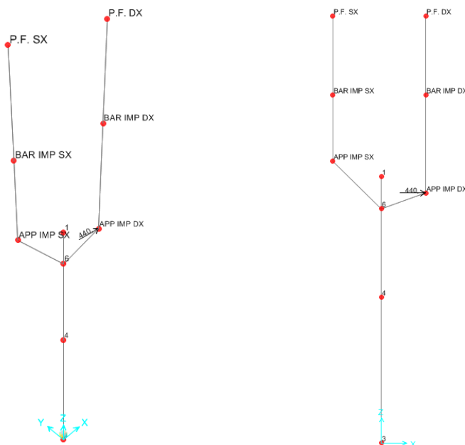
Figura 8.1 Vista 3D (a sinistra) e frontale (a destra) del modello di calcolo utilizzato per il dimensionamento delle pile
