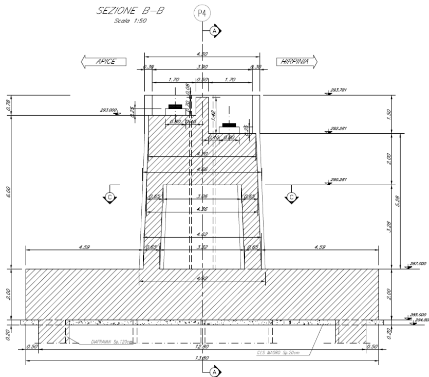
Figura 1 Sezione trasversale pila 4
