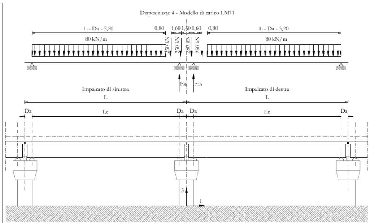
Figura 6.6 Disposizione di carico 4
