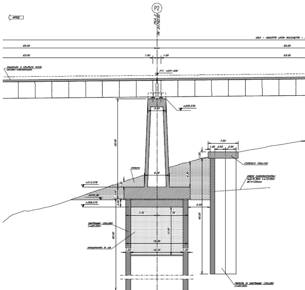
Figura 5.3 Vista globale longitudinale pila P02
