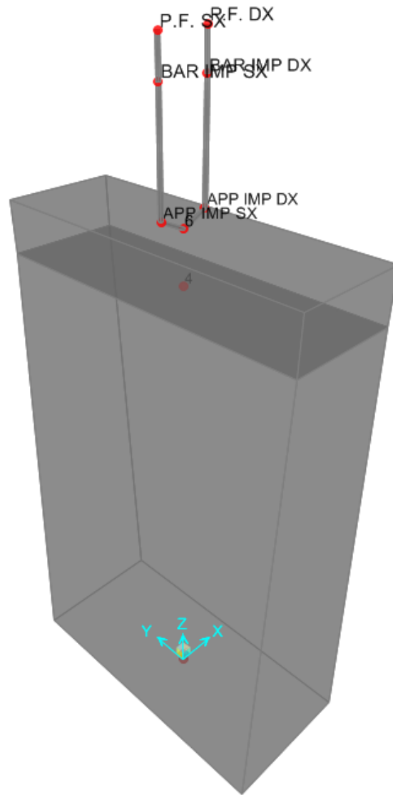
Figura 8.2 Vista estrusa del modello di calcolo delle pile
