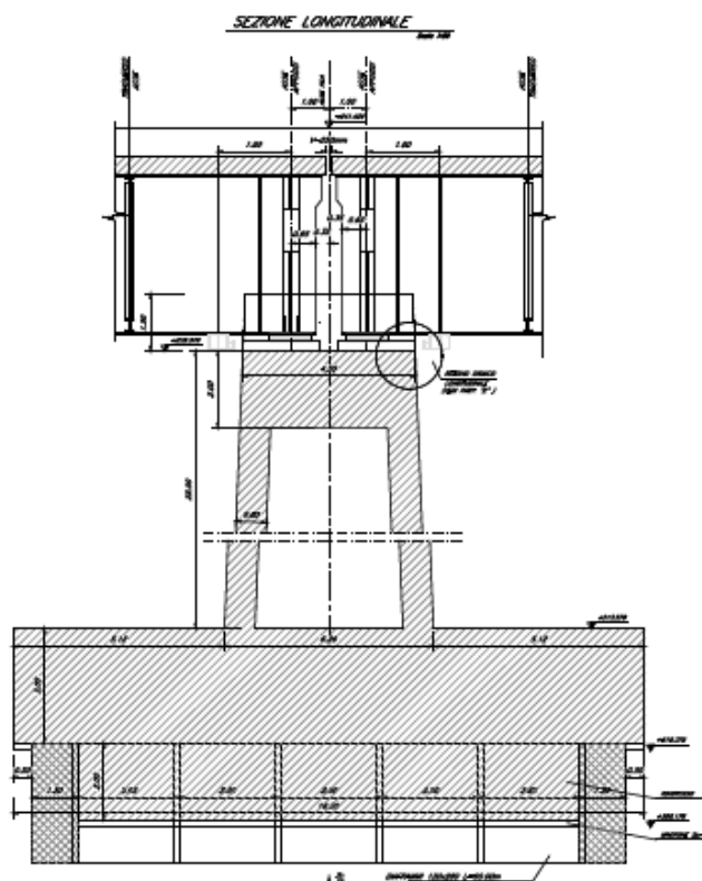
Figura 5.2 Sezione prospetto longitudinale Pila P02
