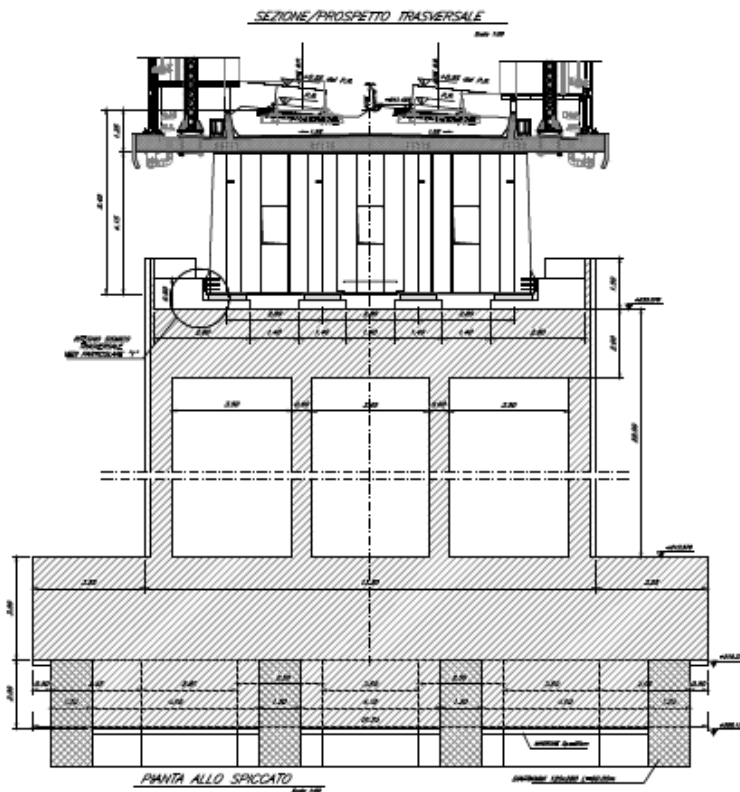
Figura 5.1 Sezione prospetto trasversale Pila P02
