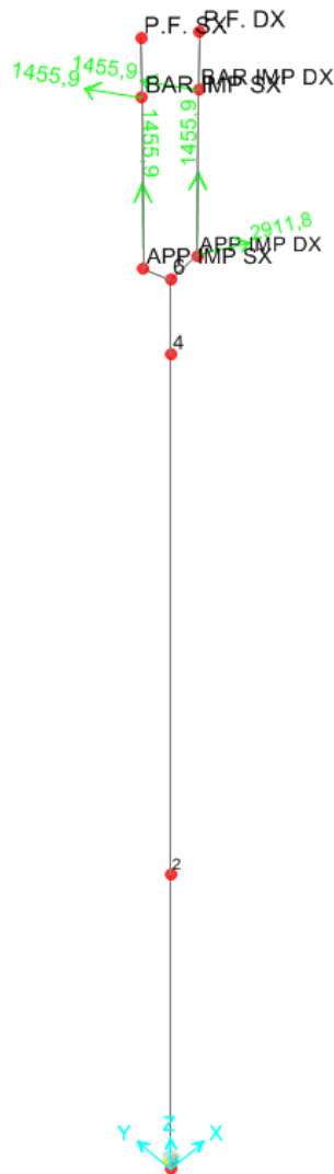
Figura 8.3 Assegnazione delle masse sismiche al modello di calcolo
