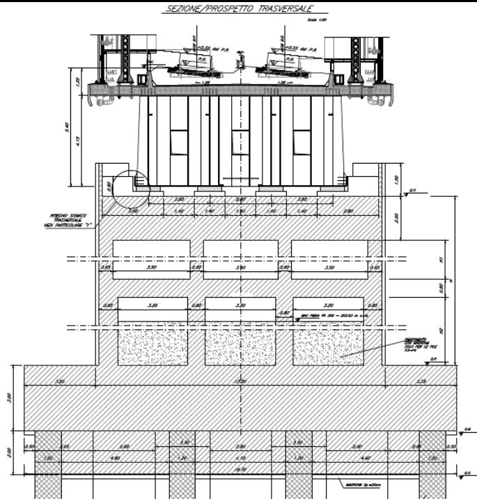
Figura 5.1 Sezione prospetto trasversale Pila P03
