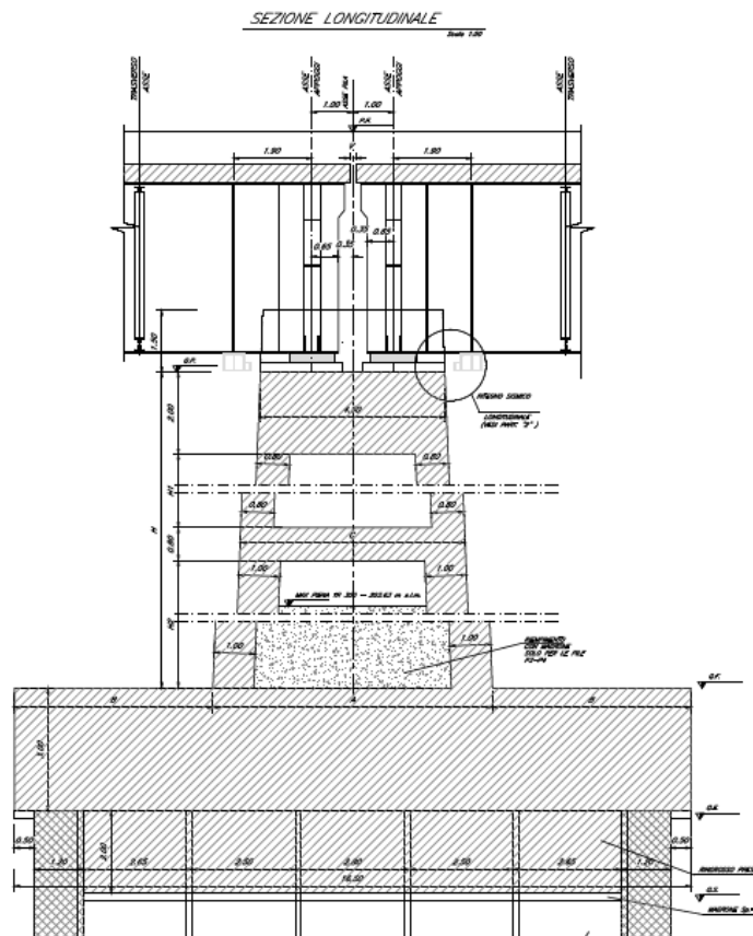
Figura 5.2 Sezione prospetto longitudinale Pila P03
