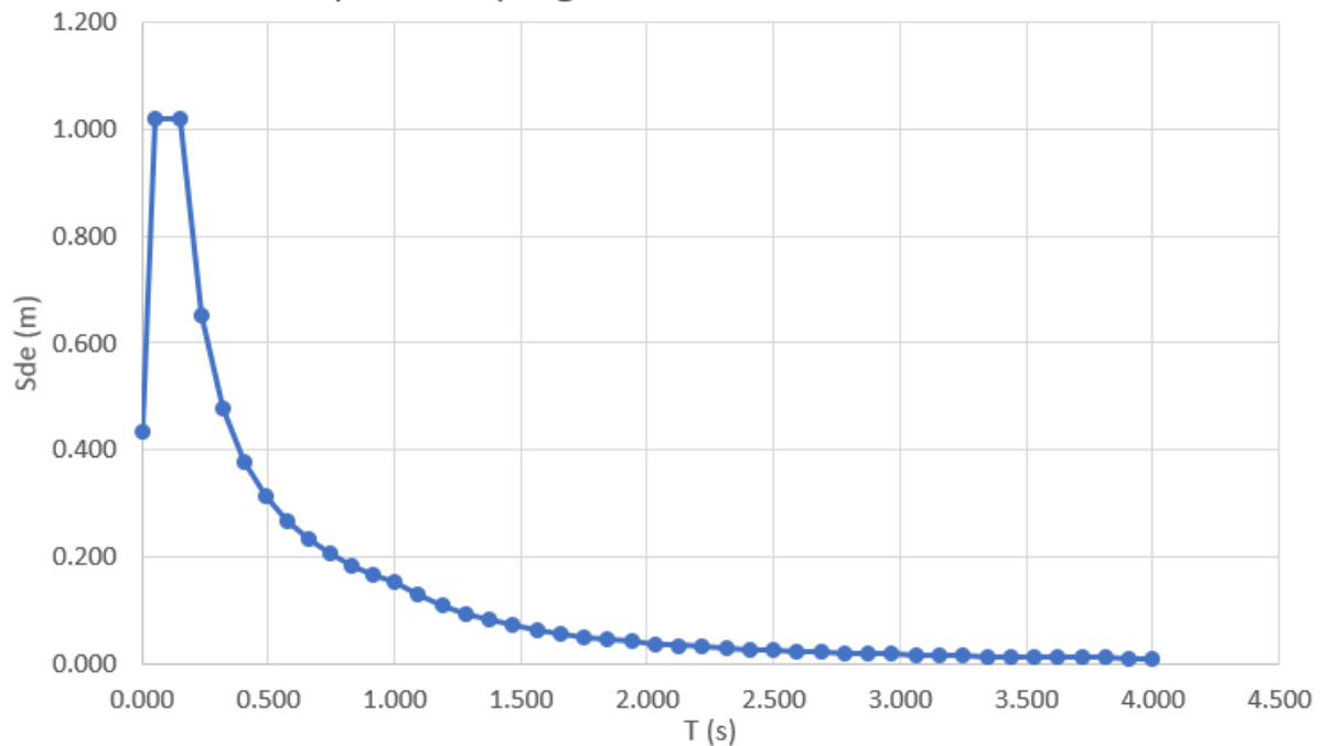
Figura 6.20 Spettro di progetto di risposta nelle componenti verticali di accelerazione per lo SLV
