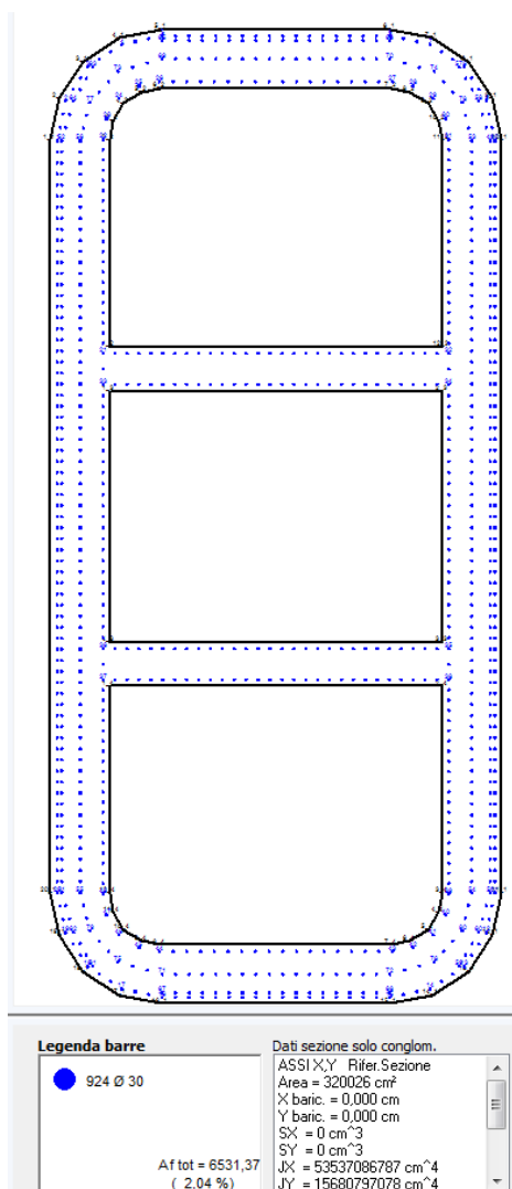
Figura 9.2 Disposizione dell'armatura verticale
