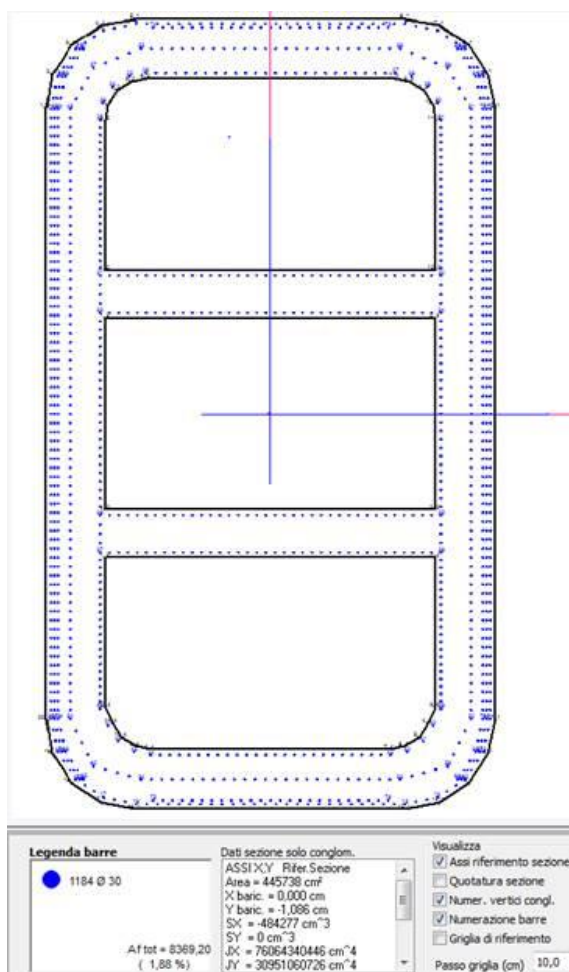
Figura 9.1 Disposizione dell'armatura verticale
