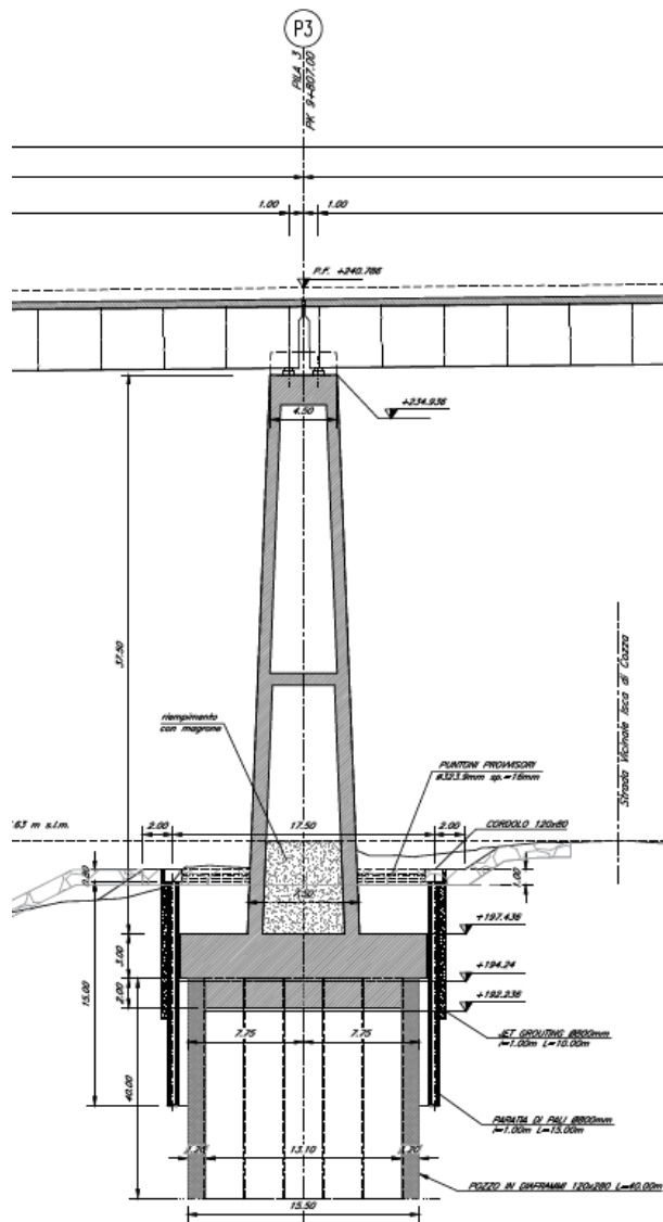
Figura 5.3 Vista globale longitudinale pila P03
