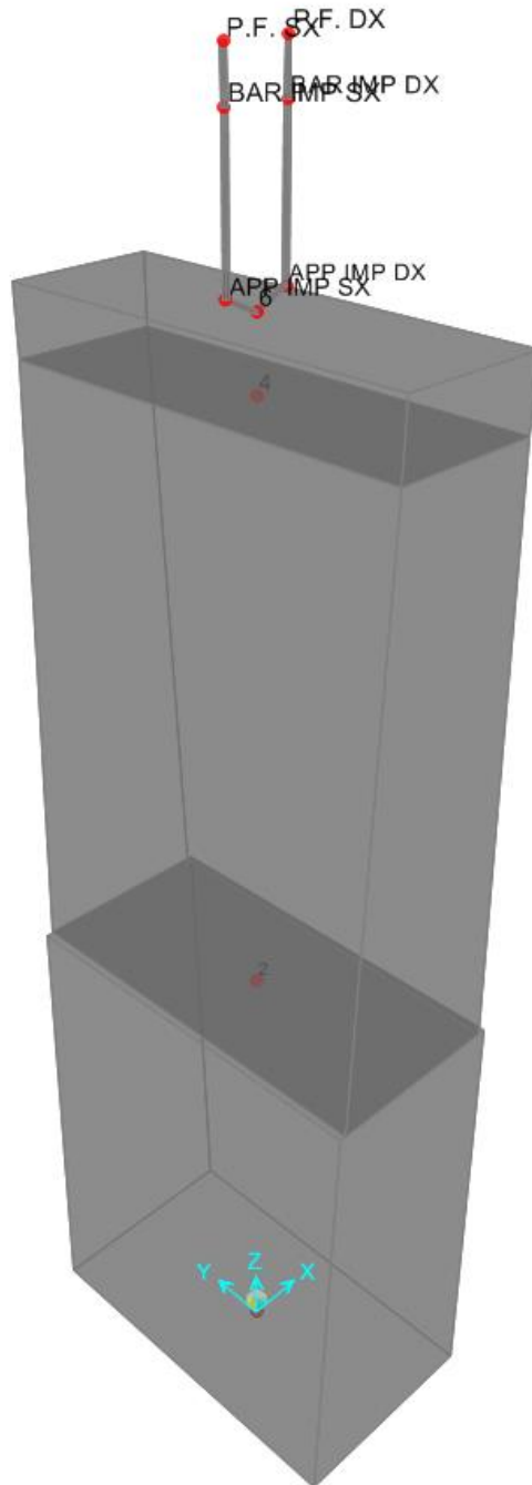
Figura 8.2 Vista estrusa del modello di calcolo delle pile
