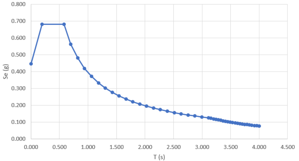
Figura 6.19 Spettro di progetto di risposta nelle componenti orizzontali di accelerazione per lo SLV
