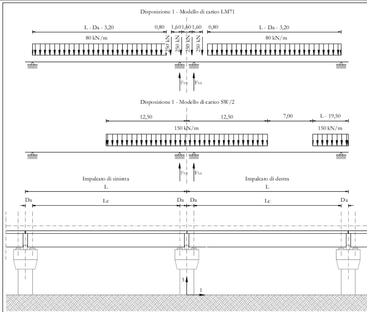
Figura 6.3 Disposizione di carico 1
