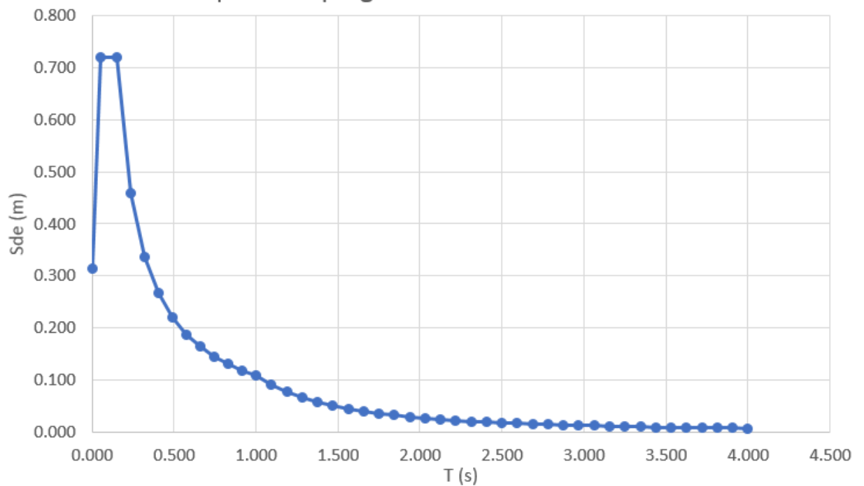
Figura 6.20 Spettro di progetto di risposta nelle componenti verticali di accelerazione per lo SLV
