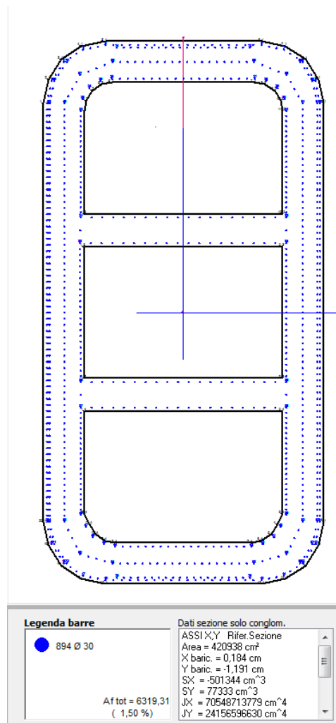
Figura 9.1 Disposizione dell'armatura verticale
