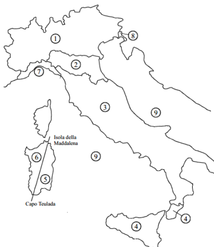
Figura 6.10 Mappa delle zone in cui è suddiviso il territorio italiano (Fig. 3.3.1 NTC08)
