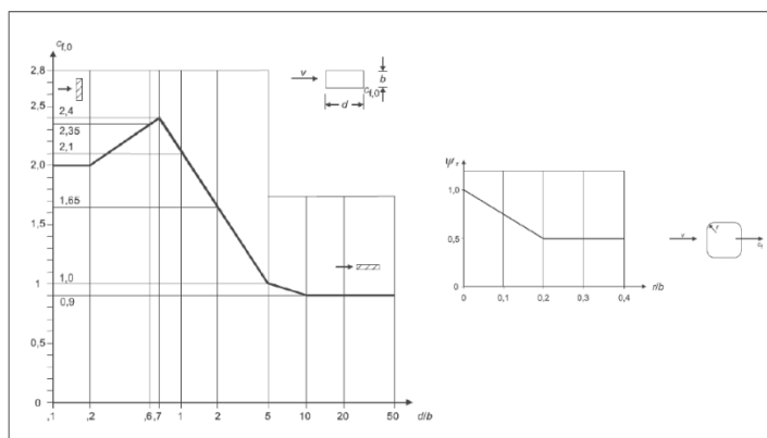
Figura 6.13 – Determinazione del coefficiente di forma c_{f,0} in funzione delle dimensioni della sezione (fig. 7.23 EC1-4) e correlazione tra il raggio di arrotondamento dello spigolo e il fattore riduttivo \psi_r (fig. 7.24 EC1-4)
