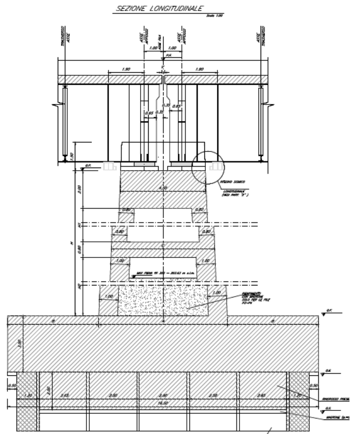
Figura 5.2 Sezione prospetto longitudinale Pila P05
