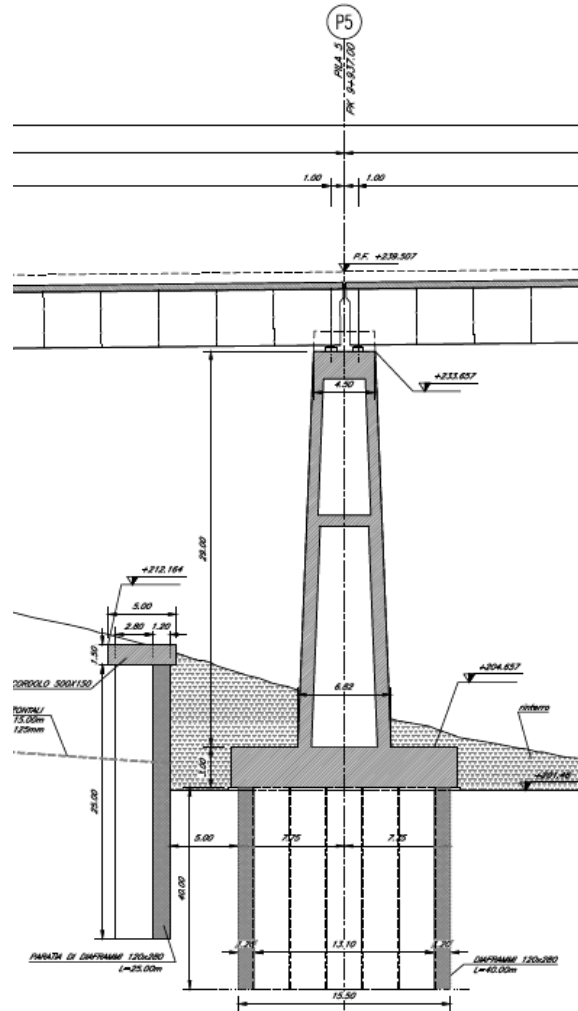
Figura 5.3 Vista globale longitudinale pila P05
