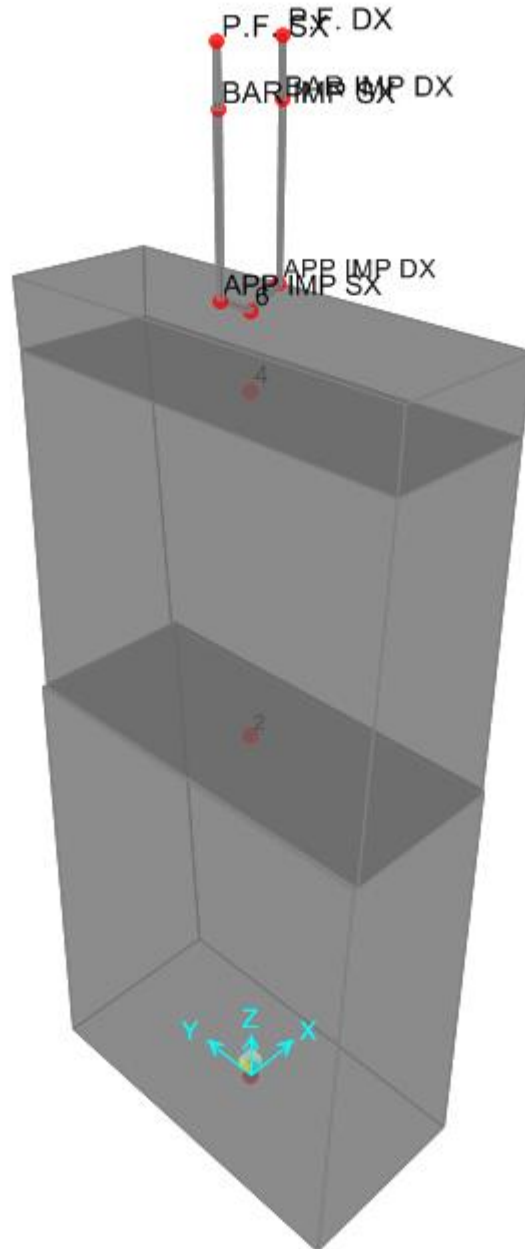
Figura 8.2 Vista estrusa del modello di calcolo delle pile
