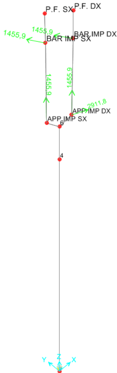
Figura 8.3 Assegnazione delle masse sismiche al modello di calcolo
