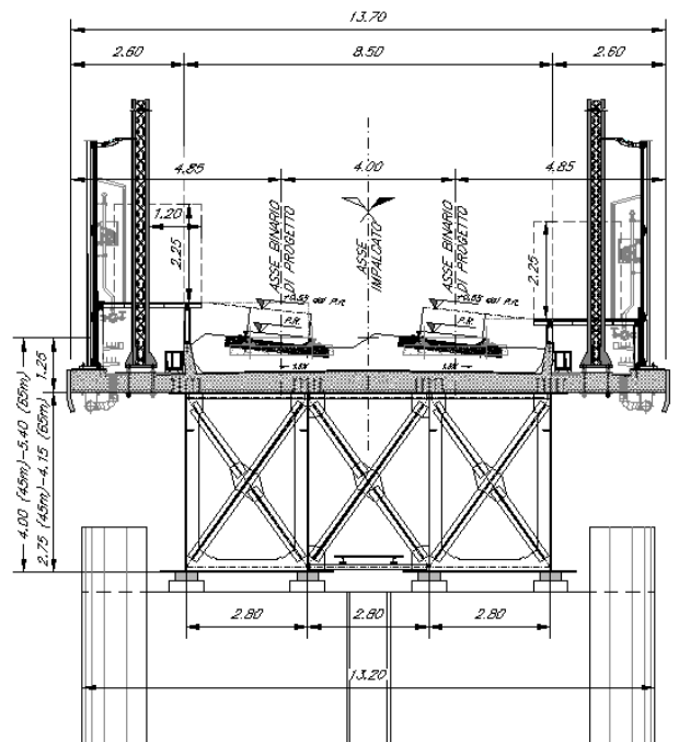
Figura 6.1 sezione trasversale impalcato L=65m
