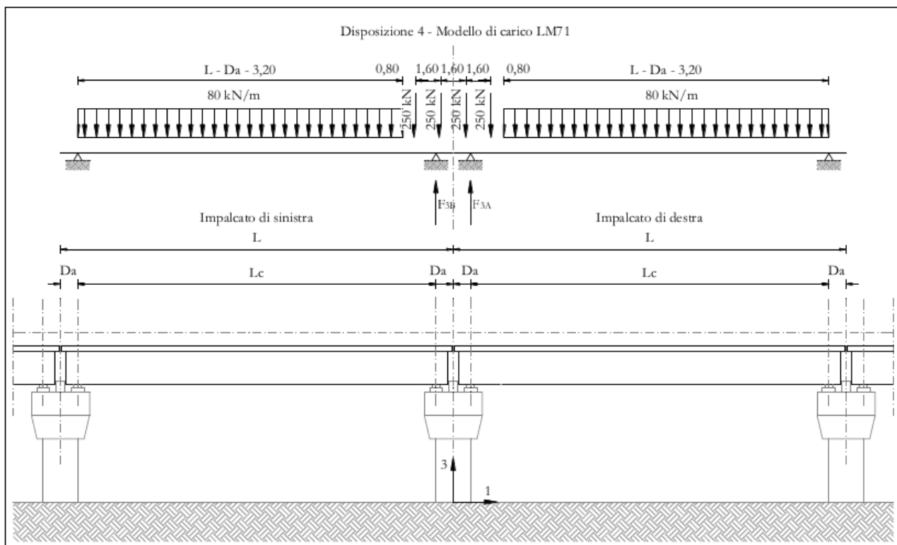
Figura 6.6 Disposizione di carico 4
