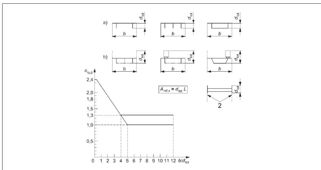
Figura 6.11 coefficiente di forza c_{fx,0} in funzione della geometria dell'impalcato (fig. 8.3 EC1-4)
