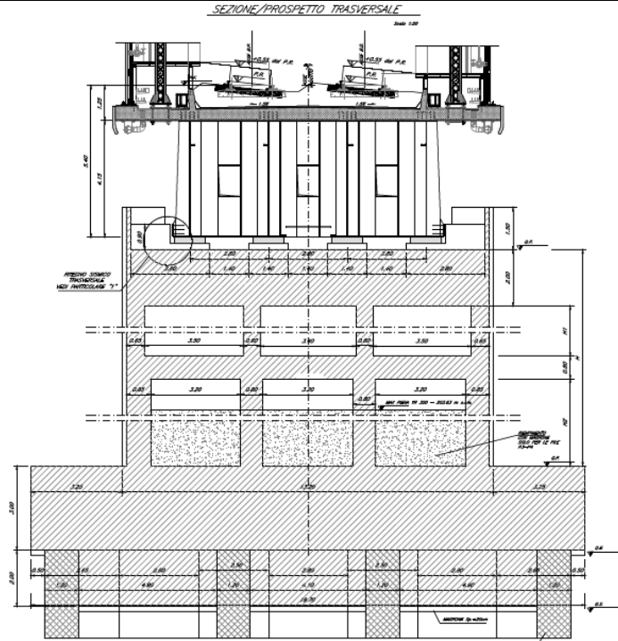
Figura 5.1 Sezione prospetto trasversale Pila P05
