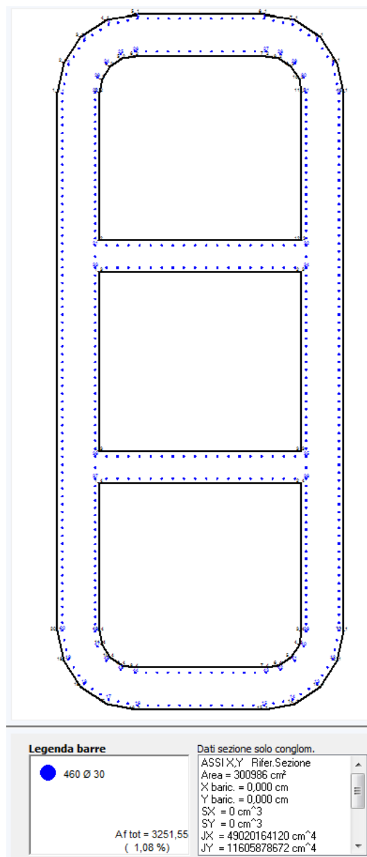
Figura 9.2 Disposizione dell'armatura verticale
