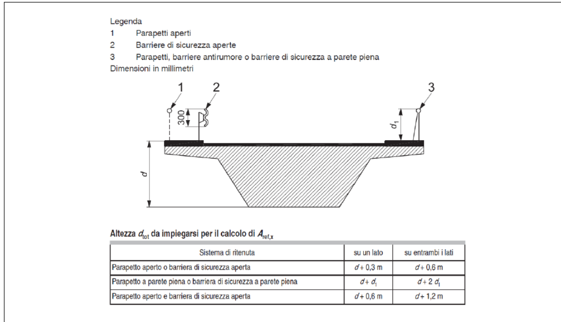
Figura 6.12 criteri per la determinazione di d (fig 8.5 EC1-4)
