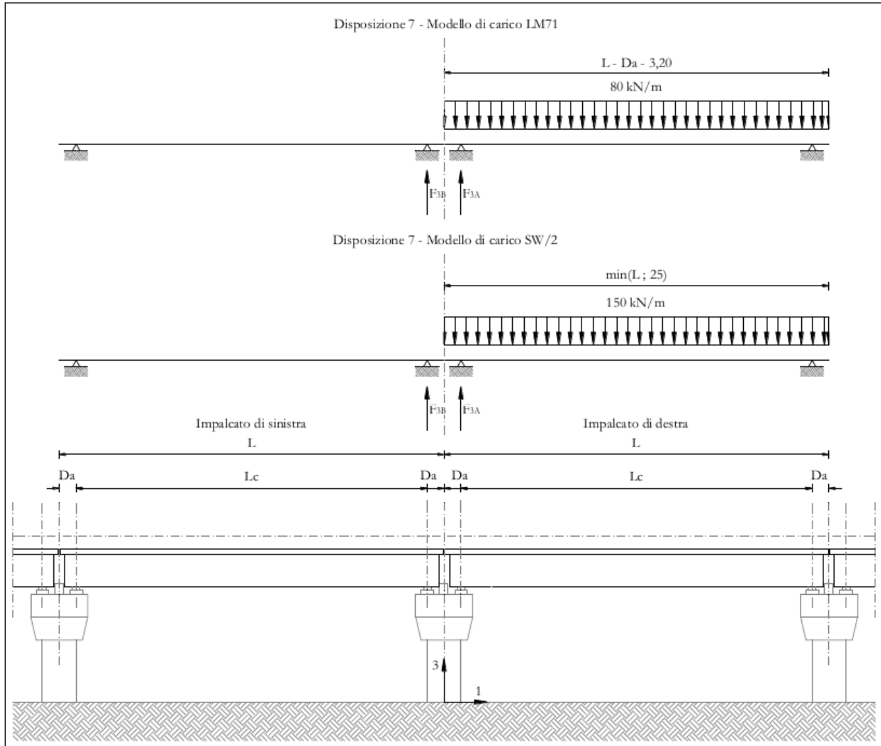
Figura 6.9 Disposizione di carico 7
