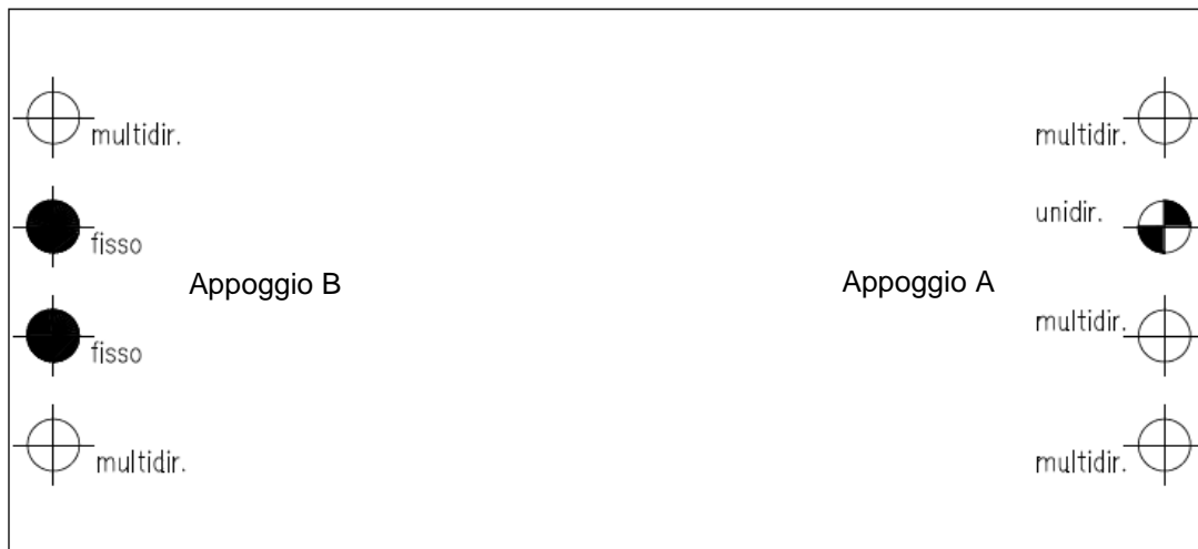
Figura 6.2 Schema degli appoggi degli impalcati
