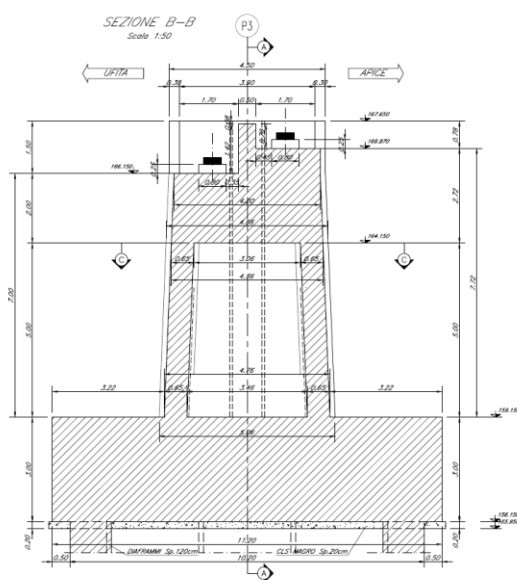
Figura 1 sezione trasversale pila 3
