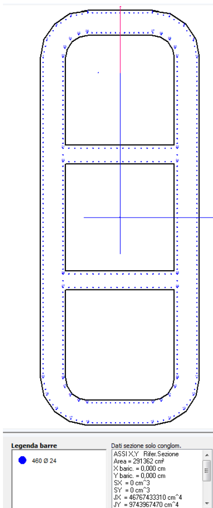
Figura 9.1 Disposizione dell'armatura verticale
