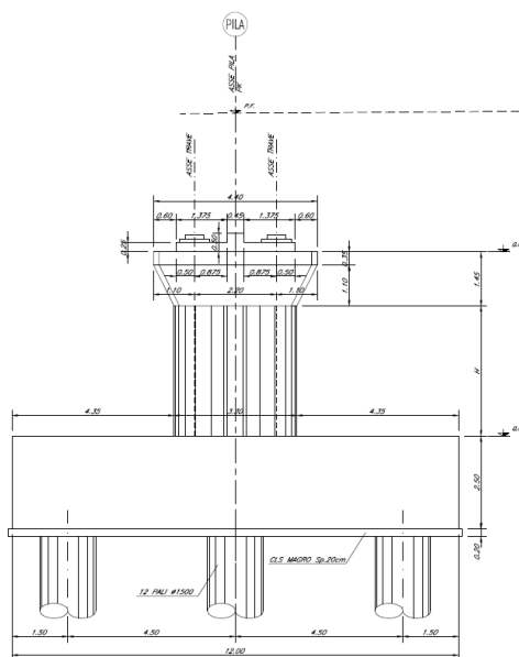
Figura 1 Sezione trasversale pila 7
