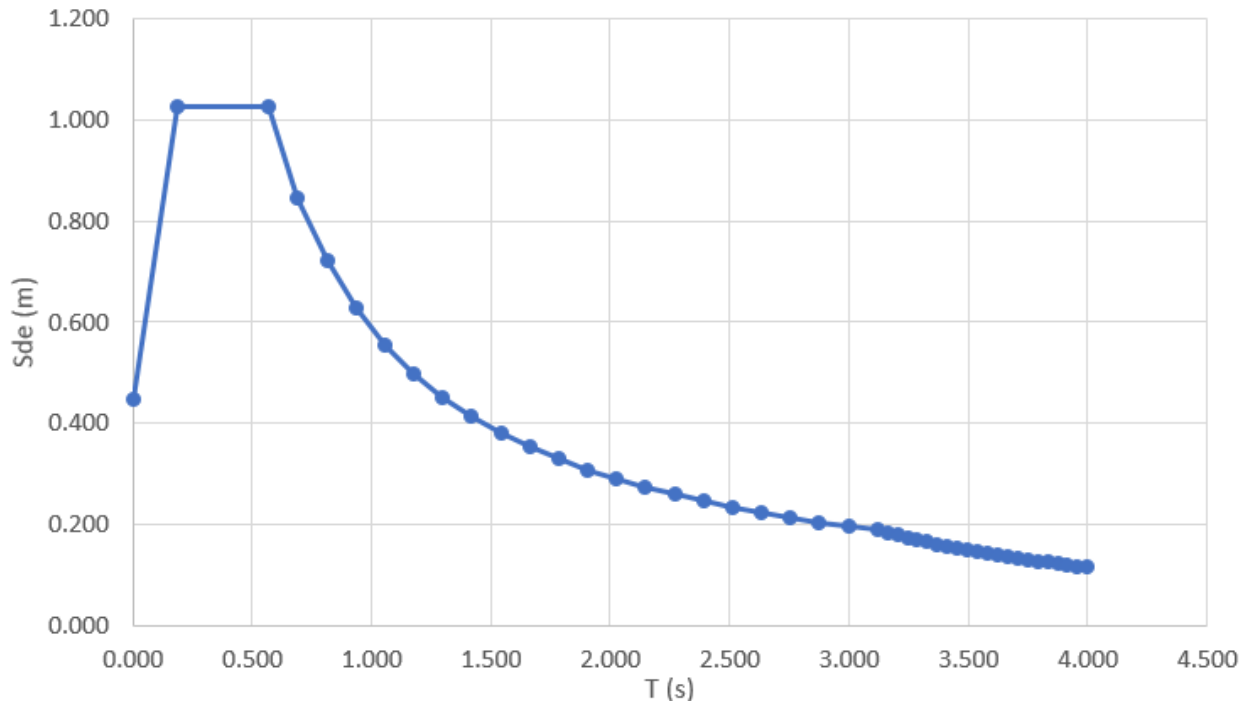
Figura 6.19 Spettro di progetto di risposta nelle componenti verticali di accelerazione per lo SLV
