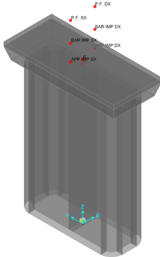
Figura 8.2 Vista estrusa del modello di calcolo delle pile
