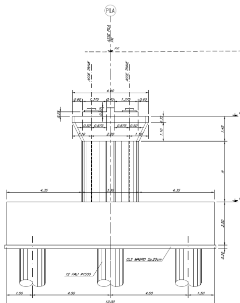
Figura 1 Sezione trasversale pila 17
