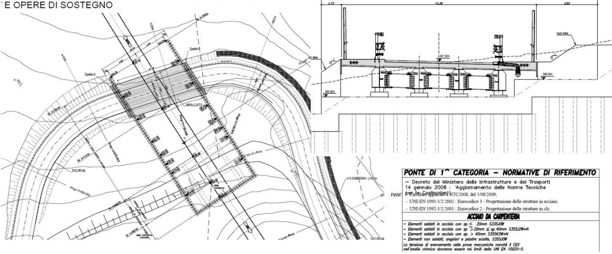
Figura 3-2. Planimetria e profilo NV05 deviazione provvisoria
