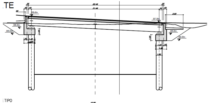
Figura 3-5. Rappresentazione grafica opere di sostegno NV05
