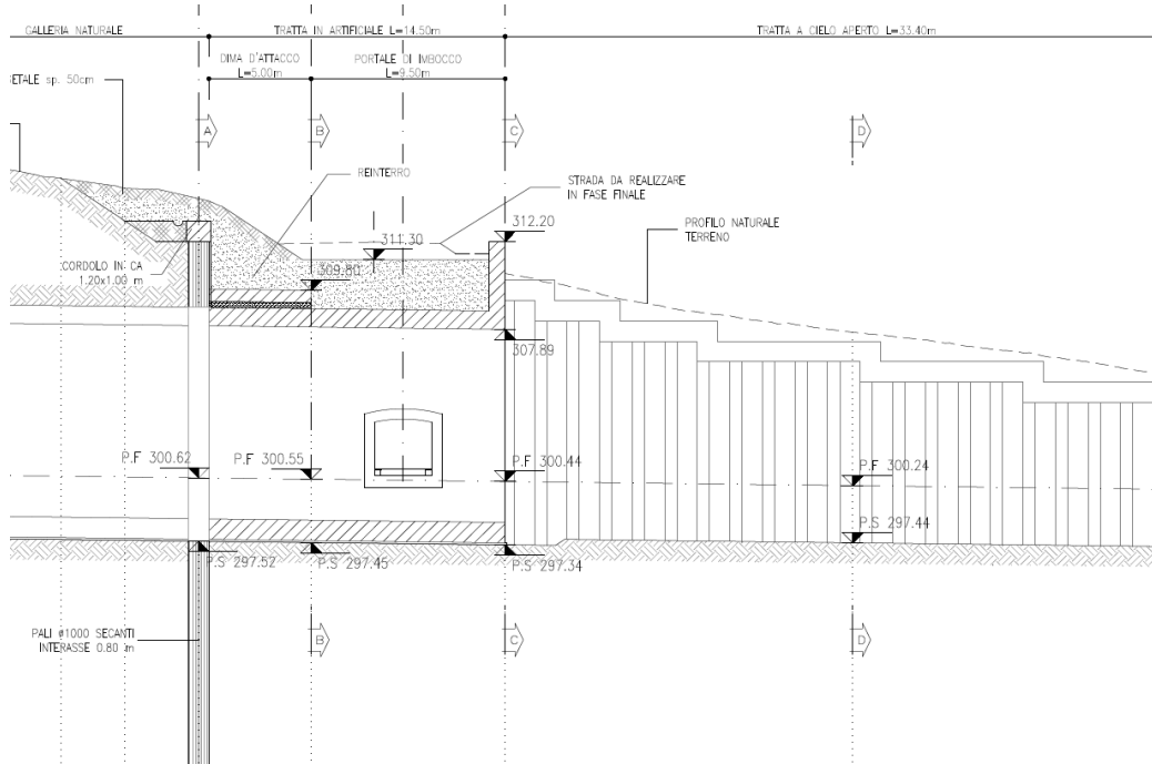
Figura 2-3. Sistemazione definitiva imbocco galleria Grottaminarda lato Napoli – Profilo longitudinale - PD
