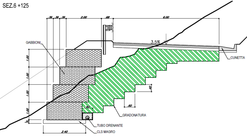
Figura 3-3. Rappresentazione grafica opere di sostegno NV05 – gabbionate
