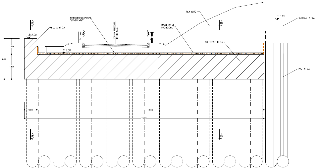
Fig. 2 – Soletta stradale – Profilo longitudinale
