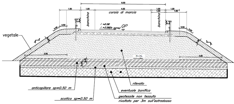
Figura 3-4. Sezione tipo in rilevato (sezione fuori sede) deviazione stradale NV05
