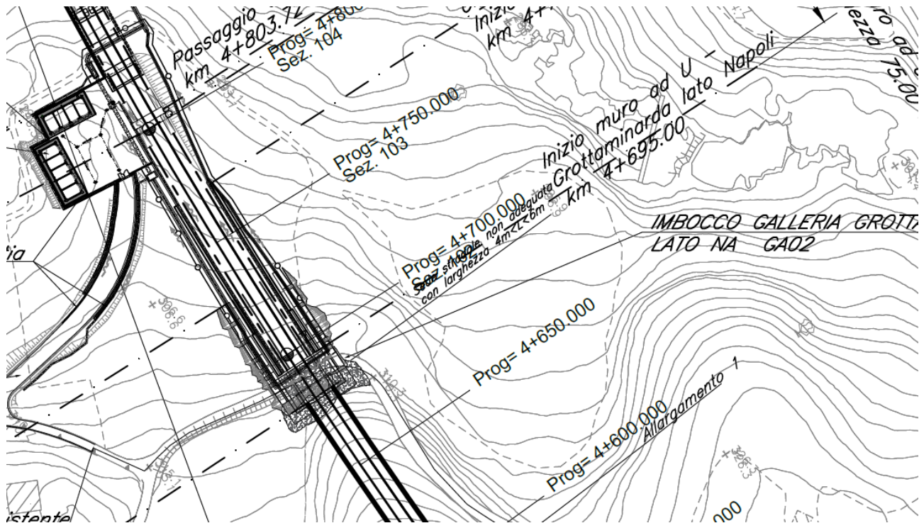
Figura 2-1. Planimetria di imbocco galleria Grottaminarda lato Napoli – PD
