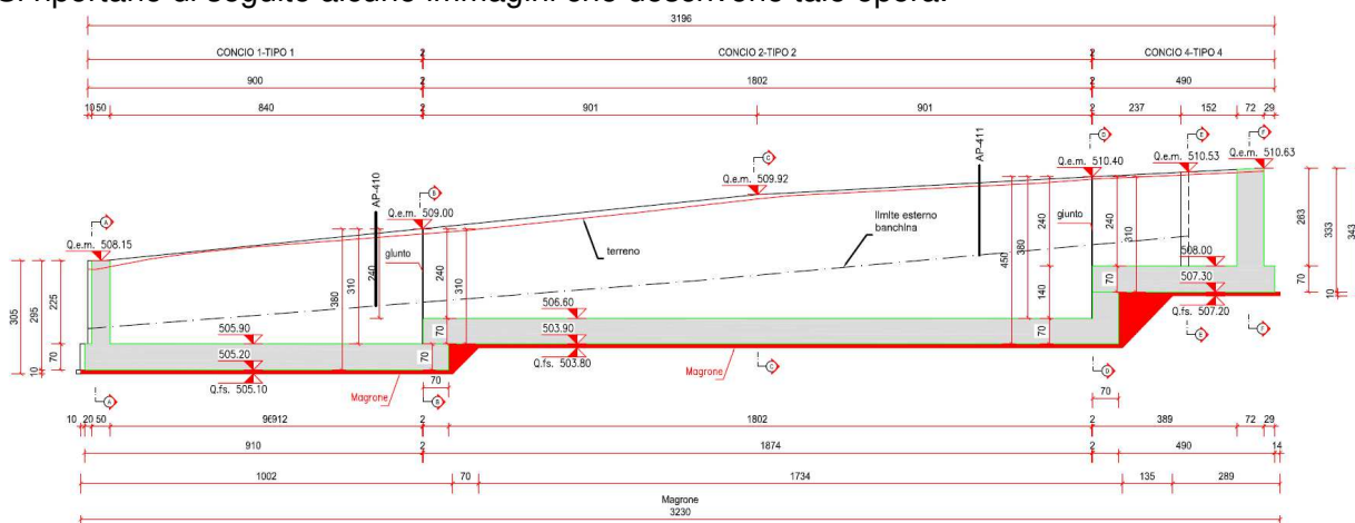
Fig. 1 Sezione longitudinale
