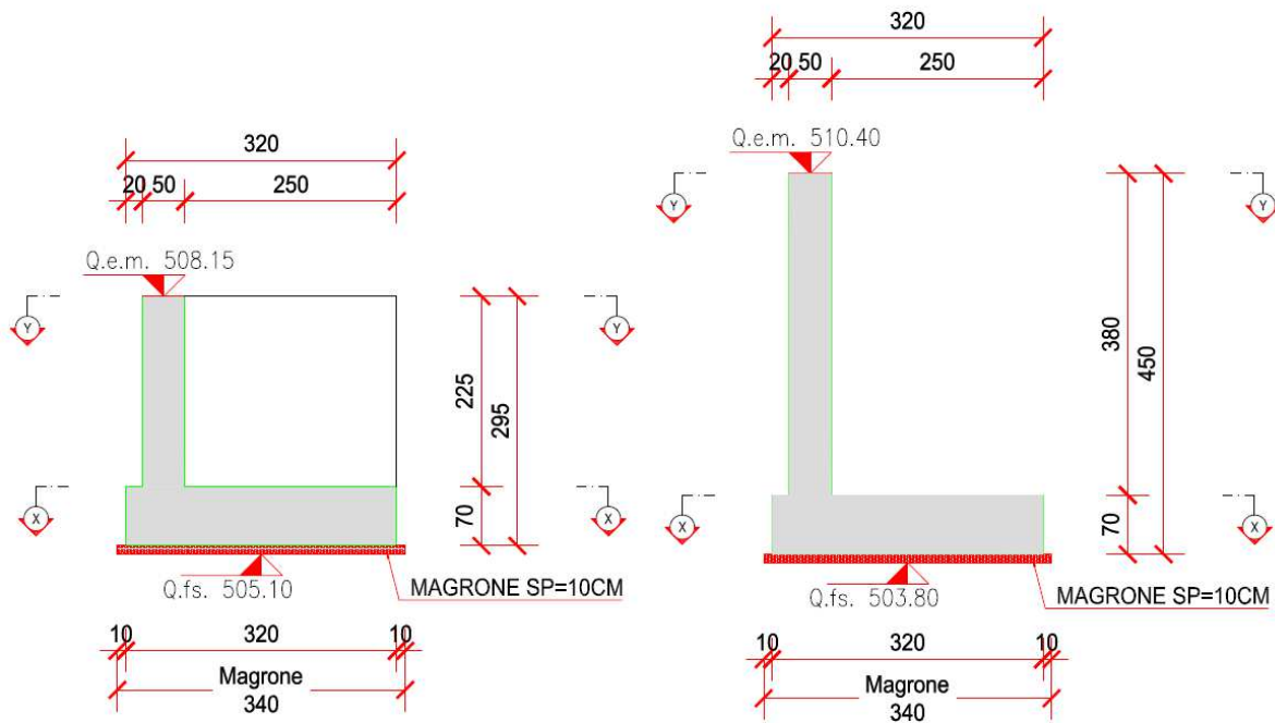
Fig. 2 Sezione trasversale inizio concio n. 1 e fine concio n. 2
