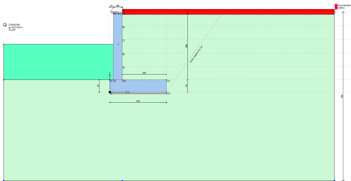
Fig. 7a Modello di calcolo
