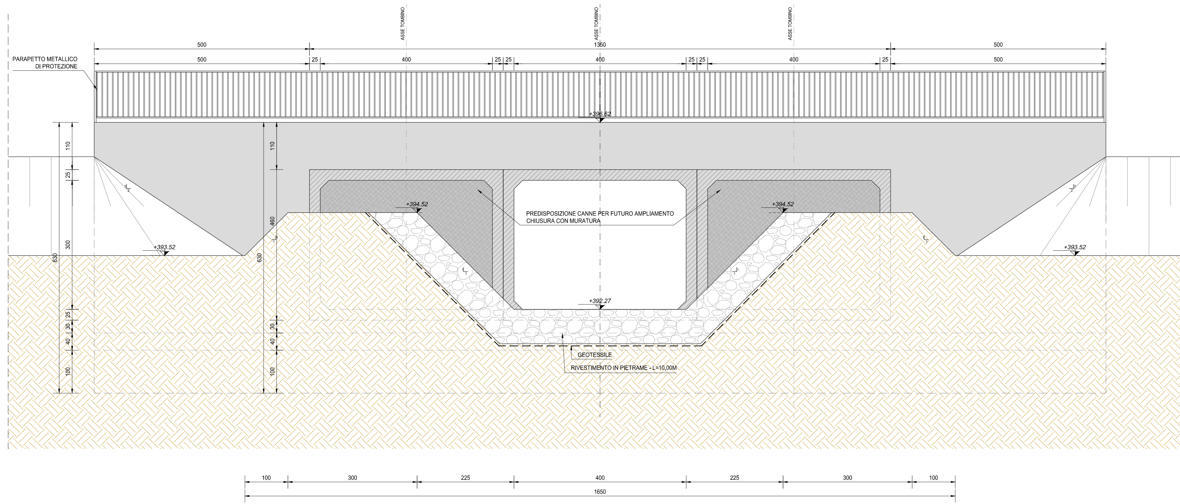
SEZIONE SEZ. E-E SCALA 1:50
