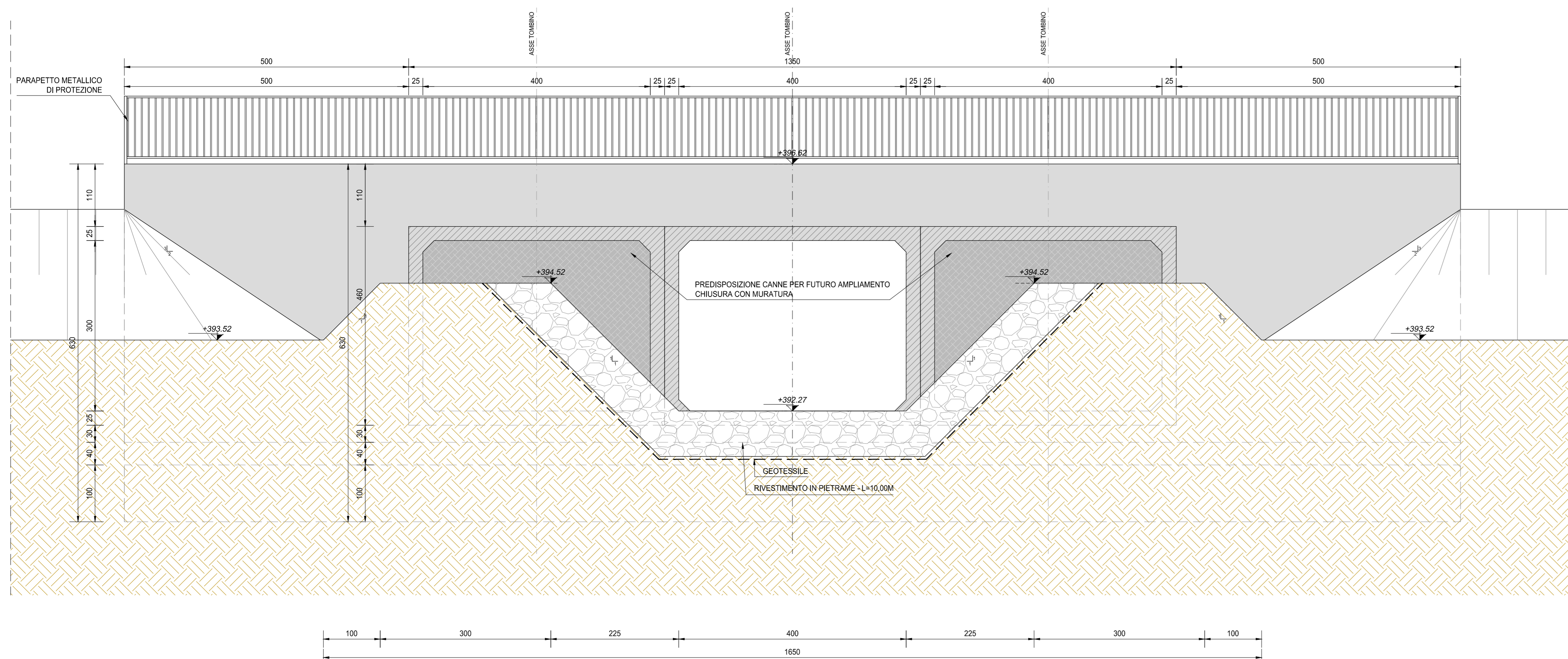
SEZIONE SEZ. E-E SCALA 1:50
