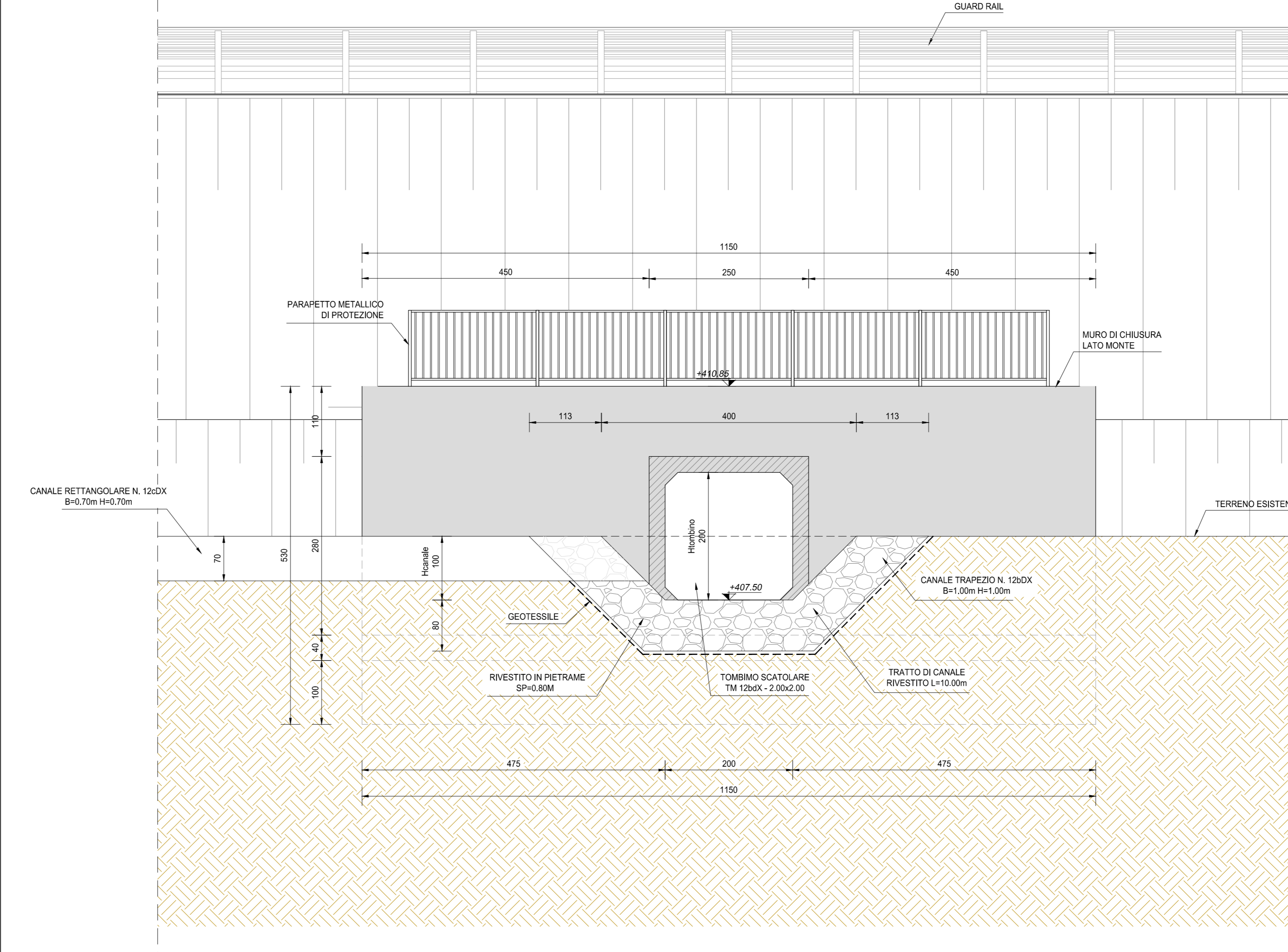
VISTA PROSPETTICA MURO DI ENTRATA LATO MONTE (SEZIONE B-B) SCALA 1:50
