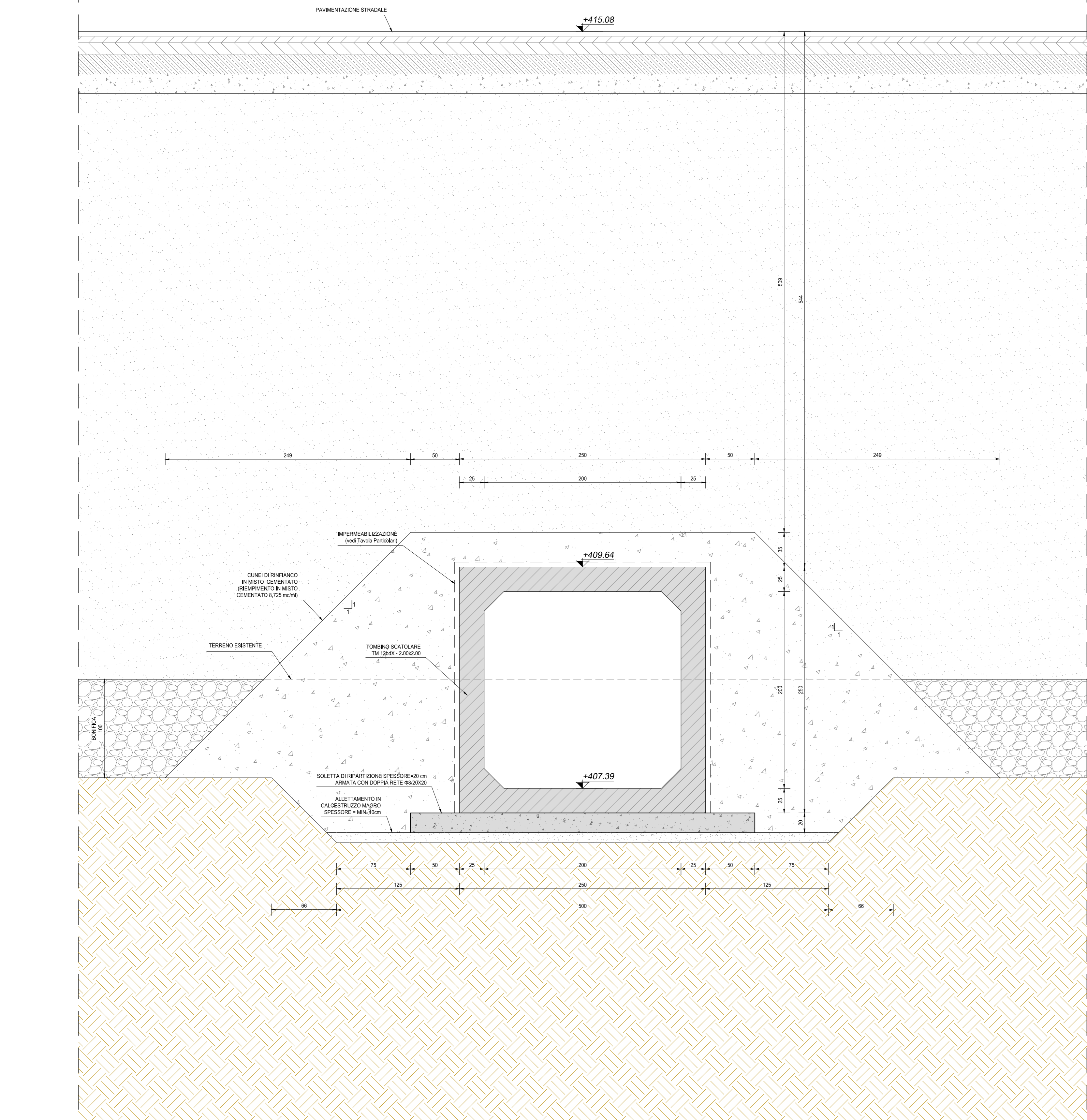
SEZIONE TRASVERSALE IN ASSE STRADA (SEZIONE C-C) SCALA 1:25
