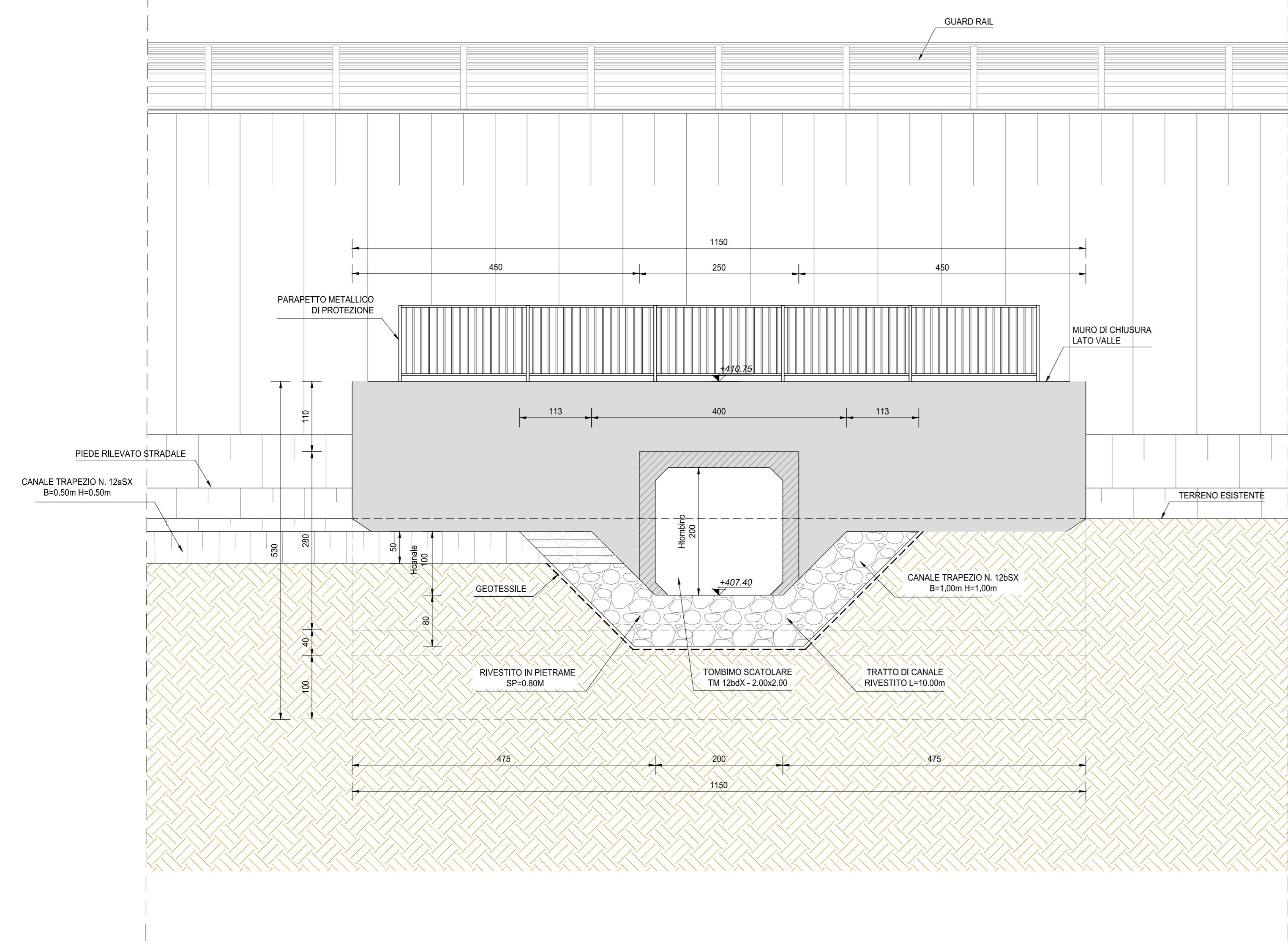
VISTA PROSPETTICA MURO DI USCITA LATO VALLE (SEZIONE D-D) SCALA 1:50
