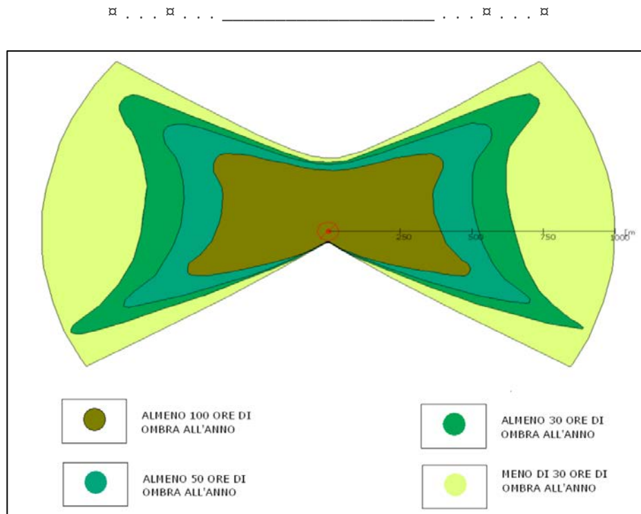
Figura 2: schema rappresentativo dell'evoluzione annuale tipo dell'ombra di un aerogeneratore
