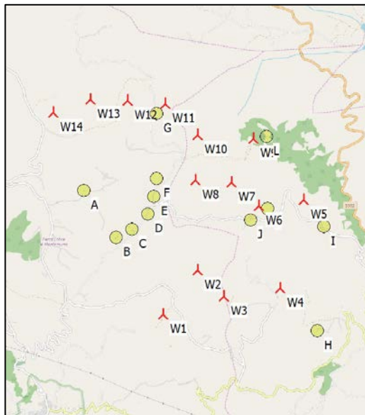
Figura 7: rappresentazione delle WTG e degli Shadow Receptor (WindPRO)
