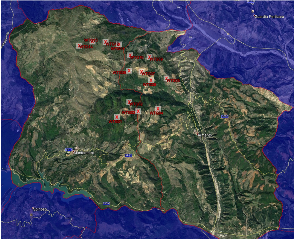
Figura 1: inquadramento territoriale dell'area da destinare alla realizzazione del parco eolico
