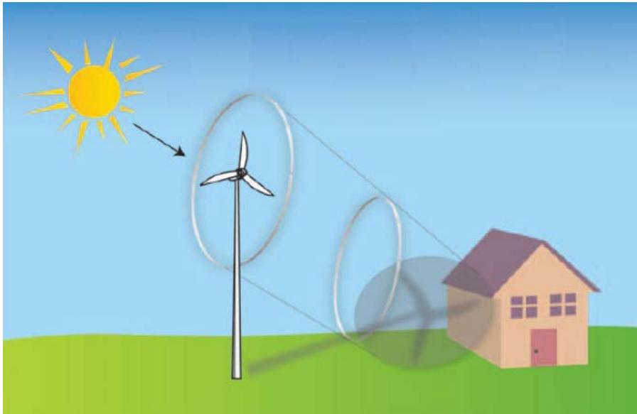
Figura 25. Illustrazione del fenomeno di shadow flickering
