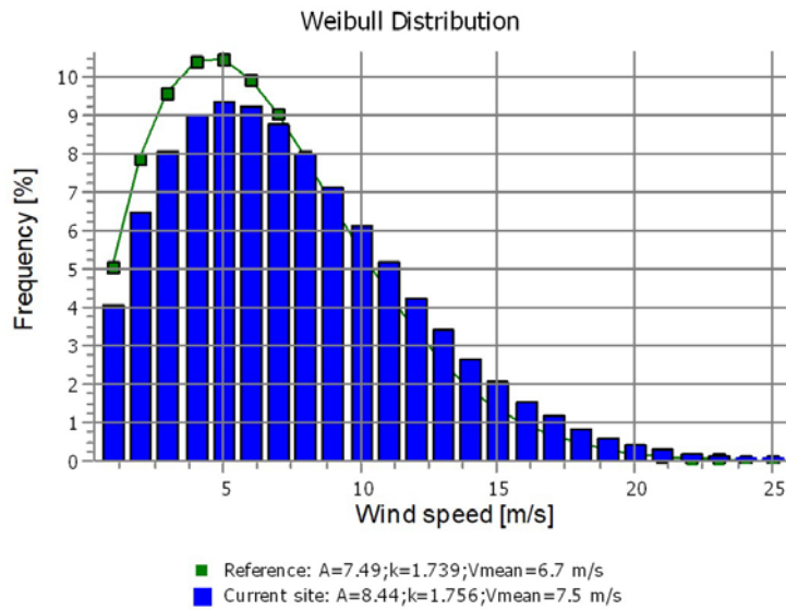
Figura 19. Curva di durata e distribuzione di frequenza della velocità del vento
