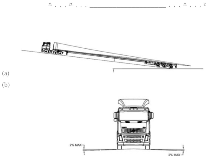
Figura 17. Illustrazioni prese dal “Wind farm Roads Requirements” della Vestas, relative alla pendenza longitudinale (a) e alla pendenza laterale della carreggiata (b).
