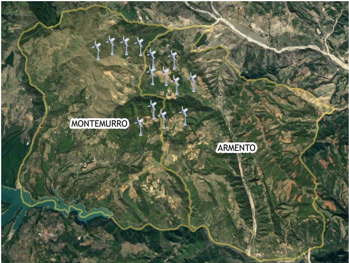
Figura 1: Inquadramento dell'area di realizzazione dell'impianto di 14 aerogeneratori per una potenza complessiva di 75 MW nell'agro dei comuni di Montemurro e Armento
