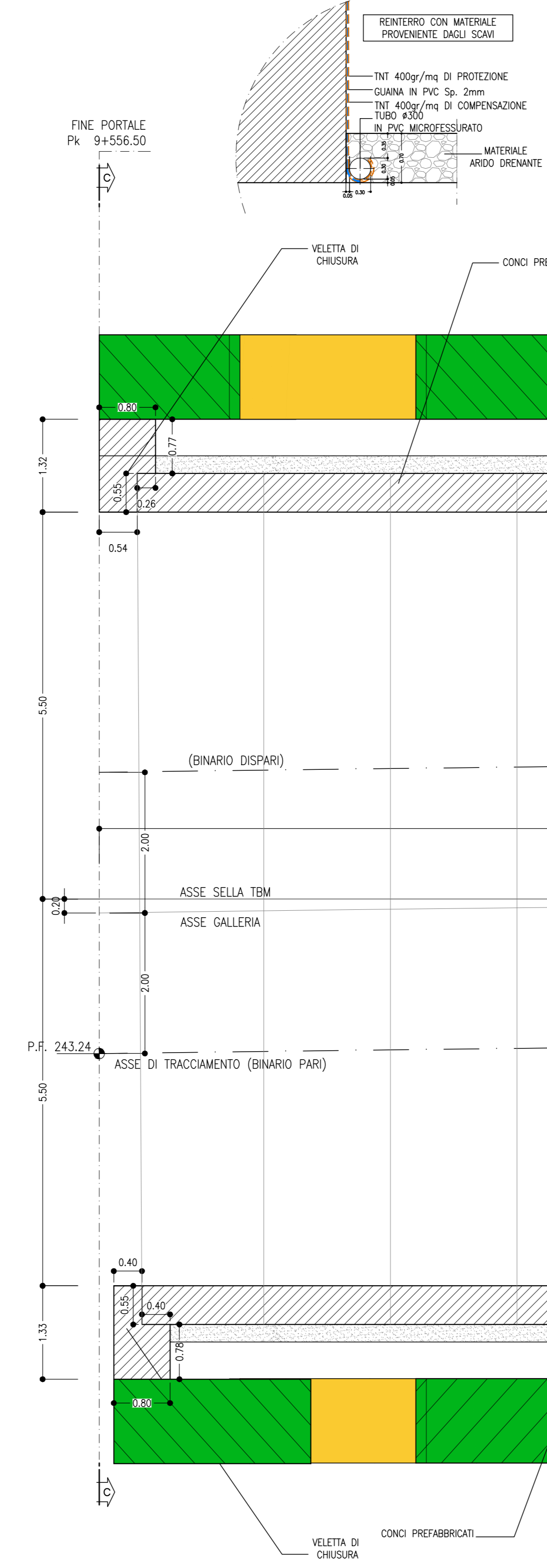
PARTICOLARE K SCALA 1:50 DETTAGLIO IMPERMEABILIZZAZIONE E DRENAGGIO
