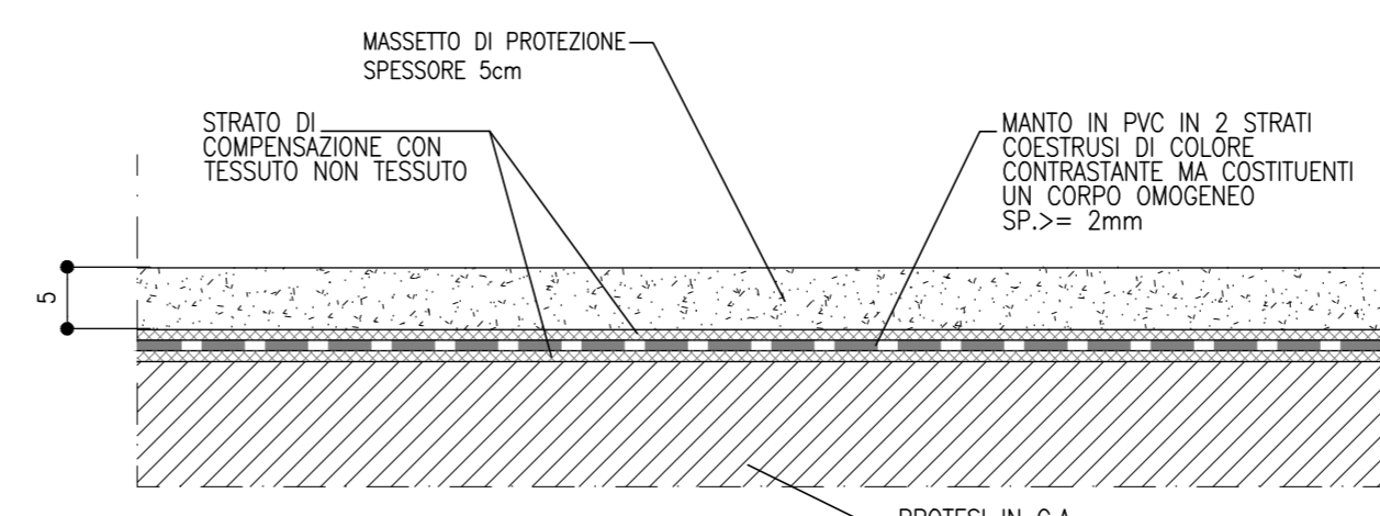
PARTICOLARE A SCALA 1:5 IMPERMEABILIZZAZIONE
