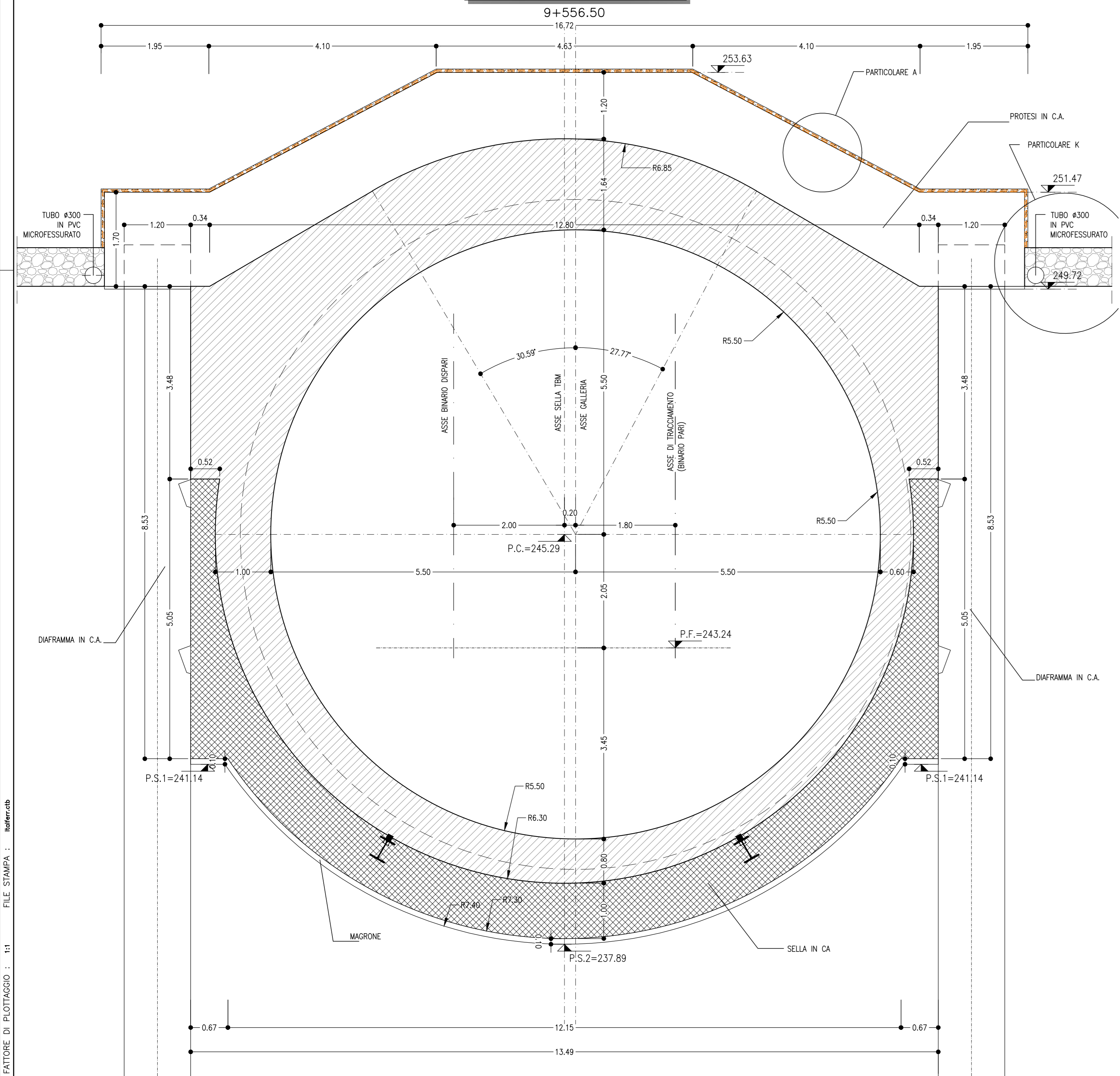
SEZIONE C-C SCALA 1:50 9+556.50
