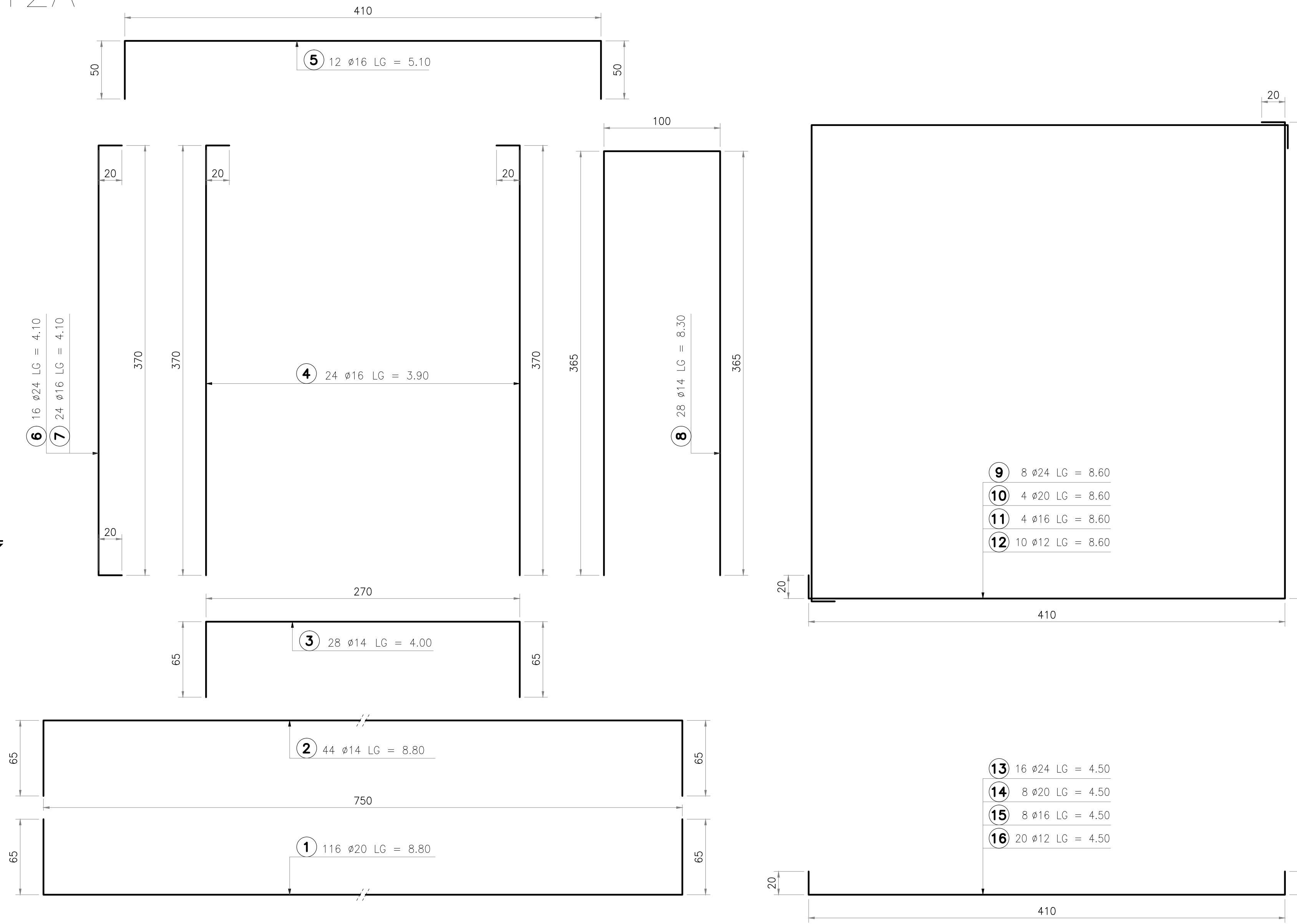
SEZIONE C-C (1:25)
