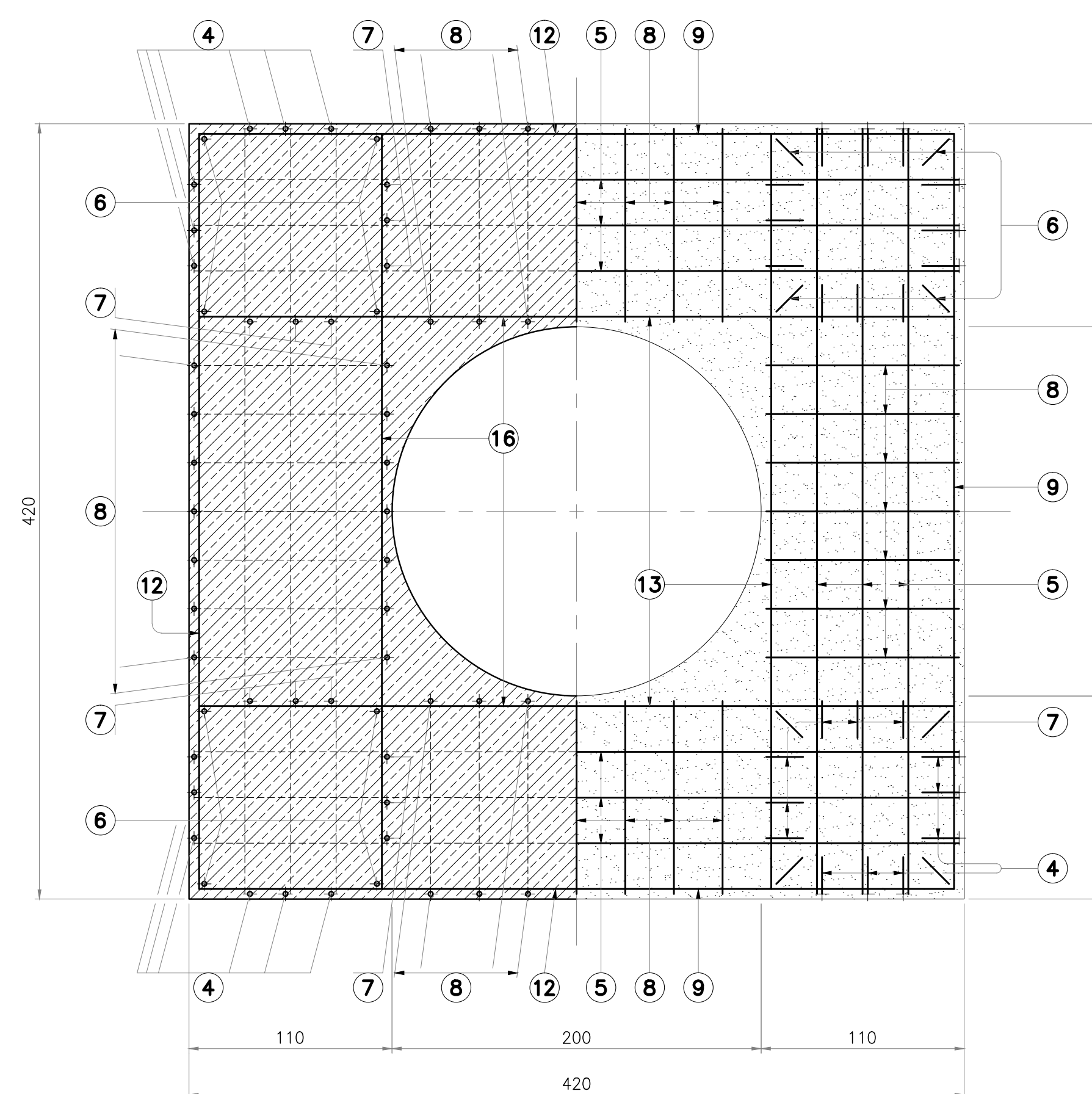
SEZIONE C-C (1:25)
