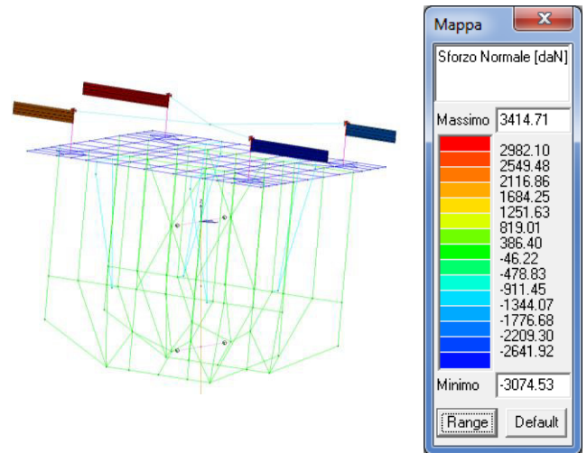
Combinazioni sismiche
