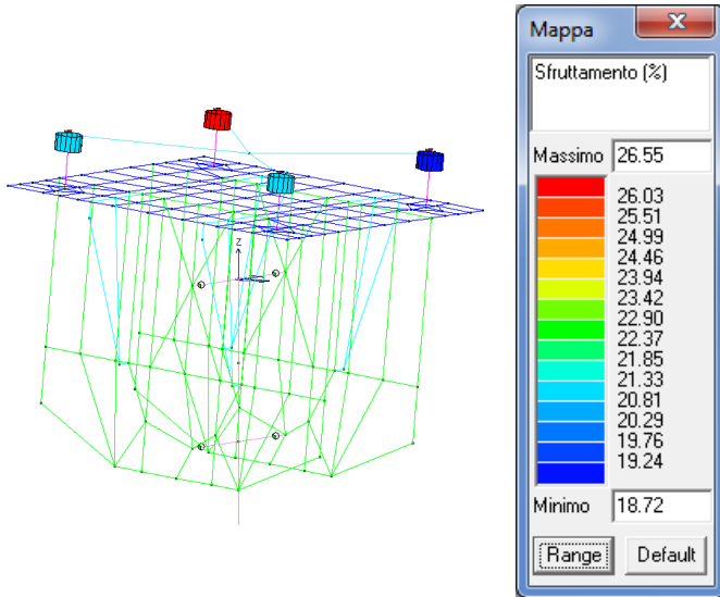
Combinazioni statiche
