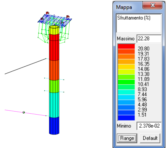
Combinazioni sismiche
