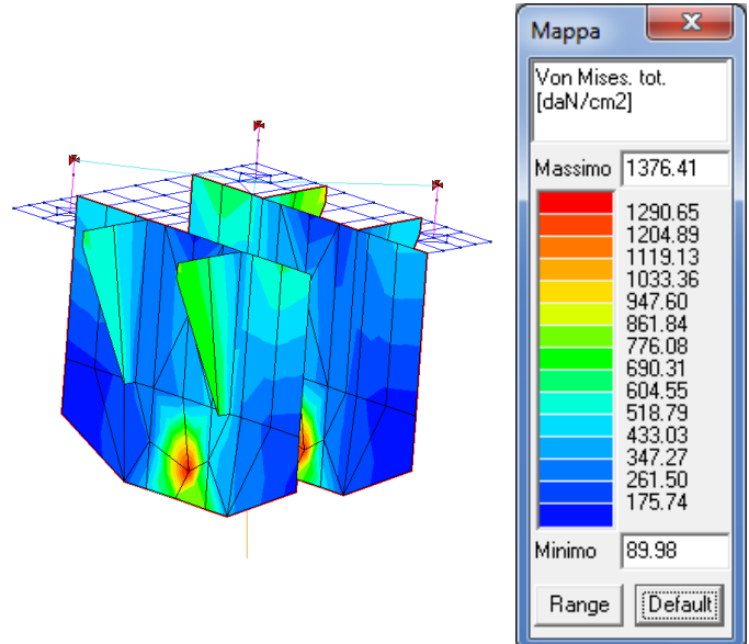
Combinazioni sismiche
