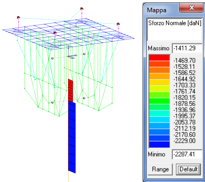
Combinazioni statiche
