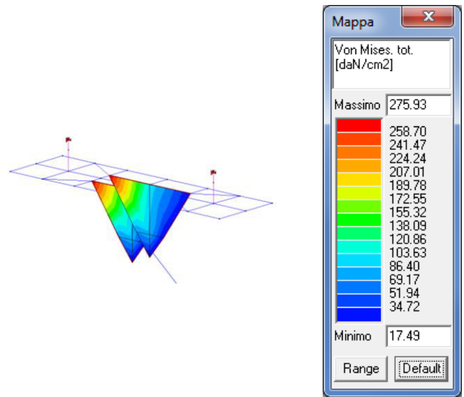
Combinazioni sismiche
