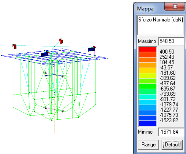
Combinazioni statiche
