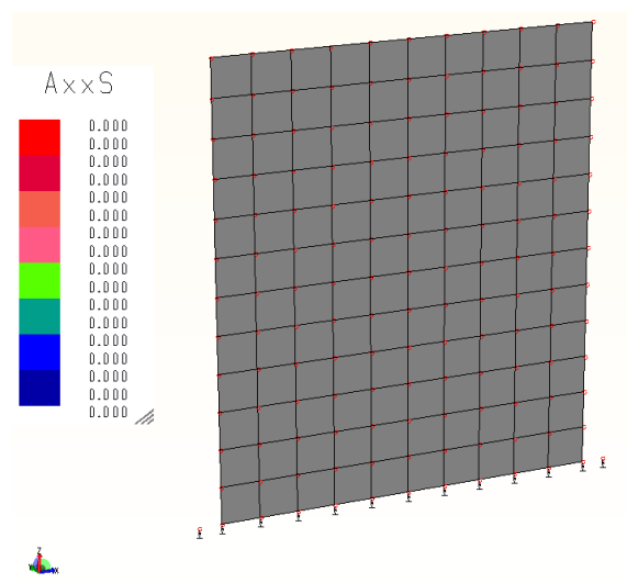
Figura 3 Armatura aggiuntiva superiore lungo x
