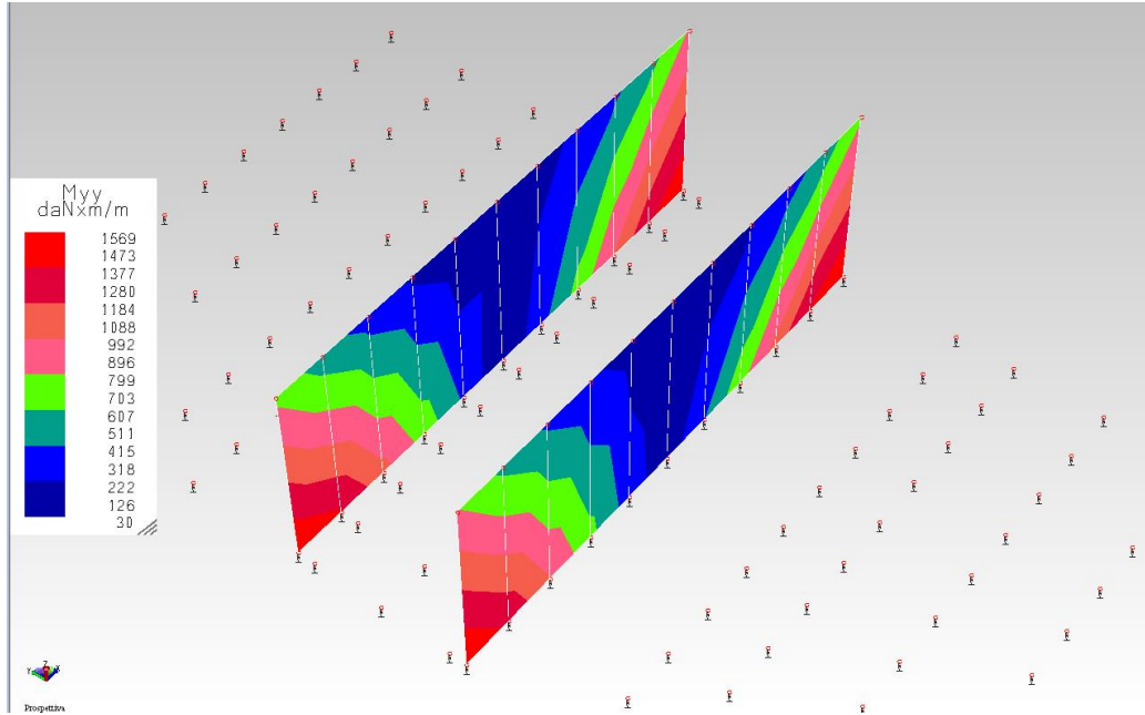
Fig. 16: Mappa di colore del momento flettente Myy (Myy,max= 1569 daN m/m).
