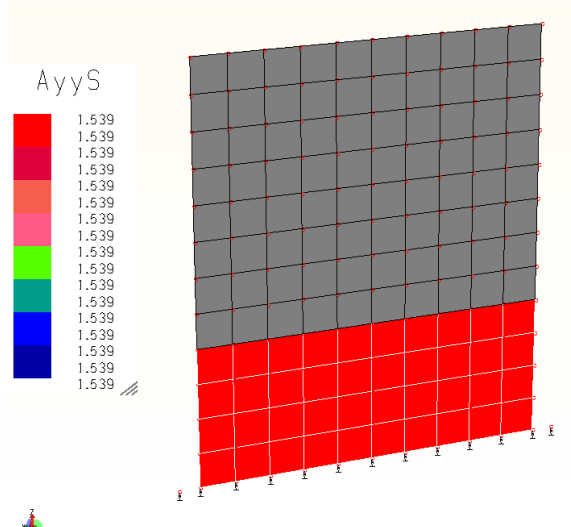
Figura 5 Armatura aggiuntiva superiore lungo y
