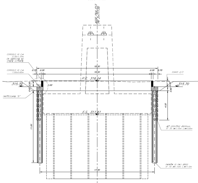
Figura 1 Sezione trasversale pila 13
