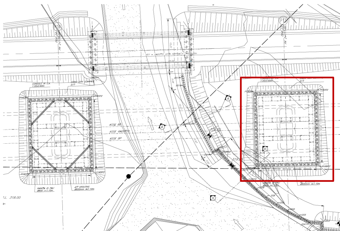
PILA P13: SEZIONE TRASVERSALE Scala 1:100
