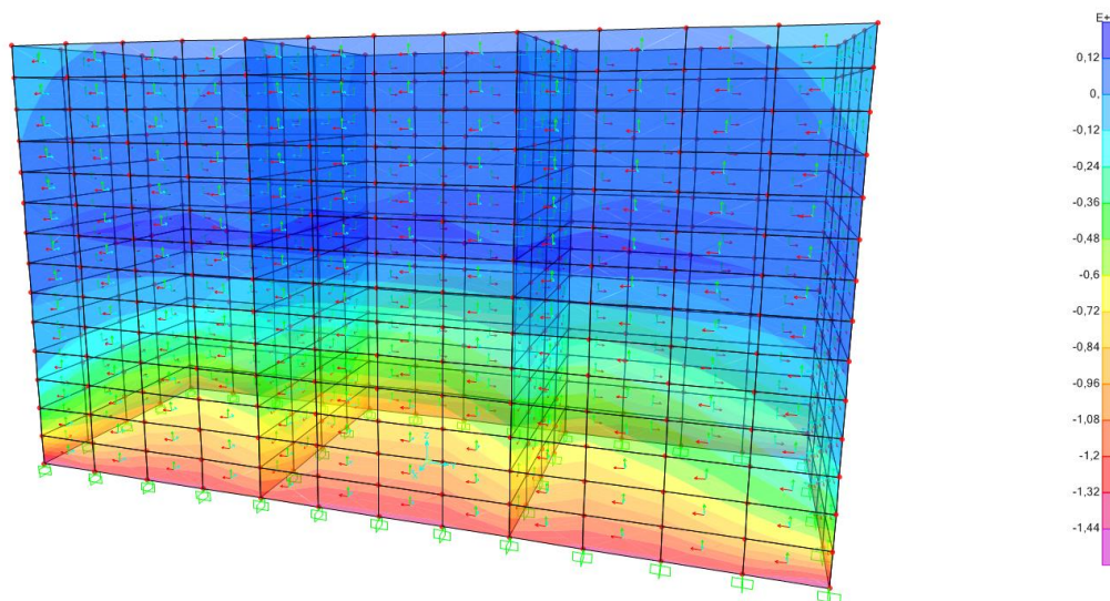
Figura.9.2 Azione assiale in direzione trasversale
