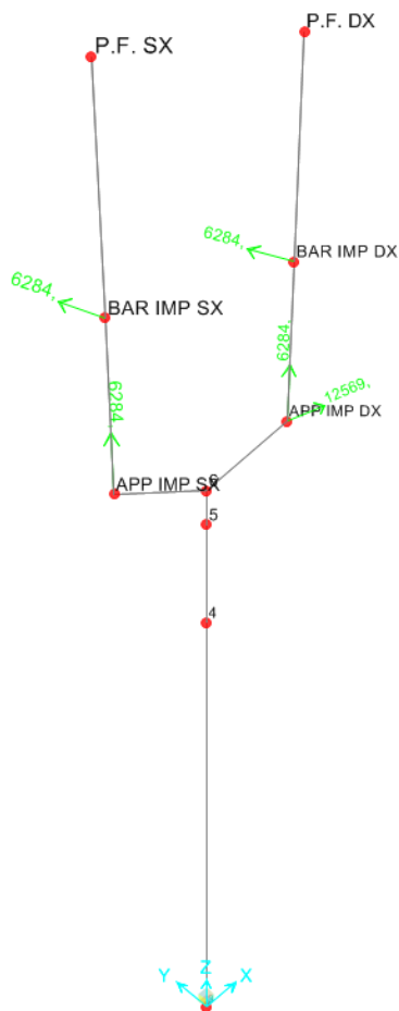
Figura 8.3 Assegnazione delle masse sismiche al modello di calcolo
