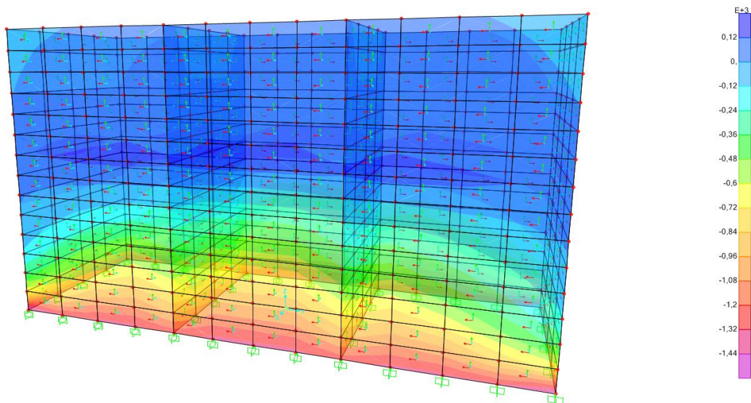
Figura.9.3 Azione assiale in direzione trasversale
