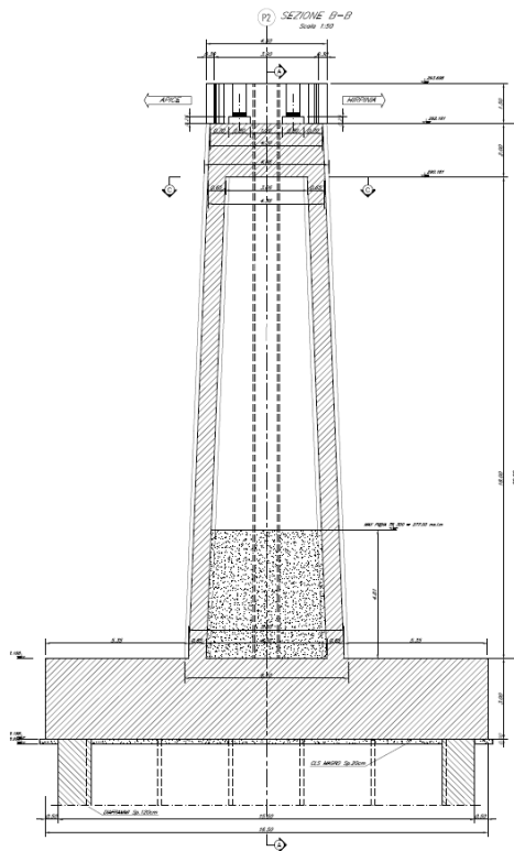
Figura 1 sezione trasversale pila2
