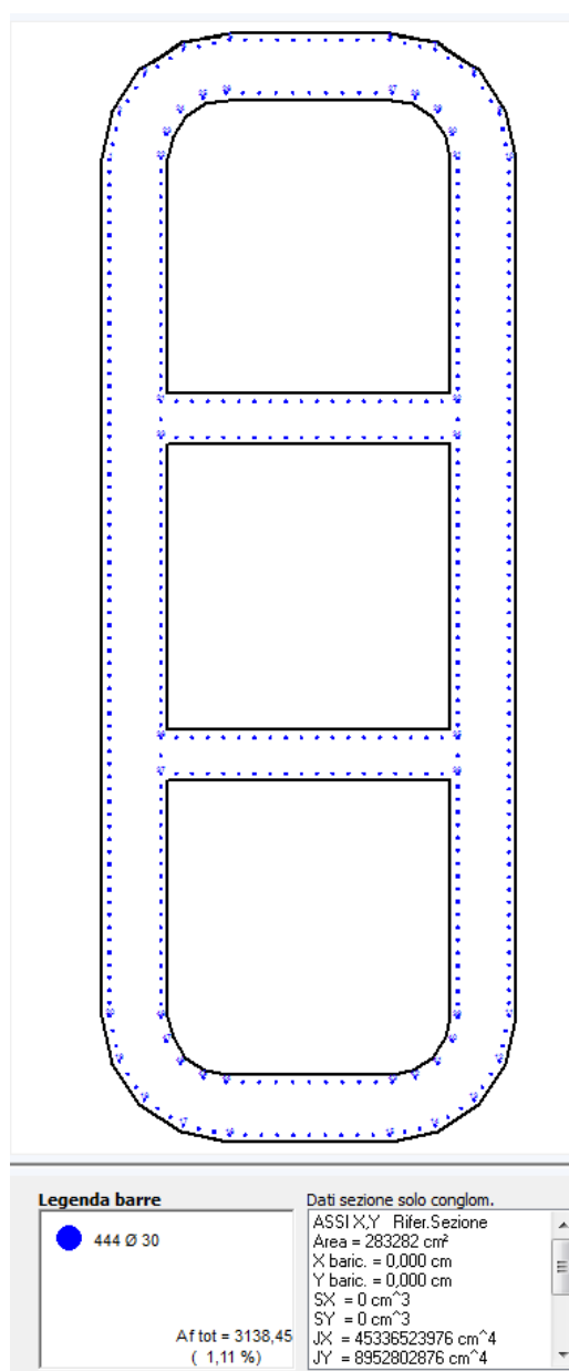
Figura 9.2 Disposizione dell'armatura verticale
