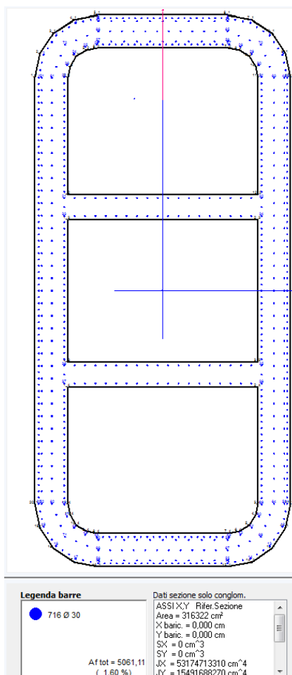
Figura 9.1 Disposizione dell'armatura verticale
