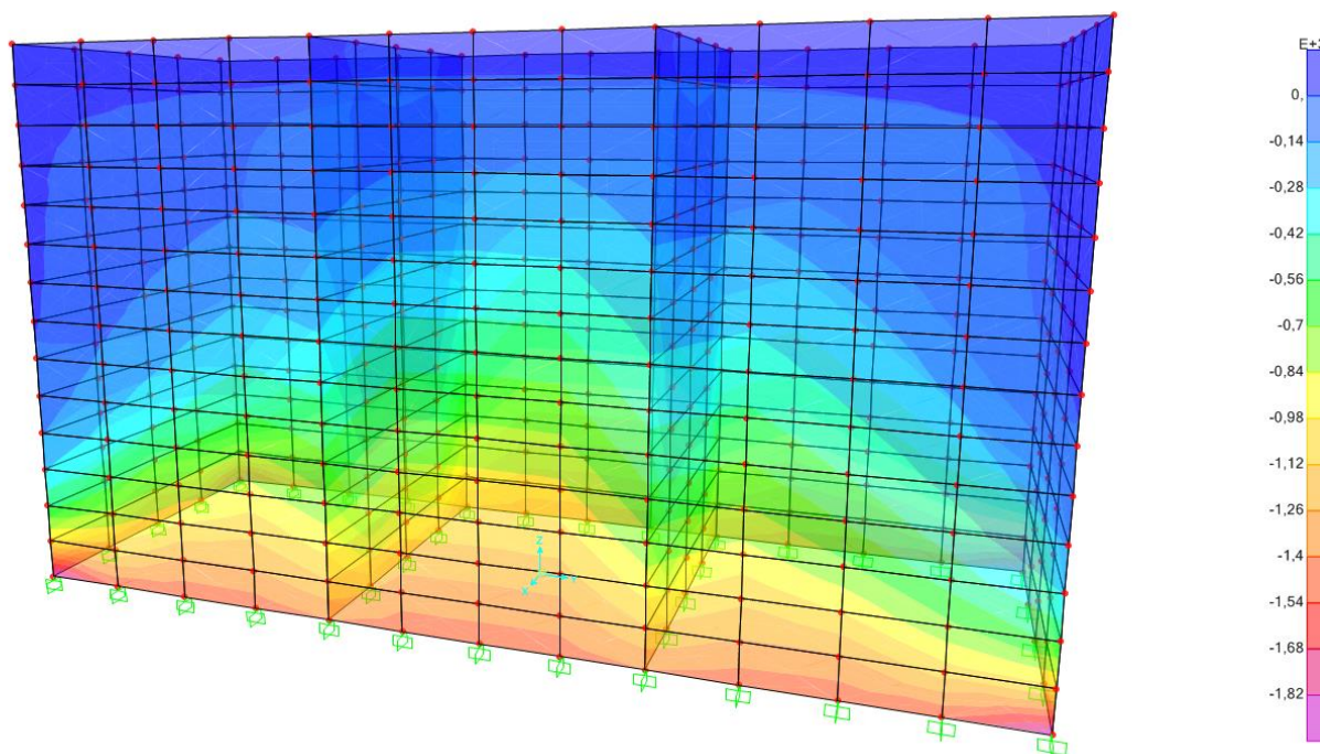
Figura 9.4 Azione assiale in direzione trasversale generata dal ritiro differenziale pila-fondazione
