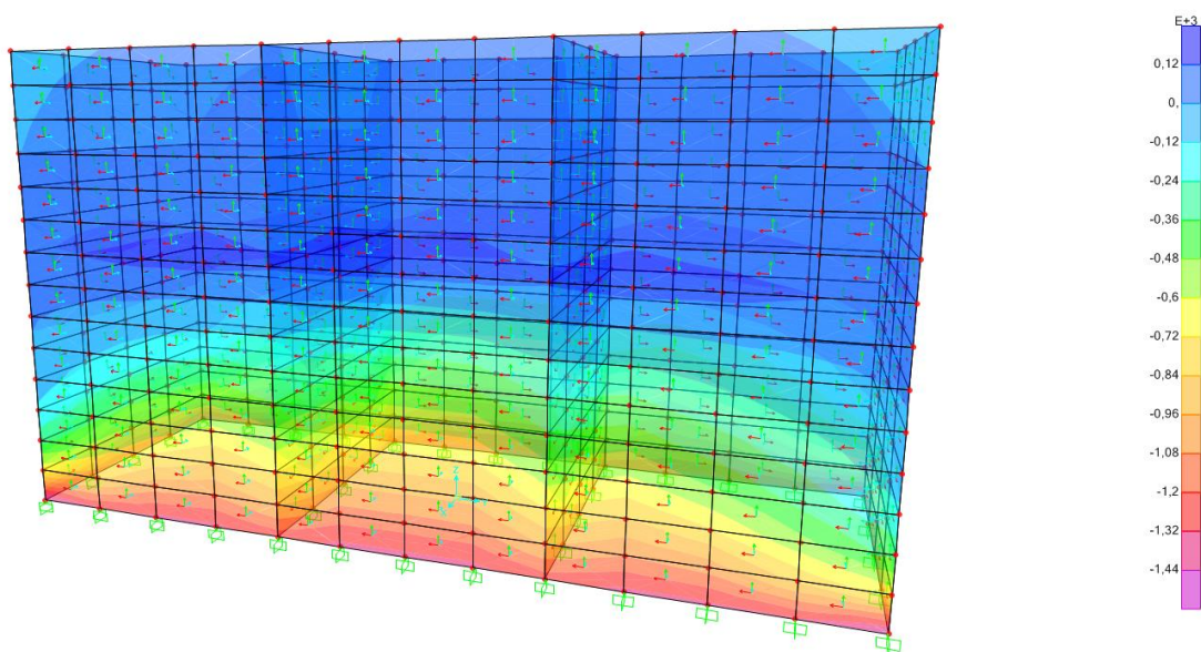
Figura.9.3 Azione assiale in direzione trasversale
