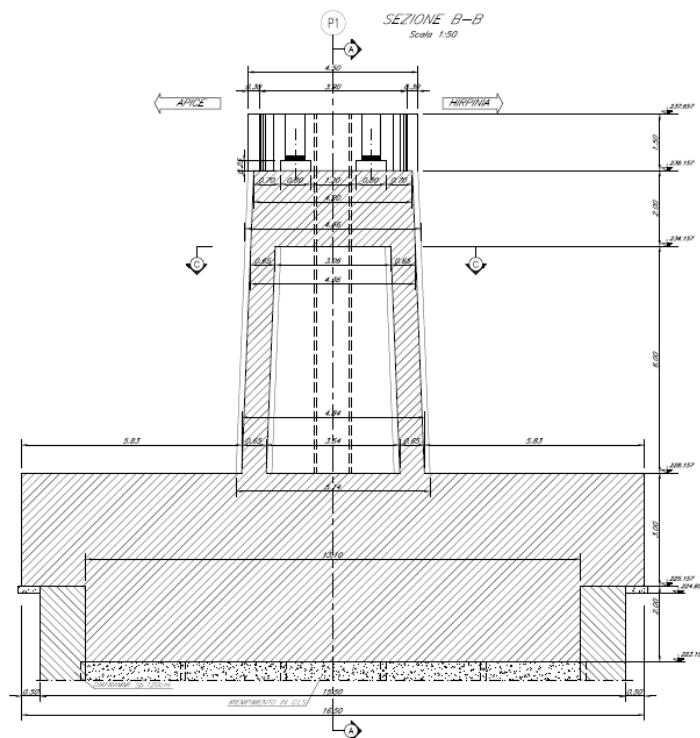
Figura 1 Sezione trasversale pila1
