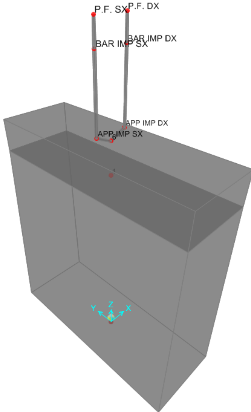
Figura 8.2 Vista estrusa del modello di calcolo delle pile
