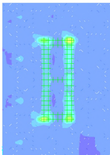
Figura 11.11 V13 min SLV
