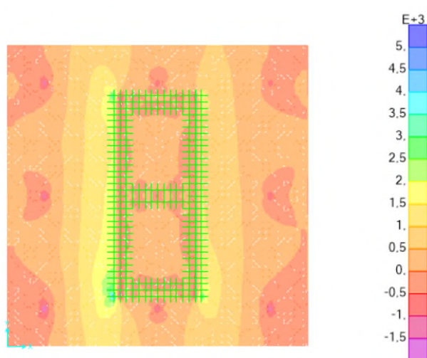
Figura 10.25 M11 min SLE
