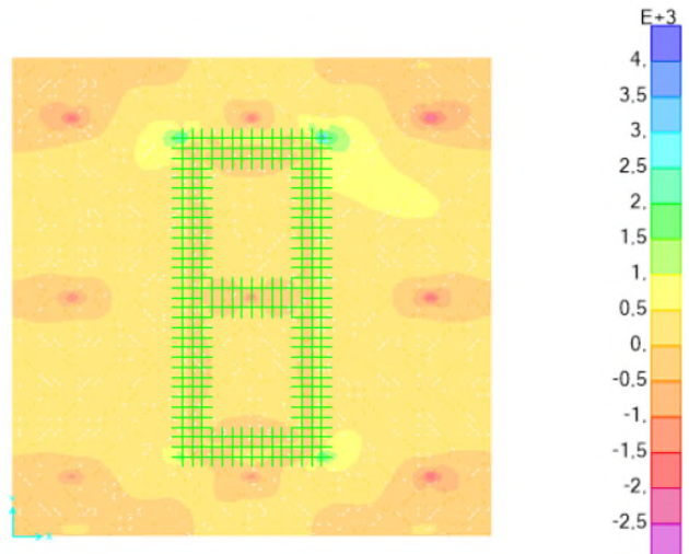
Figura 10.17 M22 min SLU
