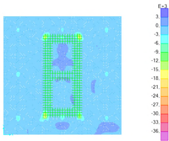
Figura 10.13 V23 min SLV
