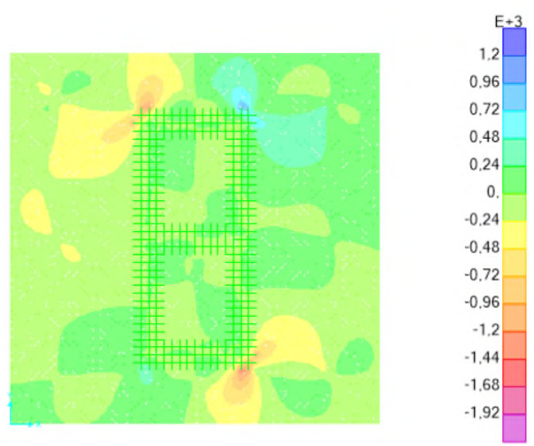
Figura 10.19 M12 min SLU
