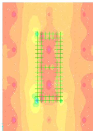
Figura 11.25 M11 min SLE
