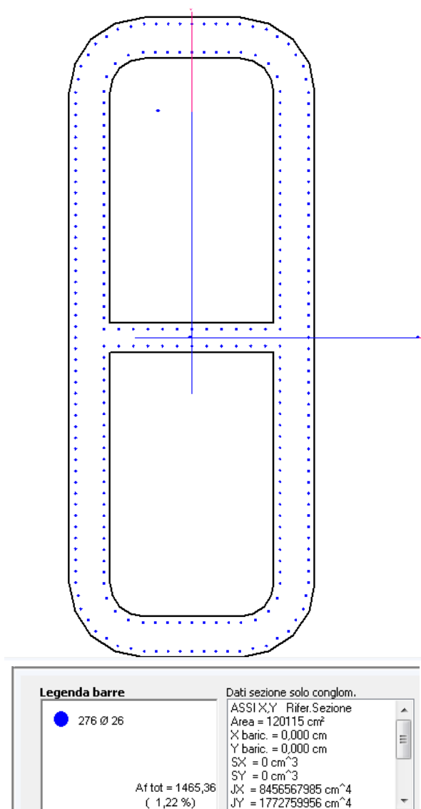
Figura 9.1 Disposizione dell'armatura verticale
