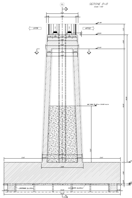
Figura 1 Sezione trasversale pila5
