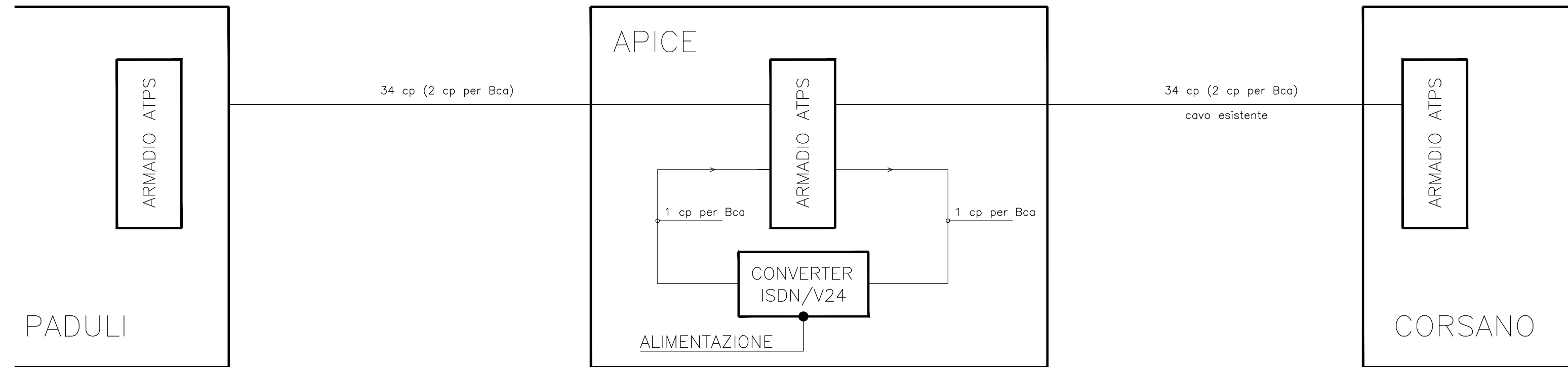
DETTAGLIO DEL CONVERTER ISDN/V24 THALES
