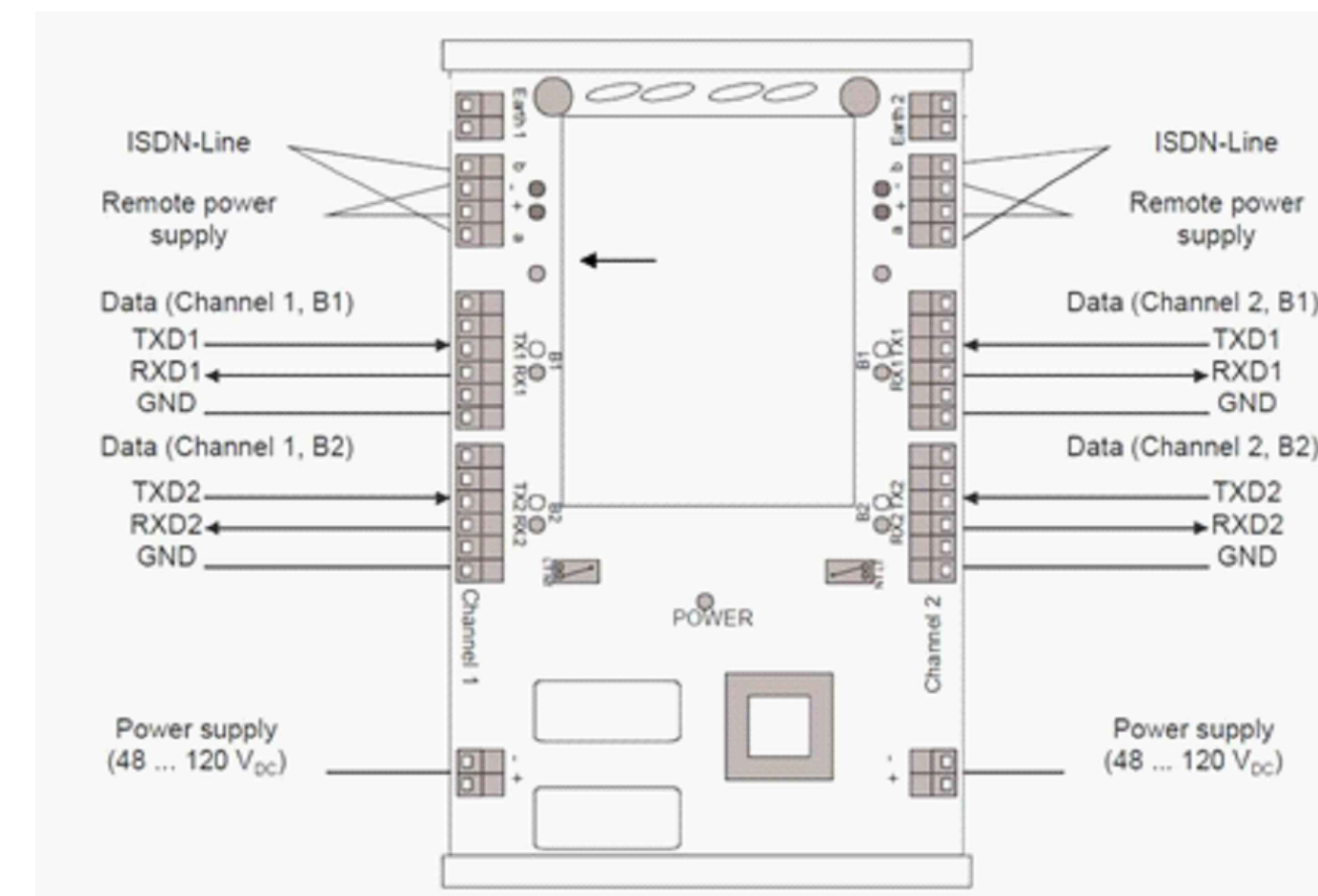
DETTAGLIO DEL CONVERTER ISDN/V24 THALES
