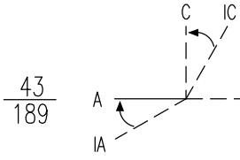
MANIPOLATORE SEZIONATORE BIPOLARE APERTURA-CHIUSURA
