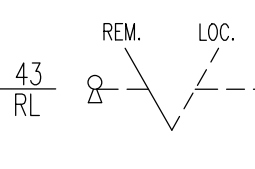
COMMUTATORE REGIME DI FUNZIONAMENTO REMOTO-LOCALE
