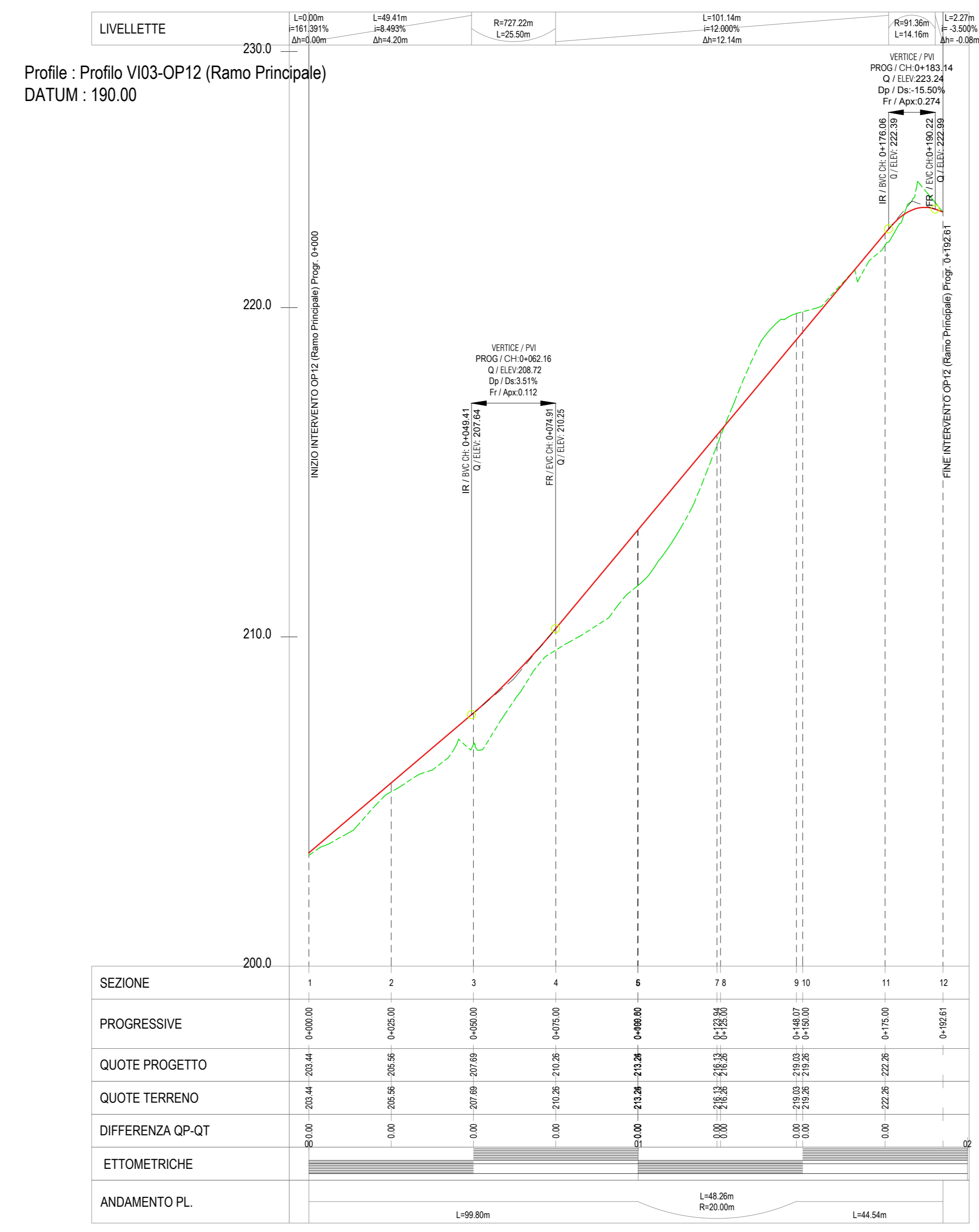
VI03 - VIADOTTO UFITA ROCCHETTA DA KM 9+632 A KM 10+047 PROFILO LONGITUDINALE Scala 1:1000/100
