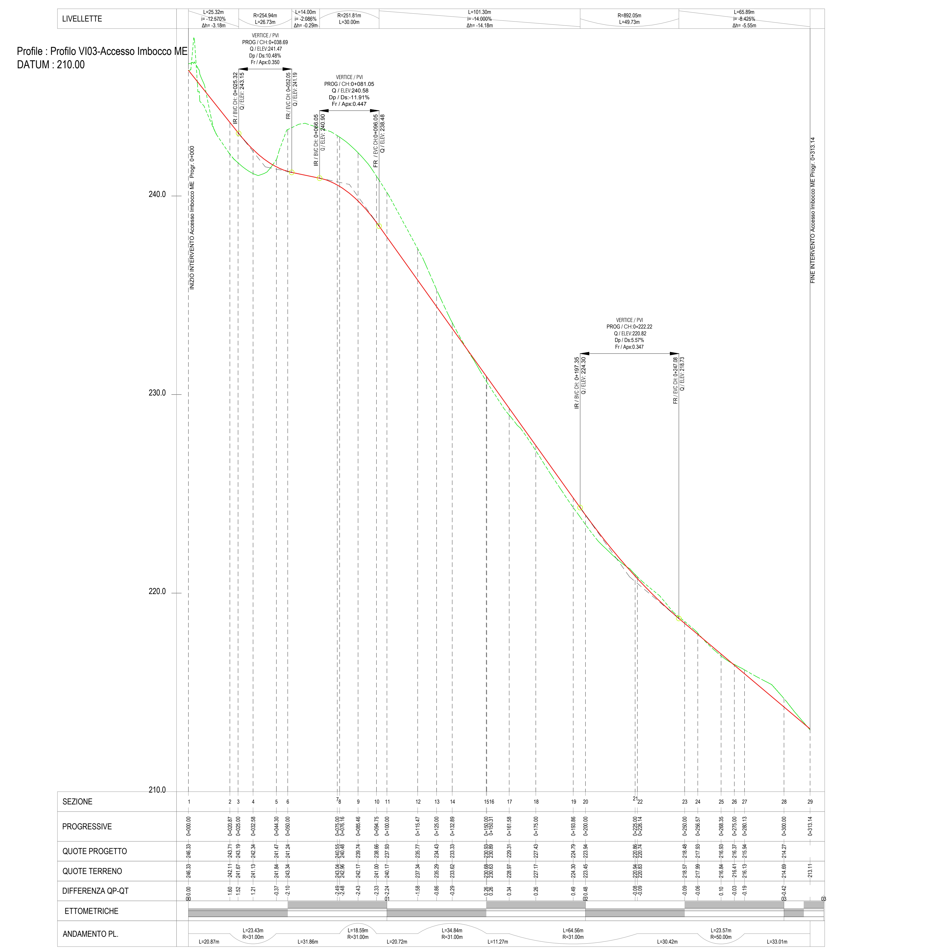
VI03 - VIADOTTO UFITA ROCCHETTA DA KM 9+632 A KM 10+047 PROFILI LONGITUDINALE Scala 1:1000/100
