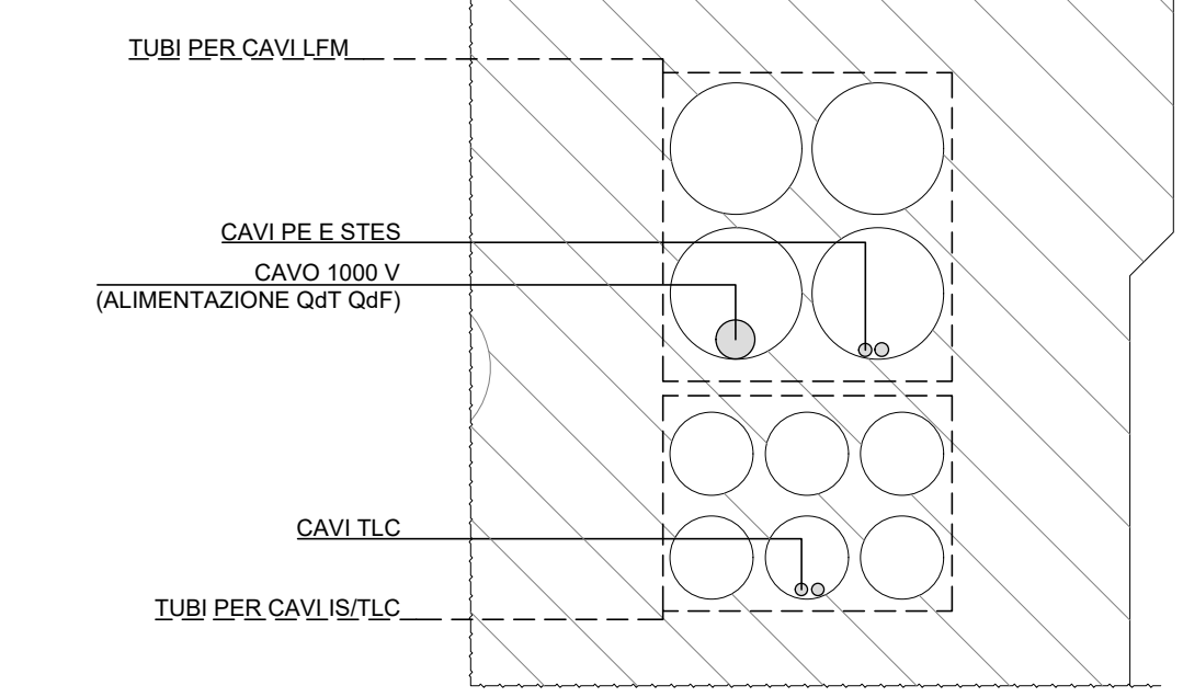
DETTAGLIO RIEMPIMENTO TUBAZIONI SOTTO MARCIAPIEDE - BINARIO PARI
