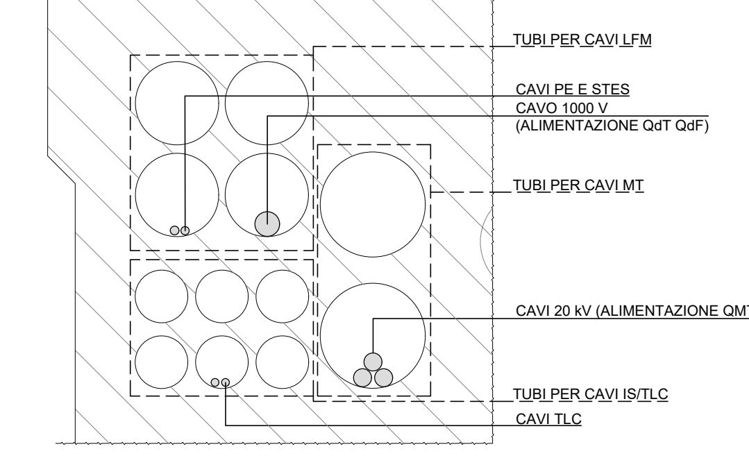
DETTAGLIO RIEMPIMENTO TUBAZIONI SOTTO MARCIAPIEDE - BINARIO PARI
