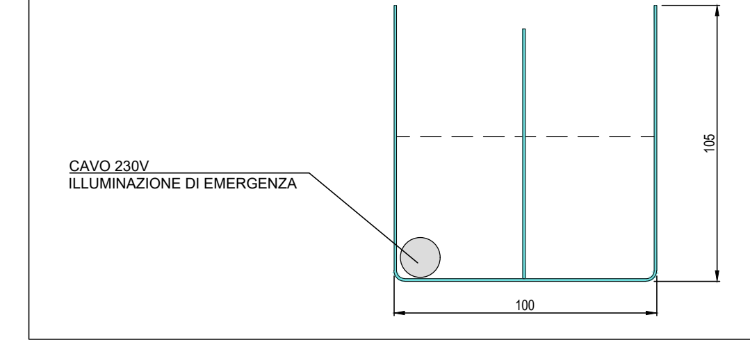
DETTAGLIO RIEMPIMENTO PASSERELLA 100 x 105 mm - BINARIO PARI E DISPARI
