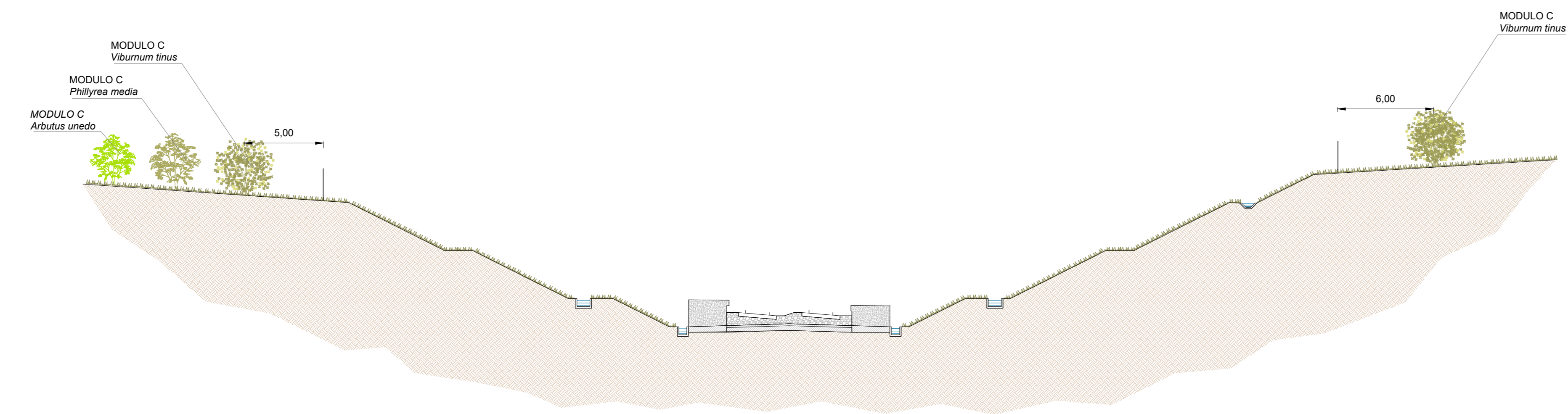
Sezione A-A'
