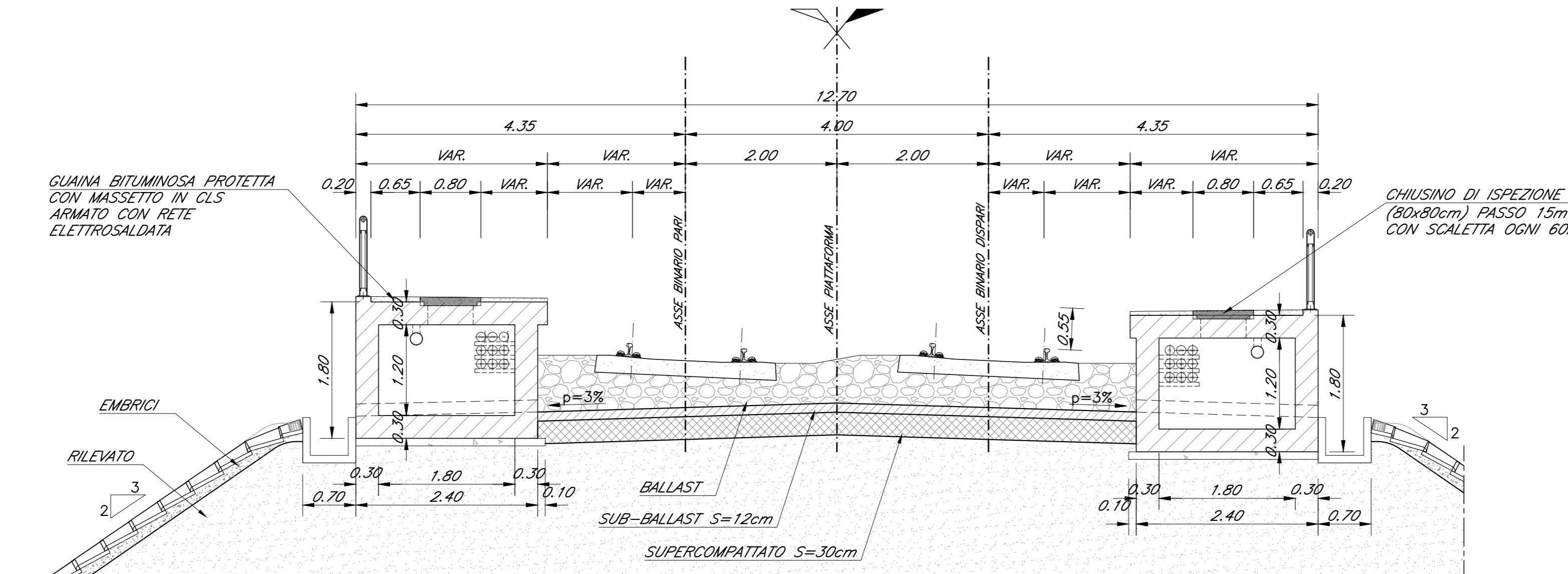
SEZIONE TRASVERSALE TIPOLOGICA SU RILEVATO TR02 Scala 1:50
