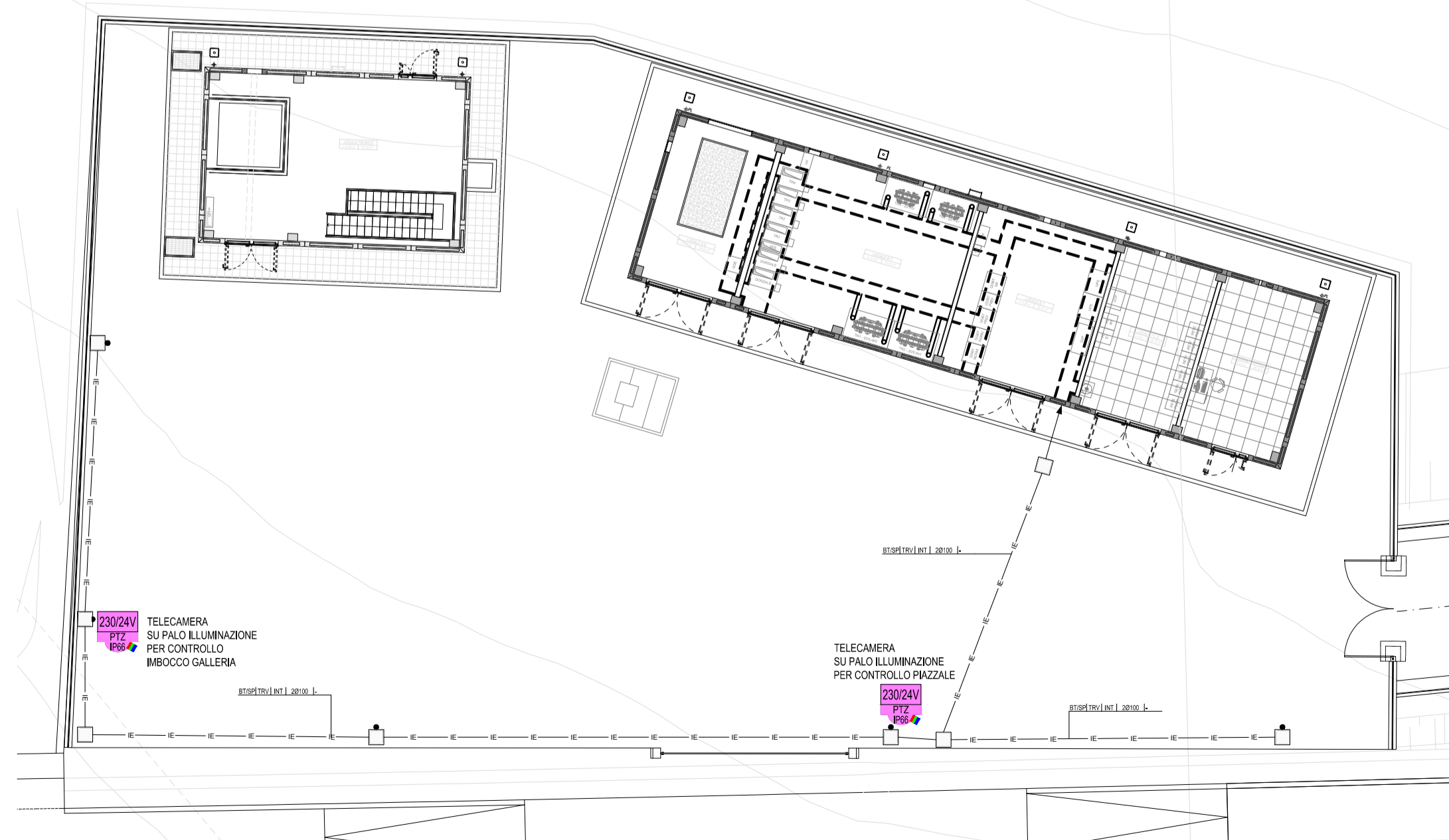
PLANIMETRIA PIAZZALE FABBRICATO FA02 TELECAMERE SU PALI ILLUMINAZIONE (Scala 1:200)
