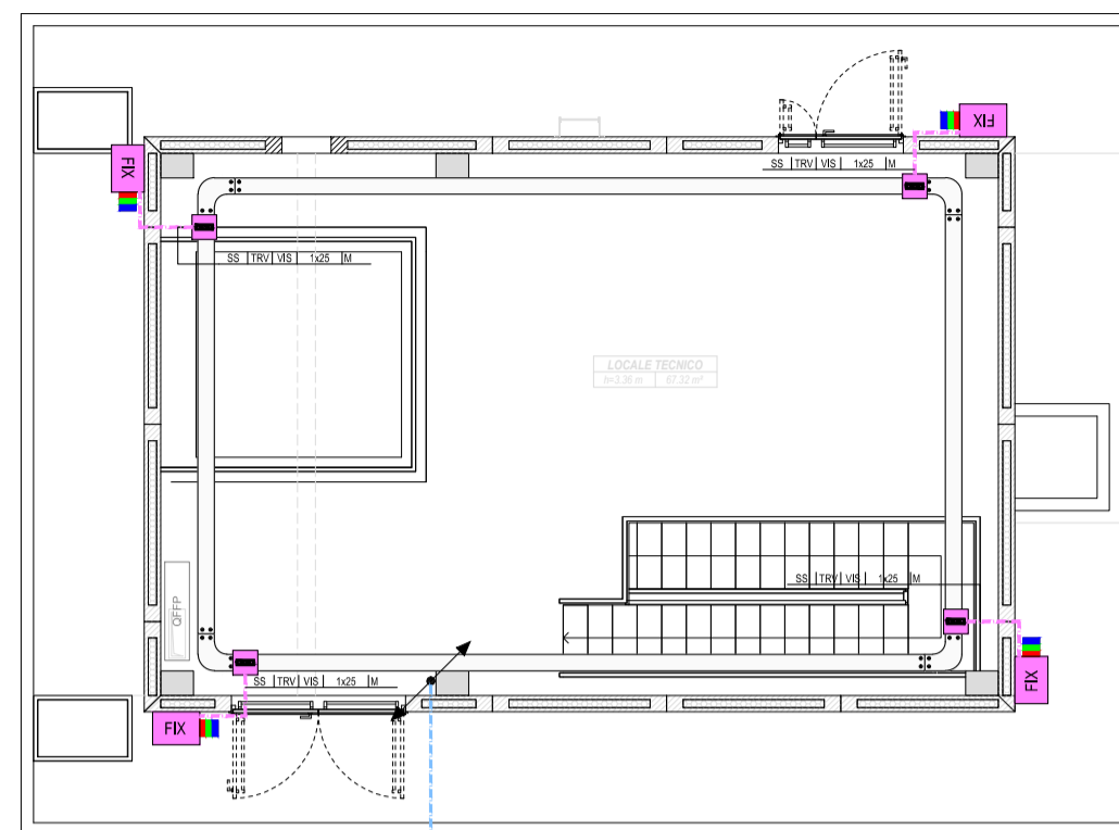
PIANTA FABBRICATO FA02B PIANTA PIANO TERRA
