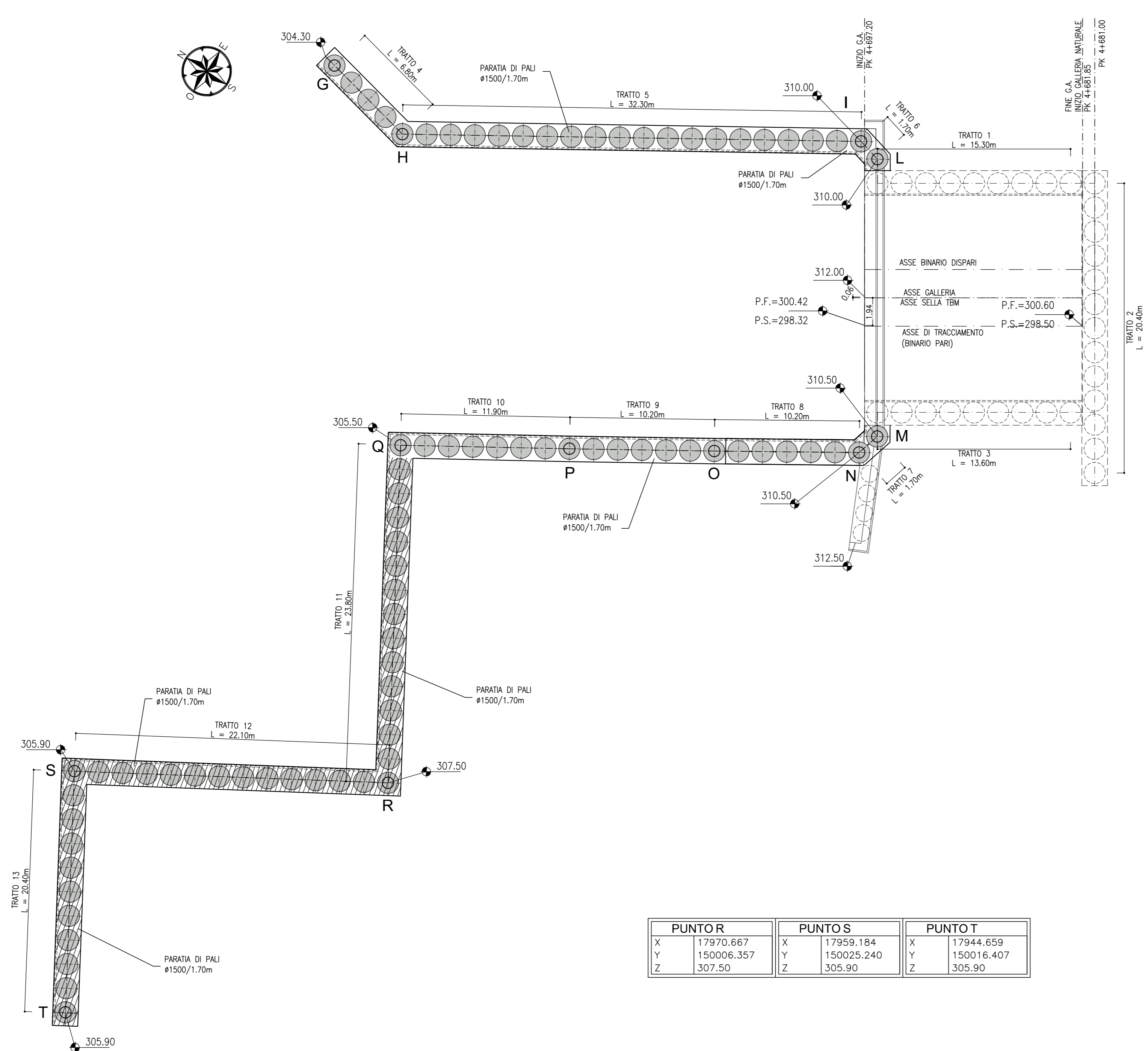
PLANIMETRIA DI INTERVENTO SCALA 1:200
