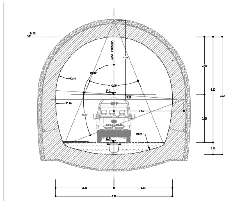
Figura 1 - Sezione tipo di intradosso uscita di emergenza carrabile
